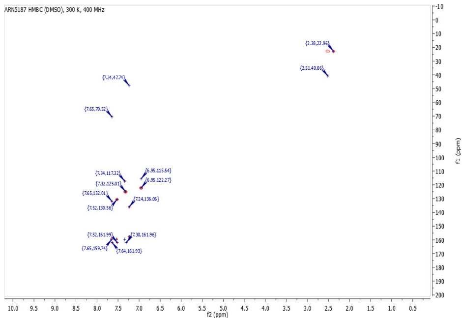
ARN5187 HMBC (DMSO), 300 K, 400 MHz
