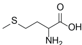
L-Methionine (Met)
