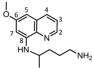
Primaquine
