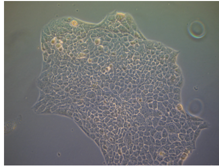
Salinomycin (8uM)
