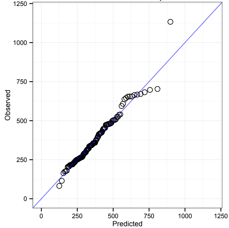
b-Quantile-Quantile plot
