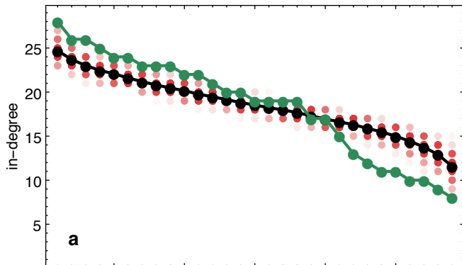
macaque
