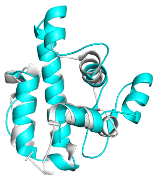
LHD
