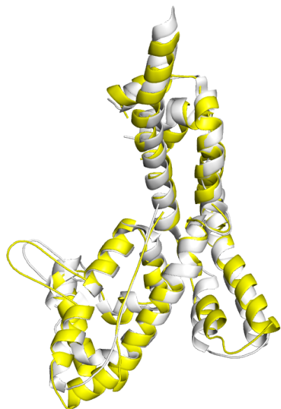
Helical-I
