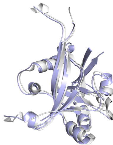
OBD
