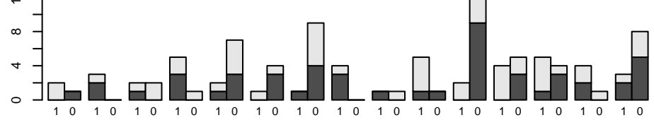
Leuconostoc mesenteroides
