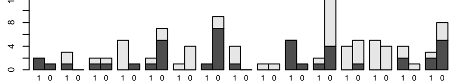
Moraxella boevrei
