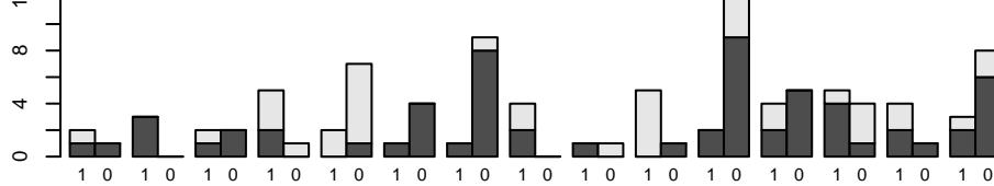
Leuconostoc pseudomesenteroides
