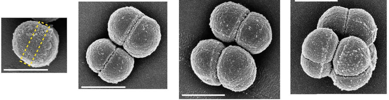
Salinicoccus roseus
