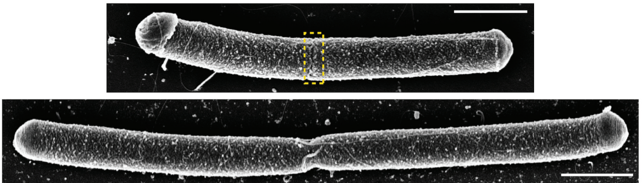
Bacillus subtilis
