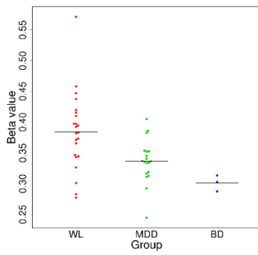
cg07398767 (CA10)
