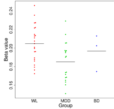
cg19006127 (N/A)
