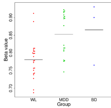
cg03773183 (N/A)
