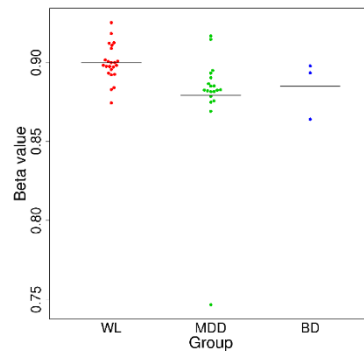
cg08292919 (GABBR1)
