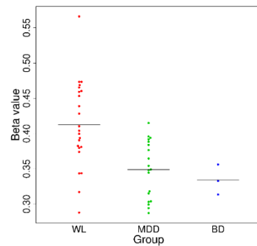
cg01724150 (NMNAT3)
