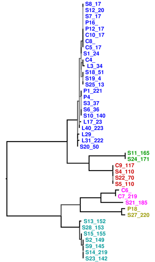
F - mreA
