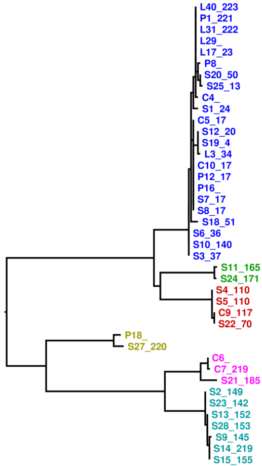
E - pfkB
