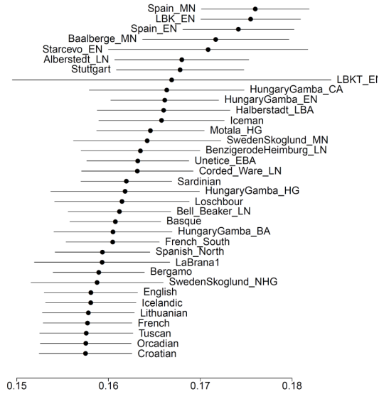
(a) Esperstedt_MN
