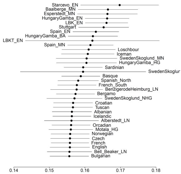
(b) HungaryGamba_CA
