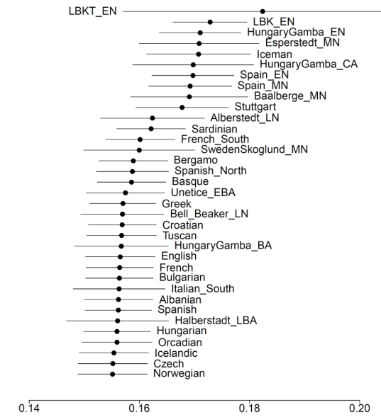
(c) Starcevo_EN
