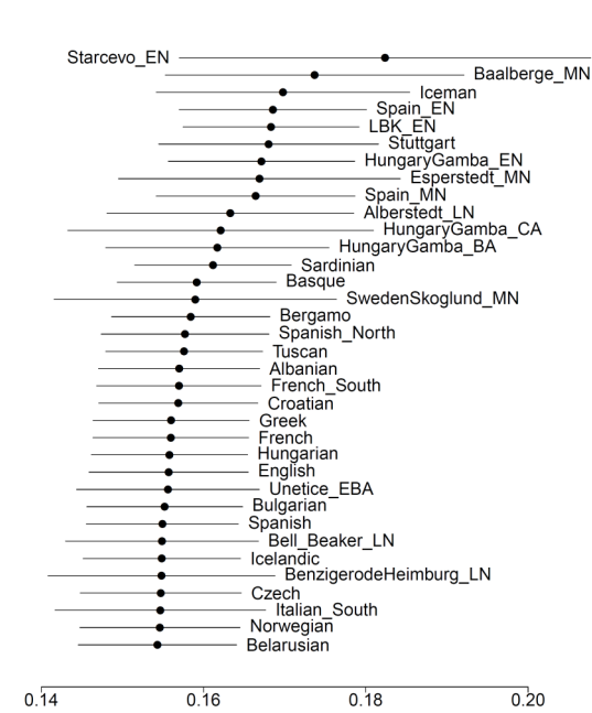
(b) LBKT_EN
