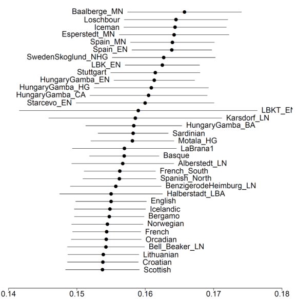
(d) SwedenSkoglund_MN
