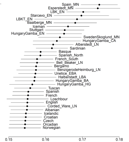
(d) Spain_EN
