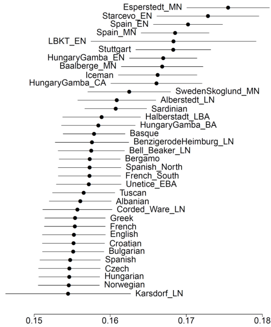
(a) LBK_EN
