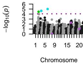
TKW, Mean
