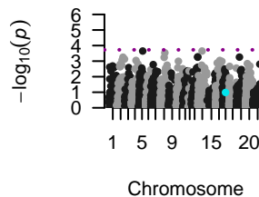
DH, RF
