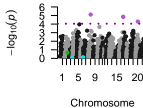
TKW, RF
