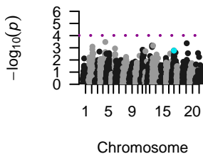
DH, MVN-EM
