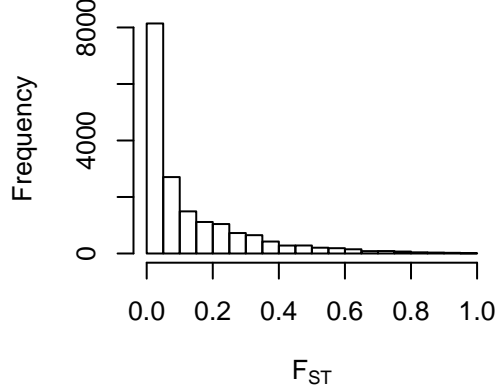
D. N=400 SN=1000 F_{ST}
