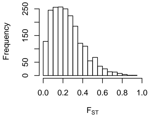
C. N=400 SN=10000 F_{ST}
