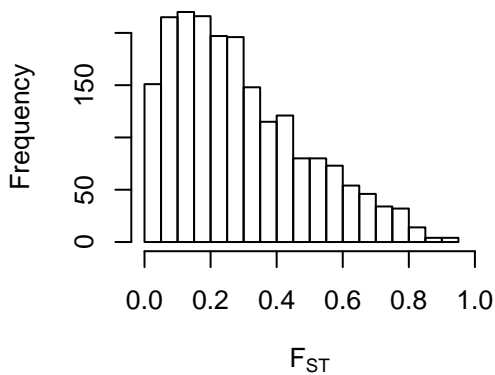
A. N=200 SN=10000 F_{ST}
