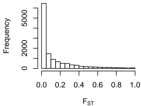
B. N=200 SN=1000 F_{ST}
