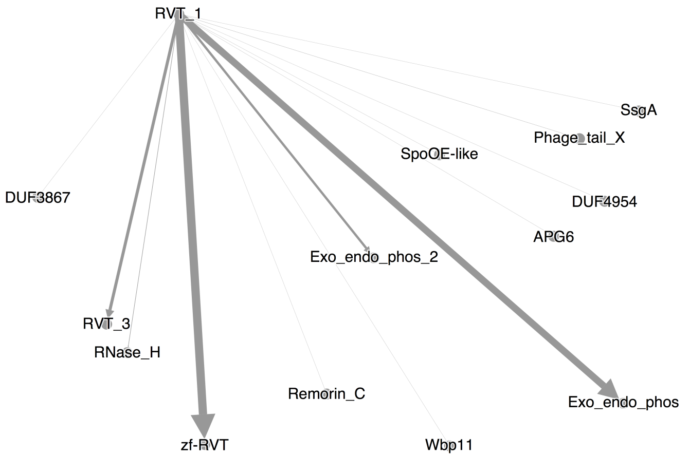
Figure 6g: Viridiplantae ORF2p domains
