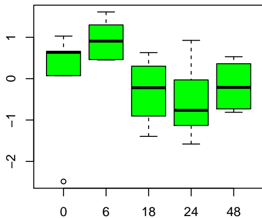
pipecolate
