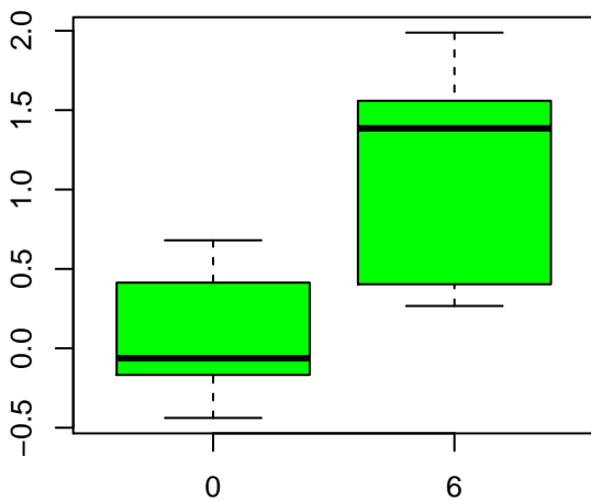
tyrosine
