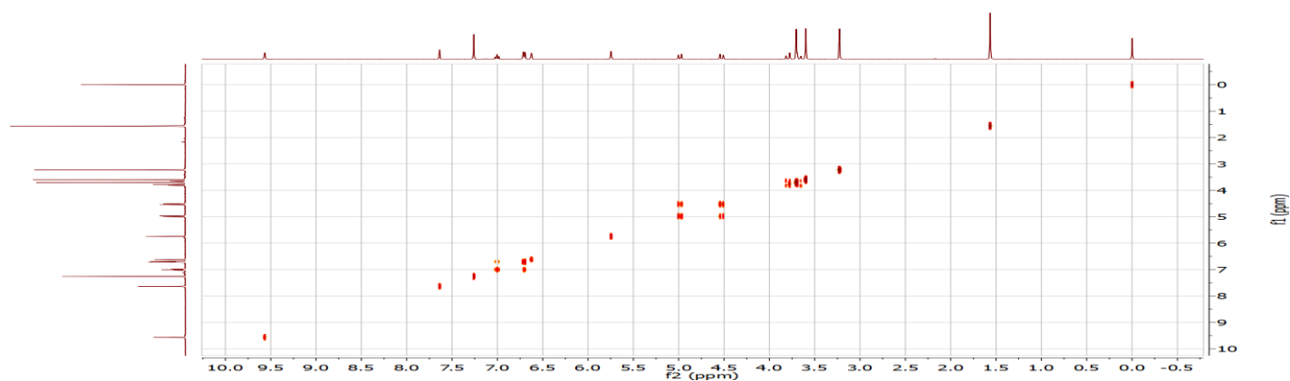
2D-COSY spectra of 6g
