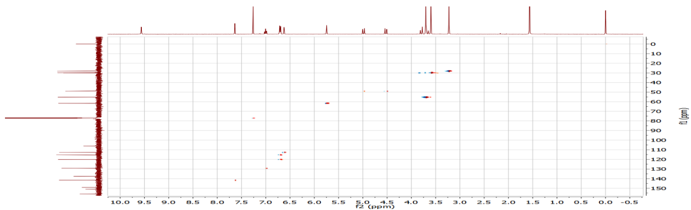
HSQC spectra of 6g
