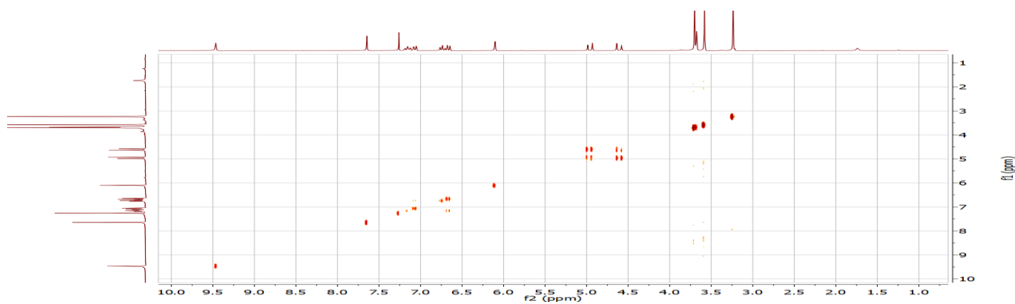
2D-COSY spectra of 6e
