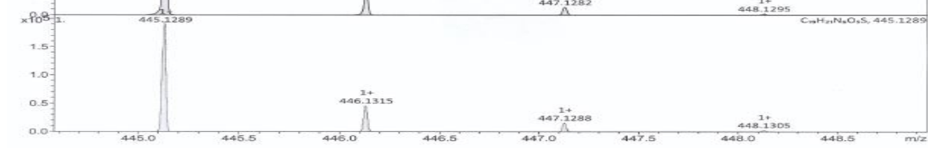
HRMS spectra of 6g
