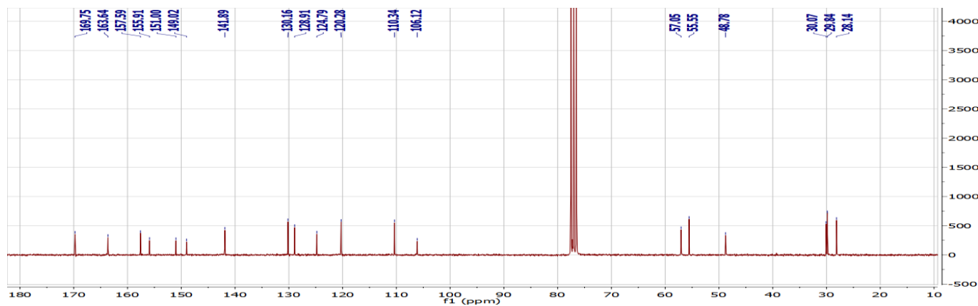
13 C-RMN spectra of 6e
