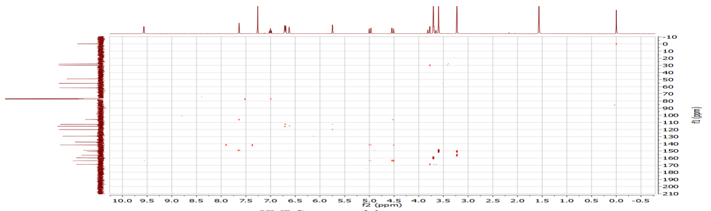
HMBC spectra of 6g
