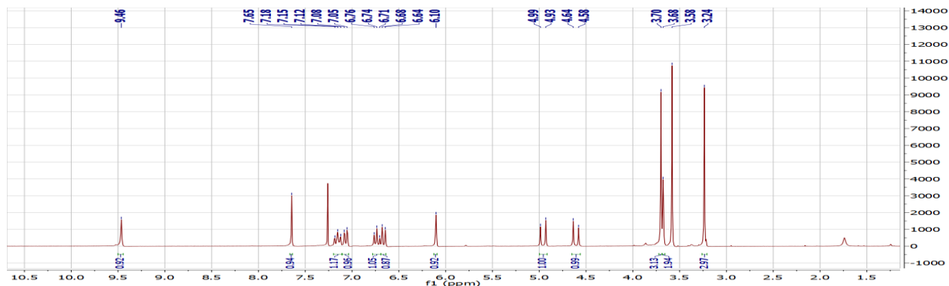
1 H-RMN spectra of 6e
