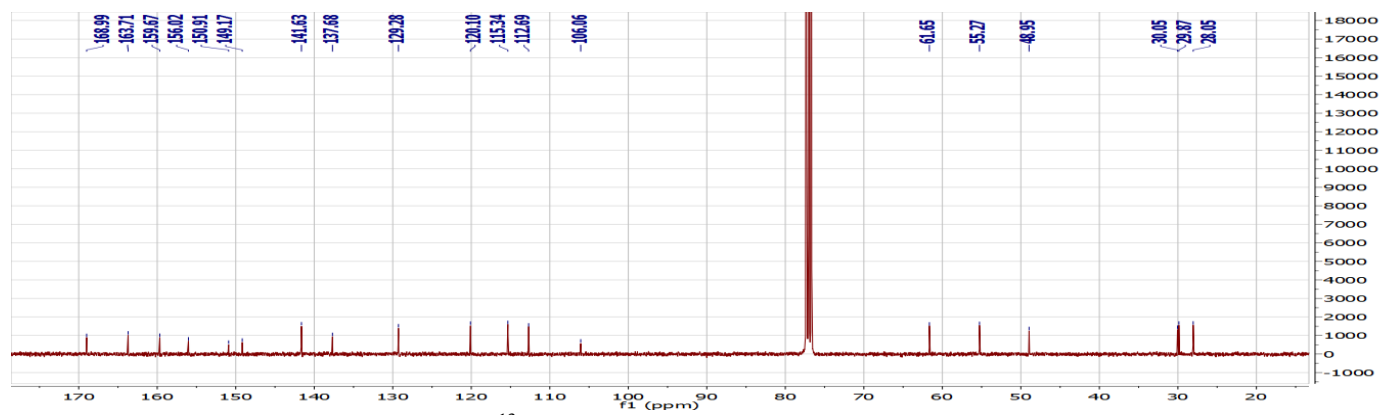
13 C-RMN spectra of 6g
