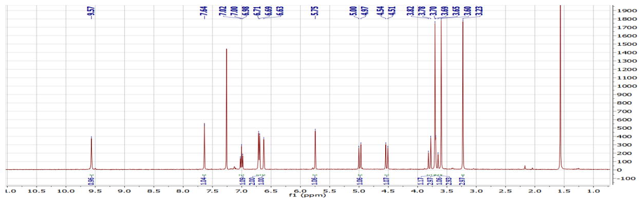
1 H-RMN spectra of 6g
