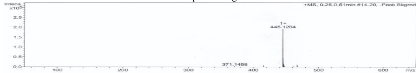
HMBC spectra of 6g
