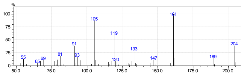
\alpha -Humulene
