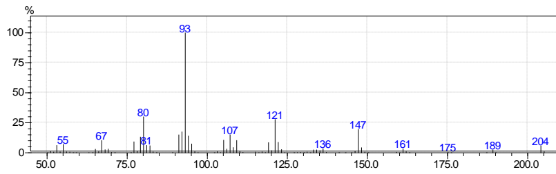
allo-Aromadendrene
