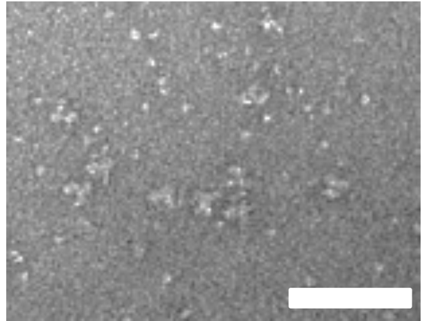
Arp2/3 + Arpin
