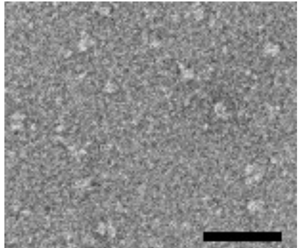
Arp2/3 + Gmf1
