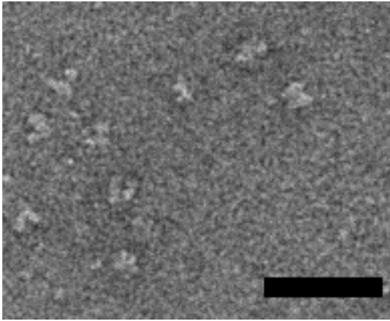
Arp2/3
