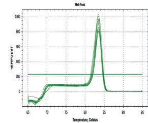
EpMADS9 SEP
