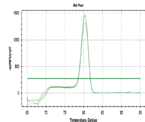
EpMADS7 SEP
