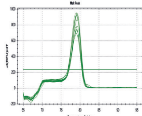
EpMADS10 FUL
