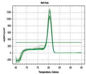
EpMADS3 AGL6
