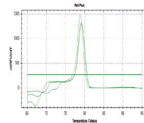
EpMADS8 SEP
