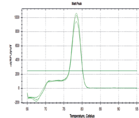
EpMADS22 AG
