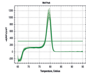
EpMADS4 AGL6
