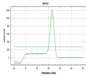
EpMADS10 FUL
