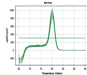
EpMADS5 AGL6
