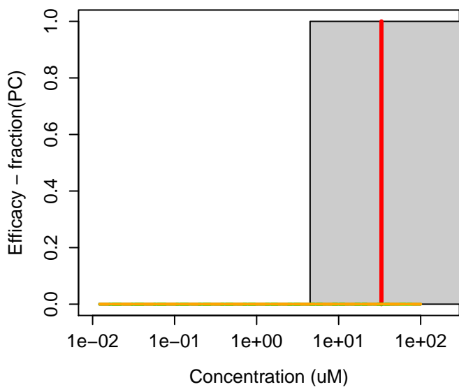
128-39-2 : 2,6-Di-tert-butylphenol
