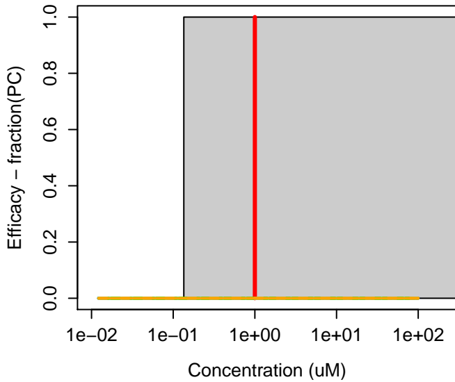
107071-66-9 : Ro 23-7637
