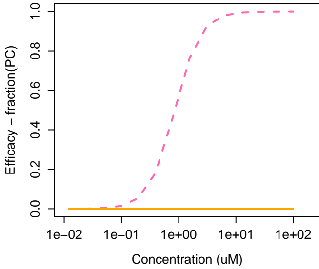
66441-23-4 : Fenoxaprop-ethyl
