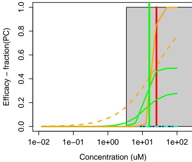
58-08-2 : Caffeine
