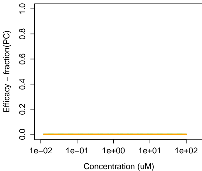
106-25-2 : (2Z)-3,7-Dimethylocta-2,6-dien-1-ol
