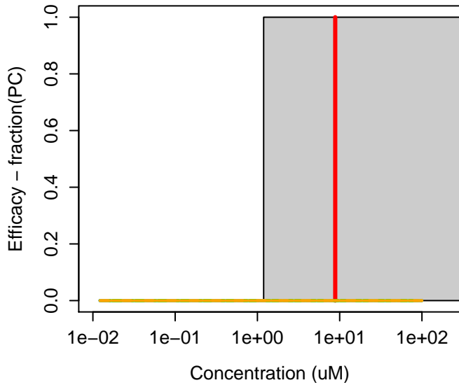
2425-06-1 : Captafol
