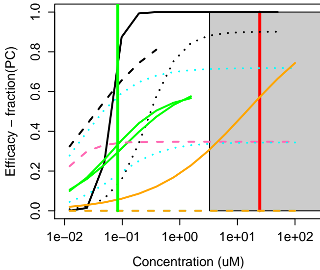
520-18-3 : Kaempferol
