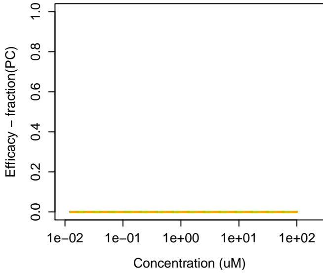
96-48-0 : 4-Butyrolactone
