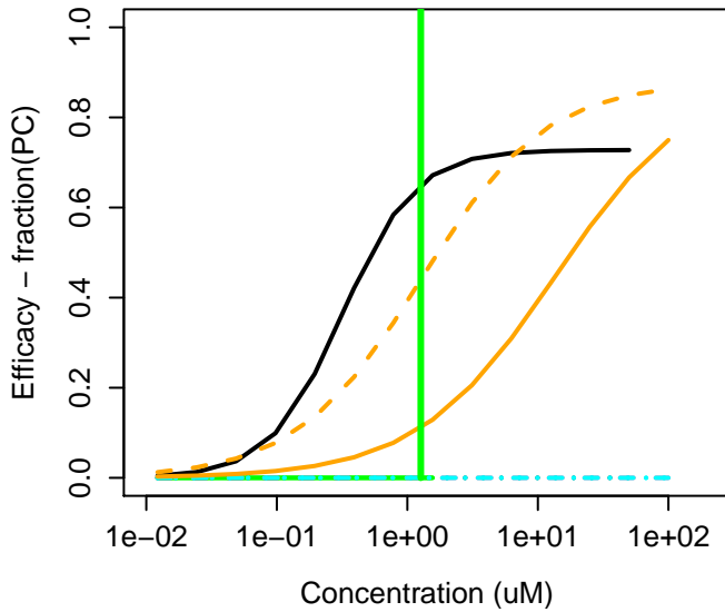
328-84-7 : 1,2-Dichloro-4-(trifluoromethyl)benzene
