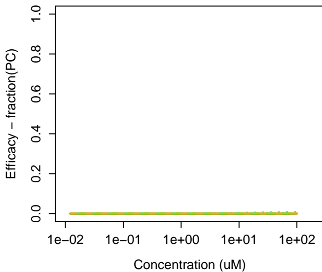
53894-23-8 : Triisononyl trimellitate
