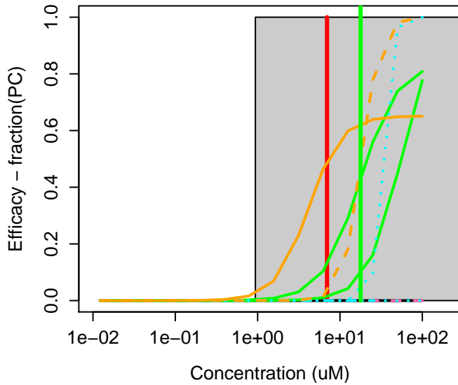
67564-91-4 : (2R,6S)-Fenpropimorph
