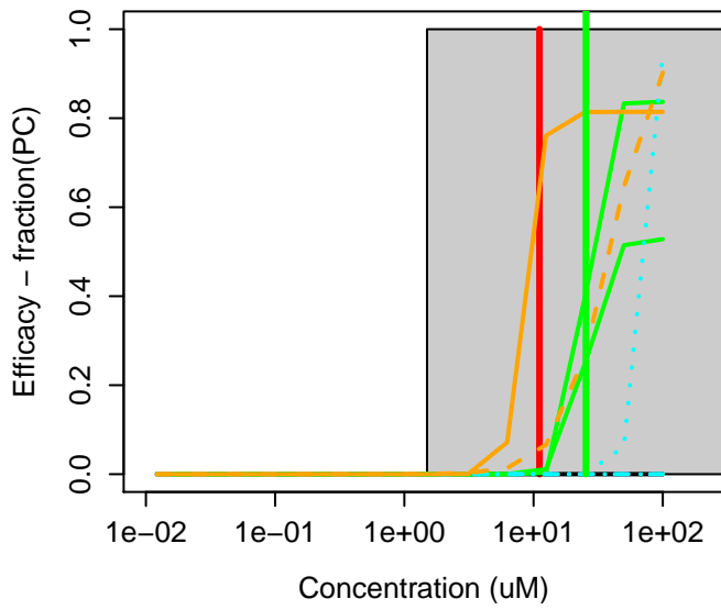
94-18-8 : Benzylparaben
