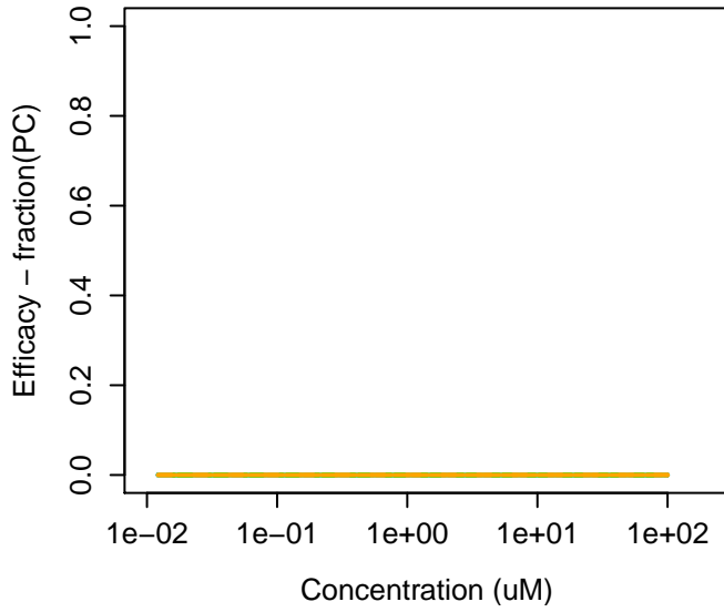
143-08-8 : 1-Nonanol
