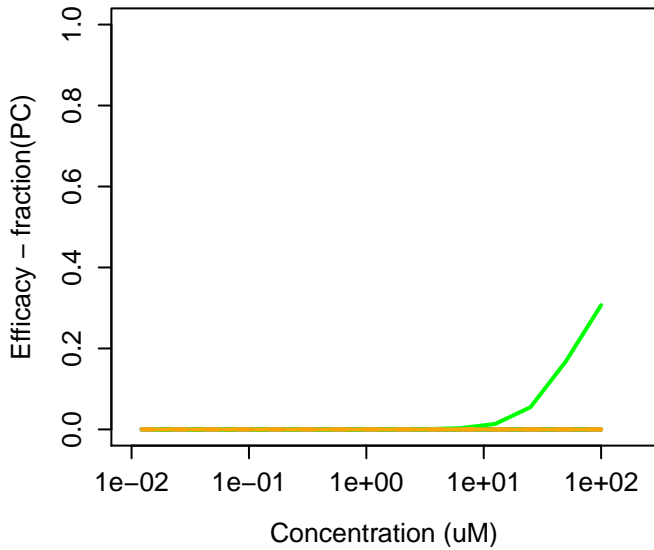
83-88-5 : Riboflavin
