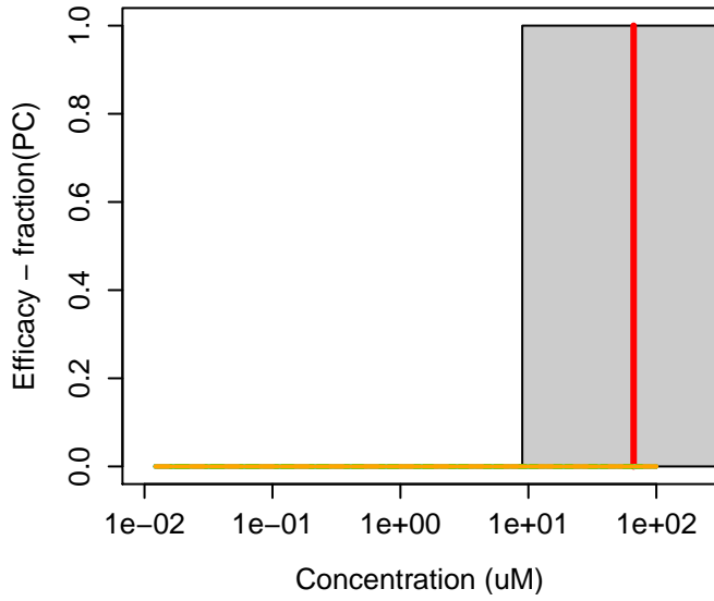
314-40-9 : Bromacil
