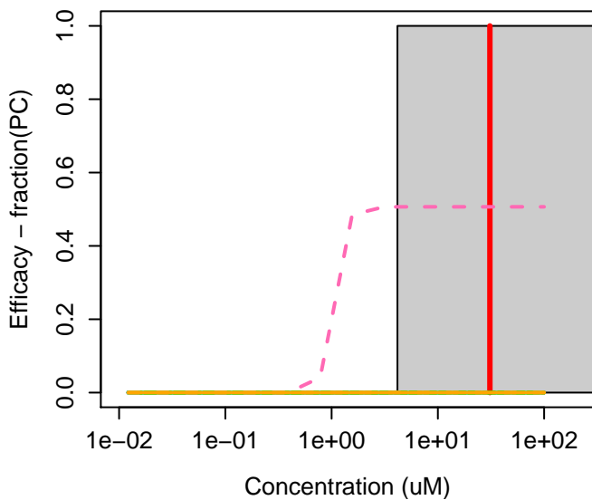
136042-19-8 : FR130739
