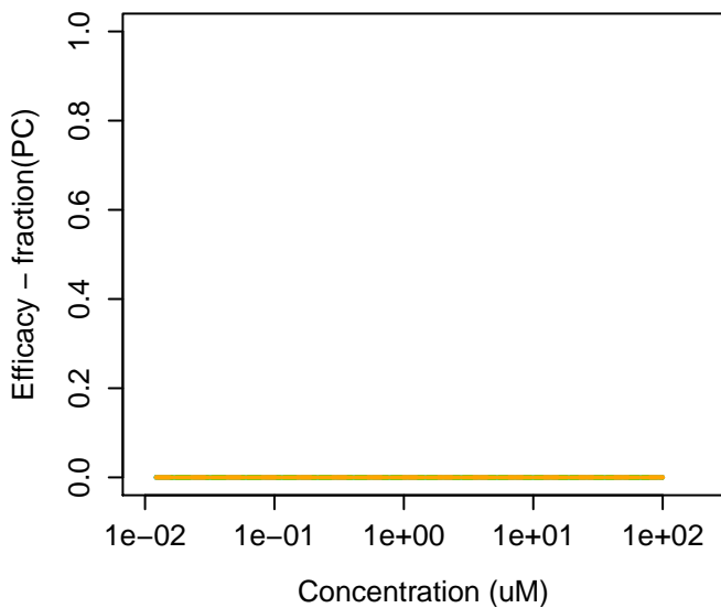
87-61-6 : 1,2,3-Trichlorobenzene
