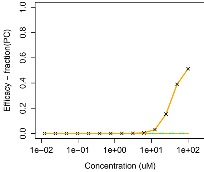
14371-10-9 : (2E)-3-Phenylprop-2-enal
