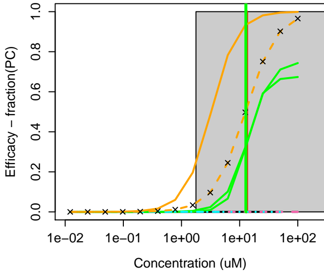
133-07-3 : Folpet
