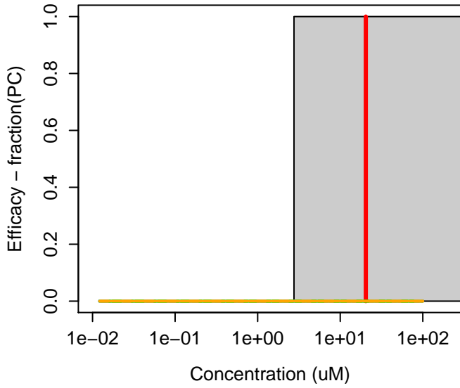
101-10-0 : Cloprop
