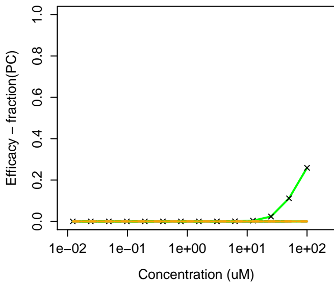
950-37-8 : Methidathion
