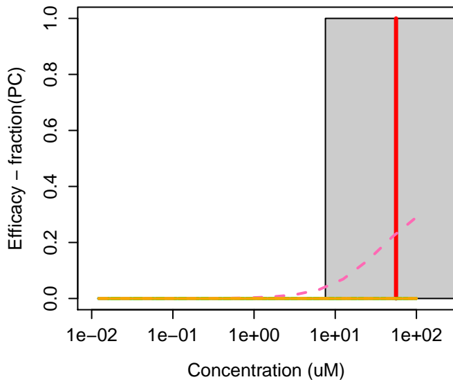
79-24-3 : Nitroethane
