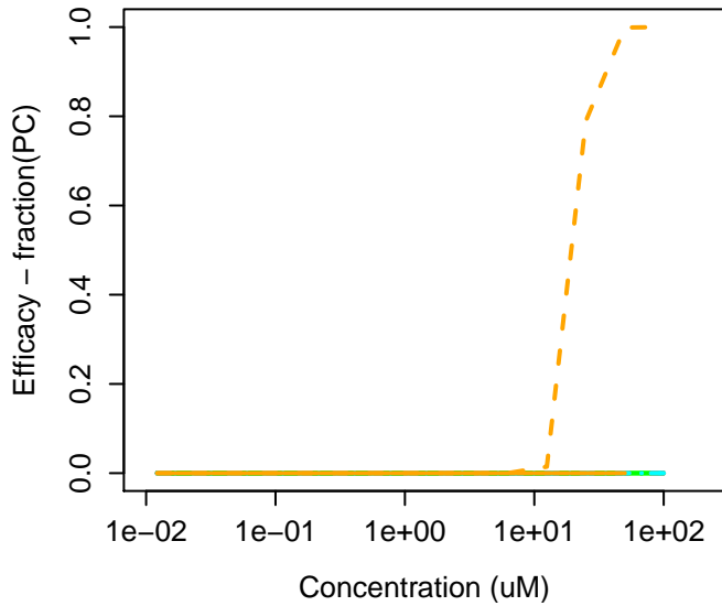
57-14-7 : 1,1-Dimethylhydrazine
