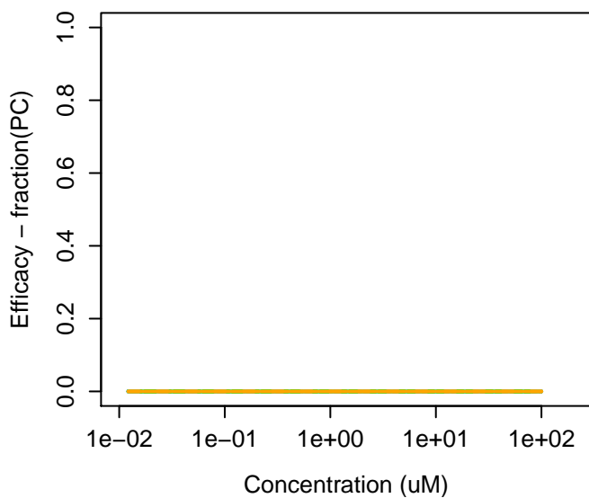
101-42-8 : Fenuron
