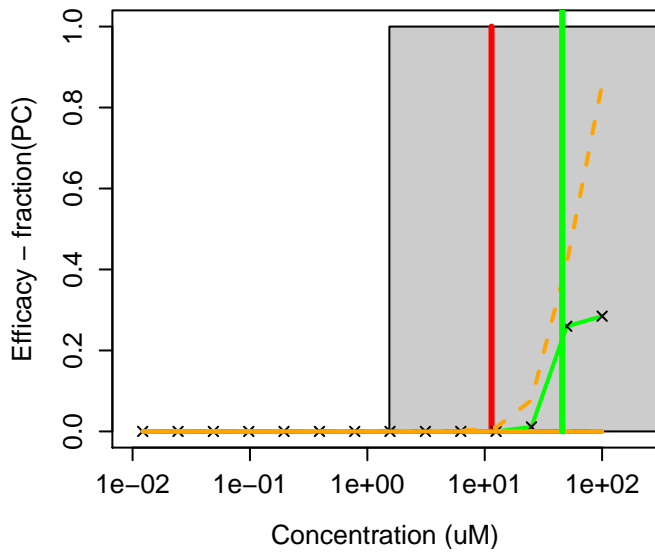
78-59-1 : Isophorone
