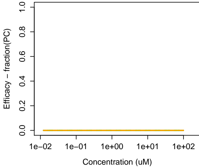
25155-18-4 : Methylbenzethonium chloride
