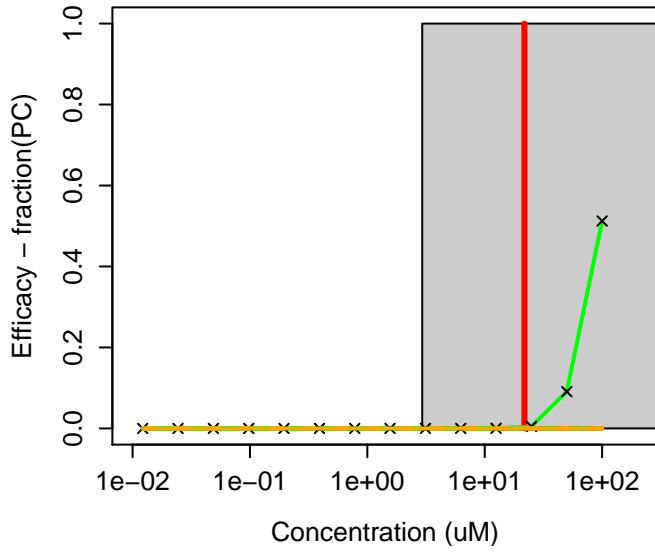
148-79-8 : Thiabendazole
