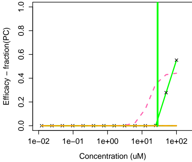
75330-75-5 : Lovastatin
