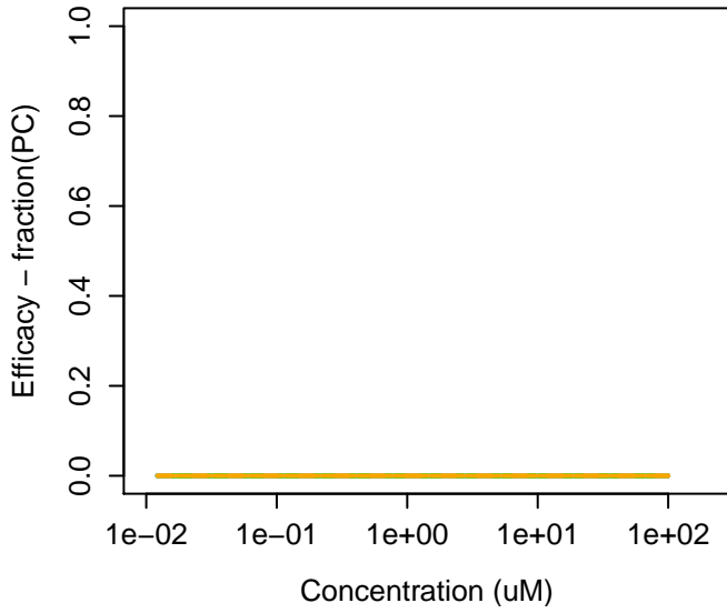
110-63-4 : 1,4-Butanediol
