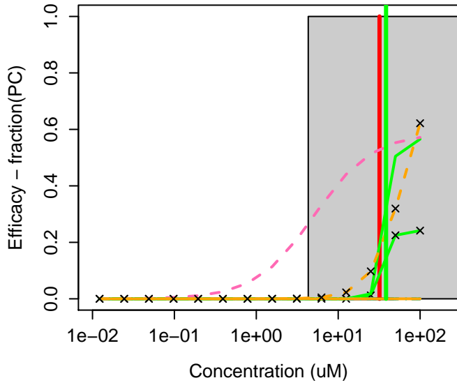
23103-98-2 : Pirimicarb
