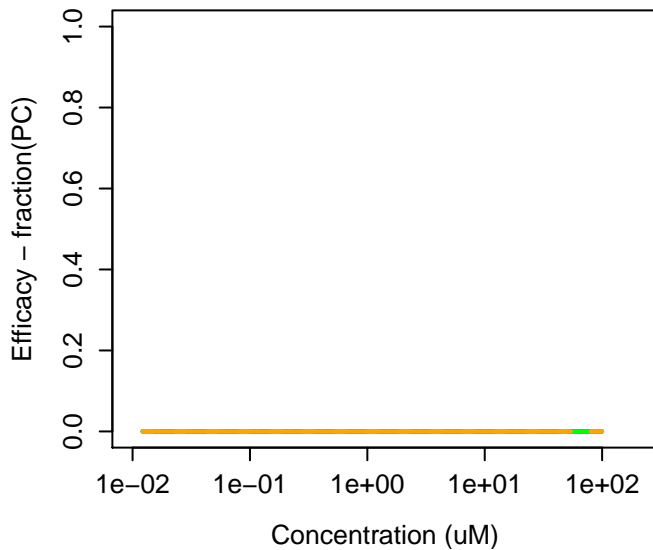
57-41-0 : 5,5-Diphenylhydantoin
