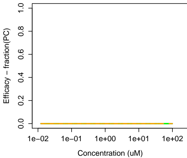
138-86-3 : Limonene
