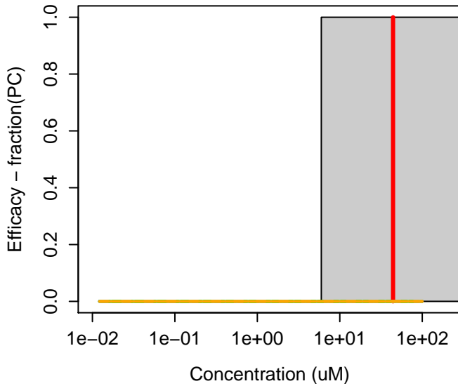
109-77-3 : Propanedinitrile
