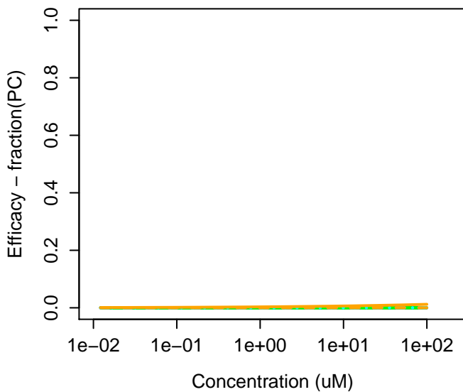
307-24-4 : PFHxA
