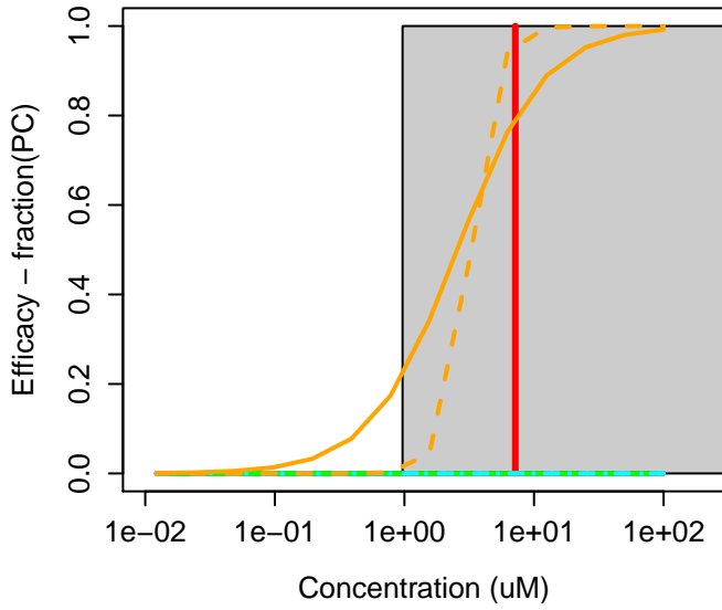
117718-60-2 : Thiazopyr
