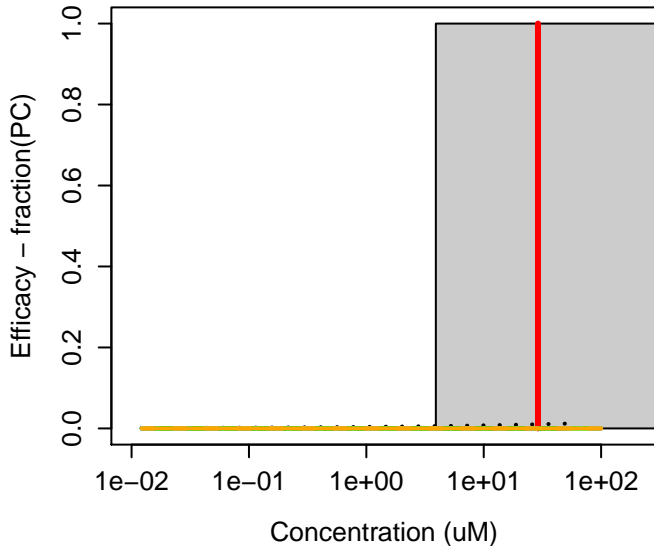
88-69-7 : 2-Isopropylphenol
