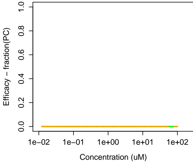
112281-77-3 : Tetraconazole
