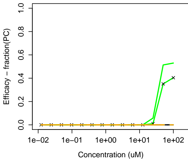
99-66-1 : Valproic acid
