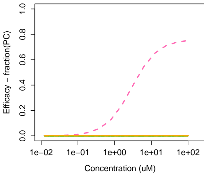
540-88-5 : tert-Butyl acetate
