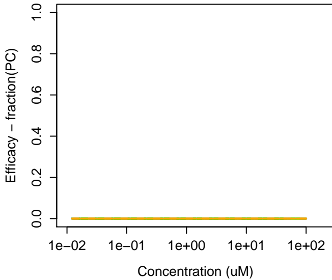
96182-53-5 : Tebupirimfos
