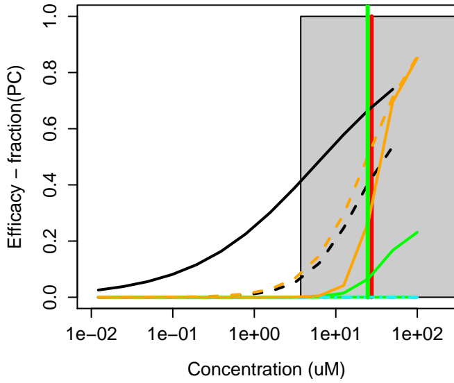
136-77-6 : 4-Hexylresorcinol
