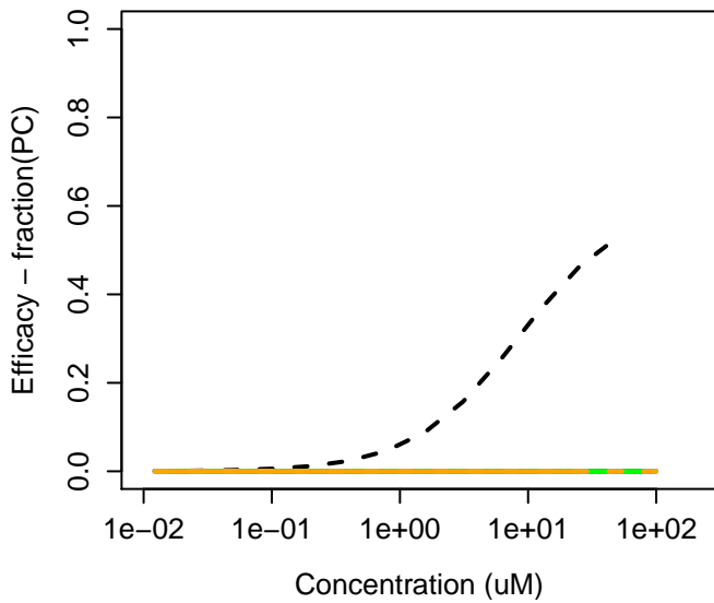
112809-51-5 : Letrozole
