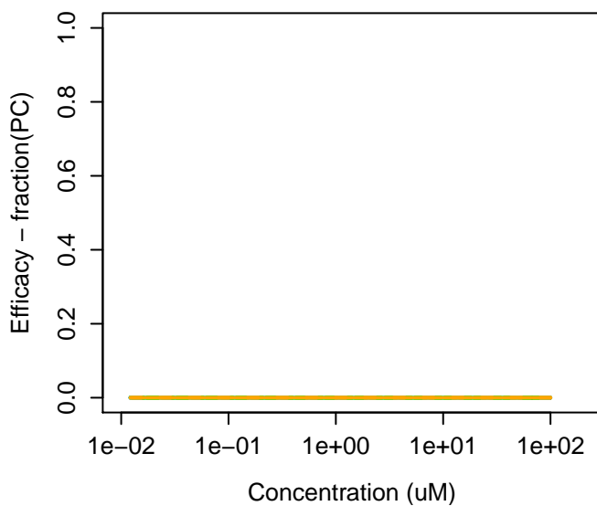
55589-62-3 : Acesulfame potassium
