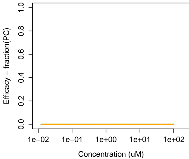
114-26-1 : Propoxur
