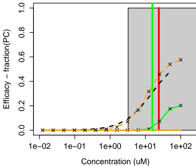
99-30-9 : Dicloran
