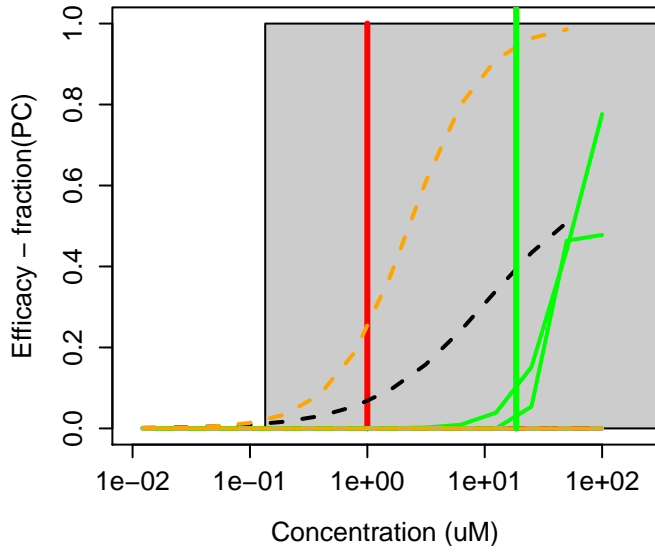
61791-12-6 : Cremophor EL
