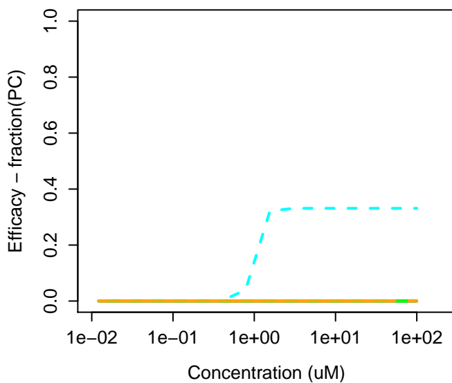
69-72-7 : Salicylic acid
