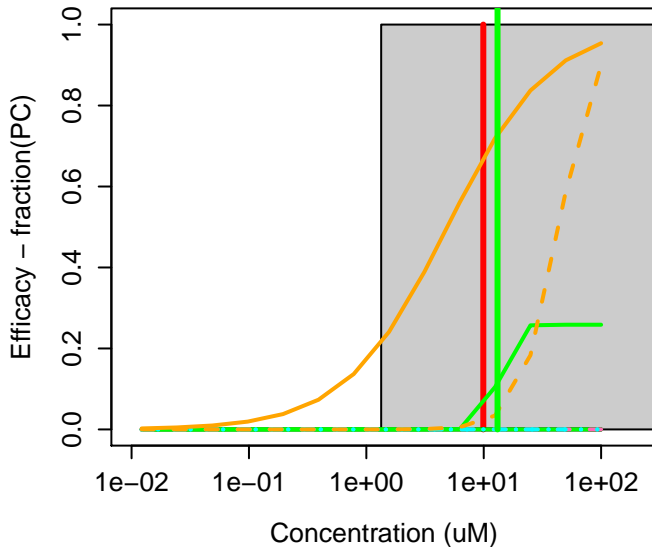
288-32-4 : Imidazole
