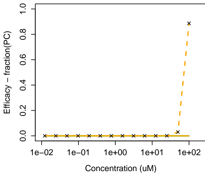
541-73-1 : 1,3-Dichlorobenzene
