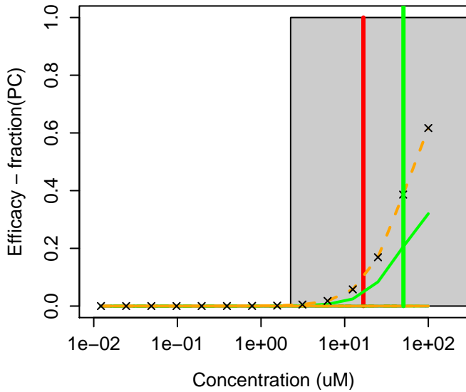
55285-14-8 : Carbosulfan
