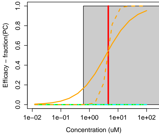
141-66-2 : Dicrotophos
