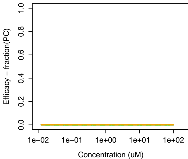
499-75-2 : Isopropyl-o-cresol
