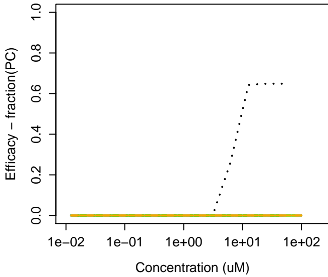
79622-59-6 : Fluazinam
