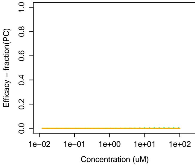
123-92-2 : 3-Methylbutyl acetate
