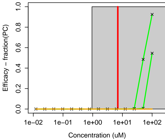
142-16-5 : Bis(2-ethylhexyl) maleate
