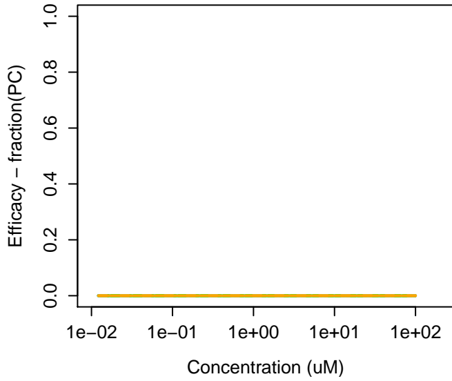
112-50-5 : 2-[2-(2-Ethoxyethoxy)ethoxy]ethano
