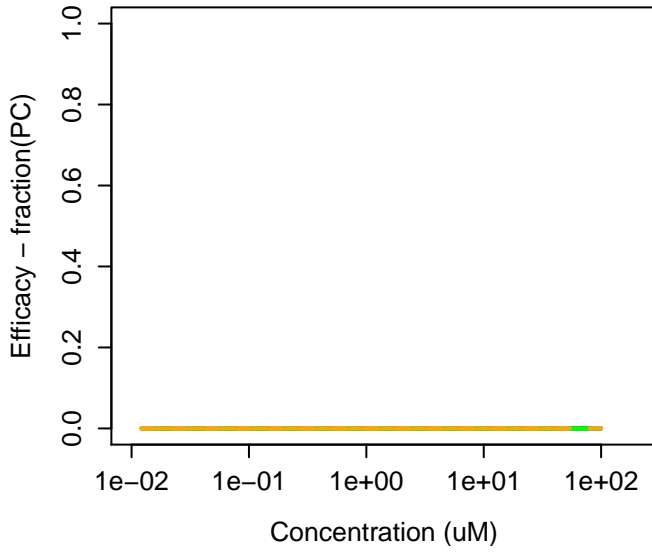
124-09-4 : 1,6-Hexanediamine
