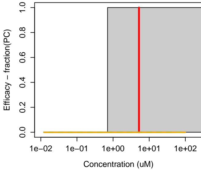
6624-73-3 : Pentane-1,5-diyl dibenzoate
