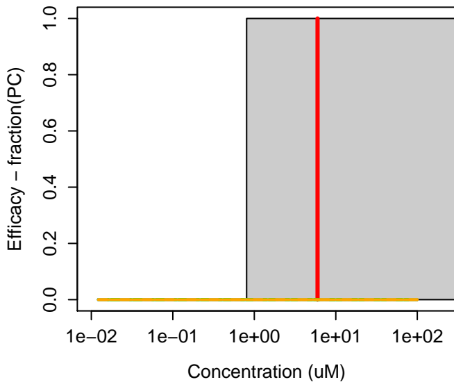
1111-78-0 : Ammonium carbamate
