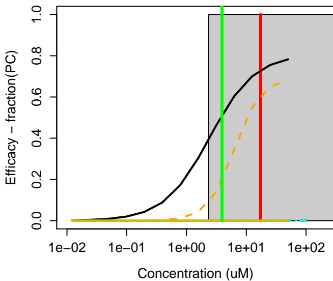
56-38-2 : Parathion
