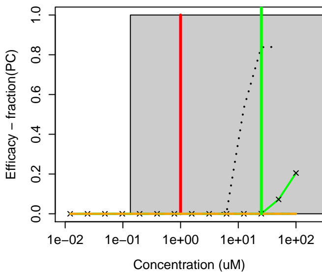
463-40-1 : Linolenic acid
