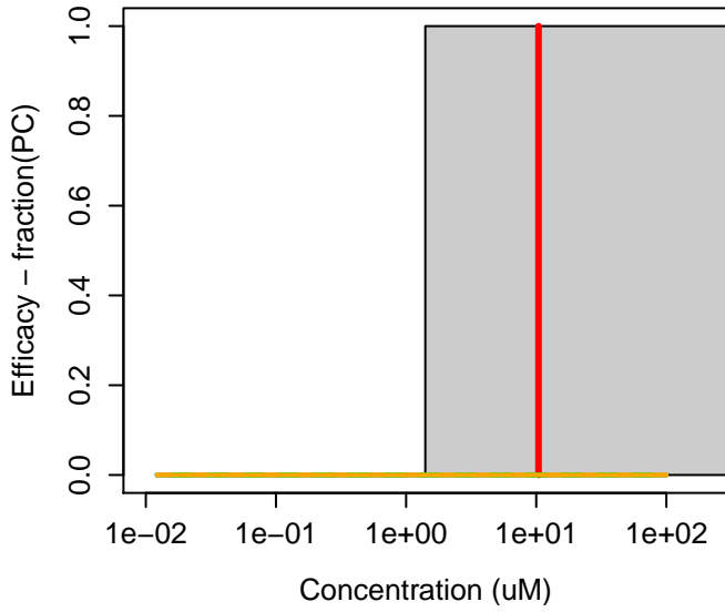
106-48-9 : 4-Chlorophenol
