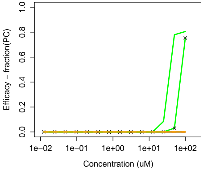
12427-38-2 : Maneb
