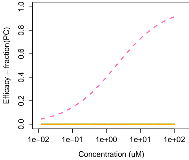
103-34-4 : 4,4'-Dithiodimorpholine
