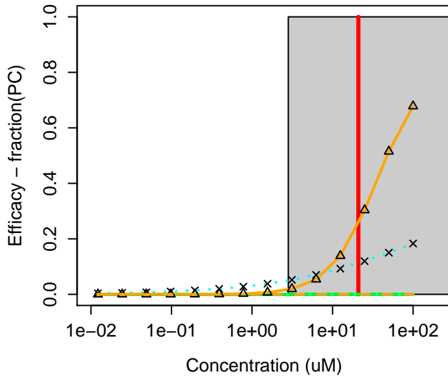
487-06-9 : 5,7-Dimethoxy-2H-chromen-2-one
