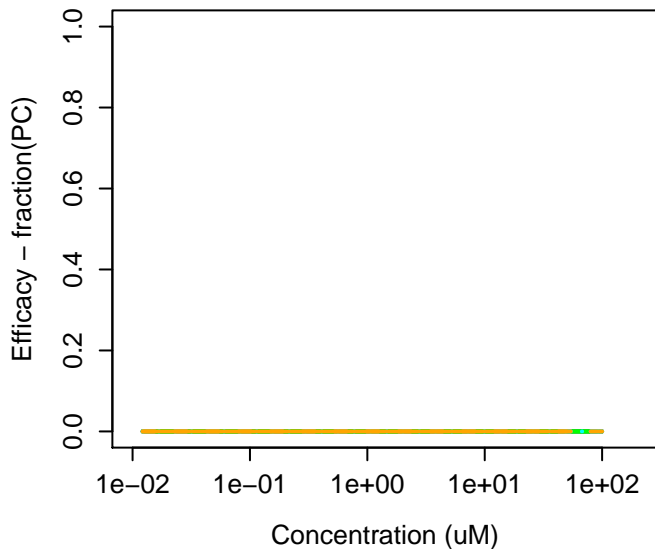
124-04-9 : Hexanedioic acid
