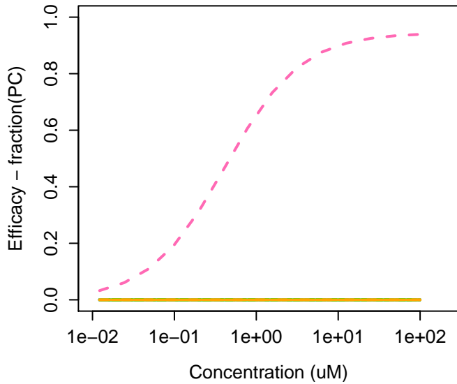
1563-66-2 : Carbofuran
