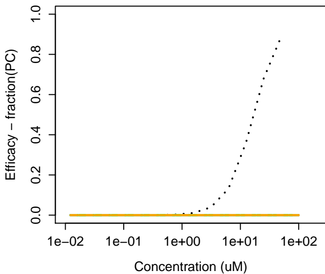
6149-03-7 : Sodium 4-octylbenzenesulfonate
