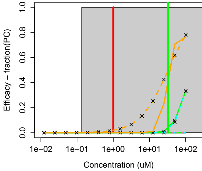
90357-06-5 : Bicalutamide
