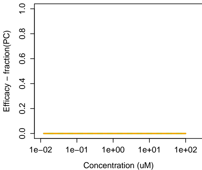
822-06-0 : 1,6-Diisocyanatohexane
