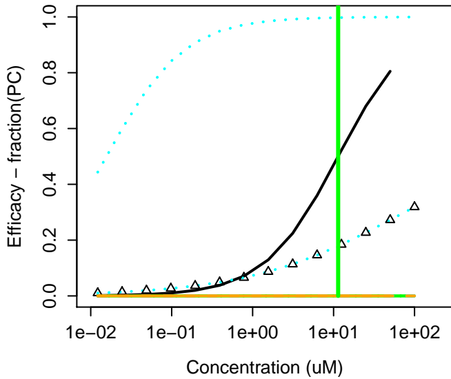
125116-23-6 : Metconazole
