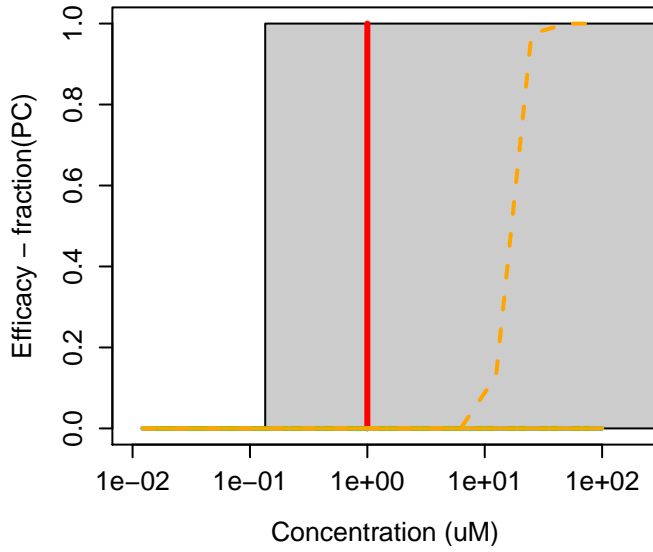
464-49-3 : D-Camphor
