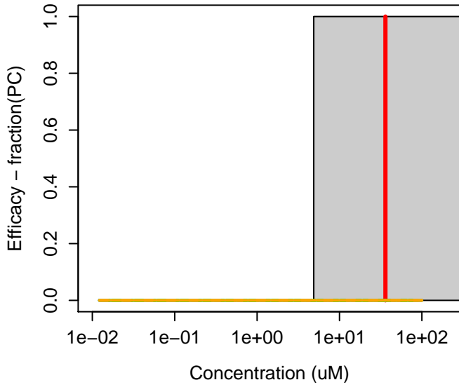
75-64-9 : tert-Butylamine
