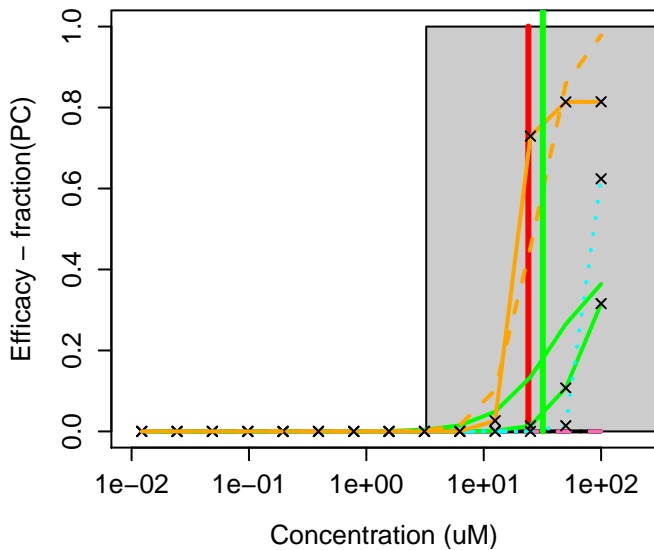
23593-75-1 : Clotrimazole
