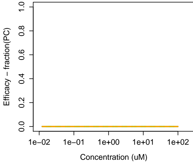
1646-88-4 : Aldoxycarb
