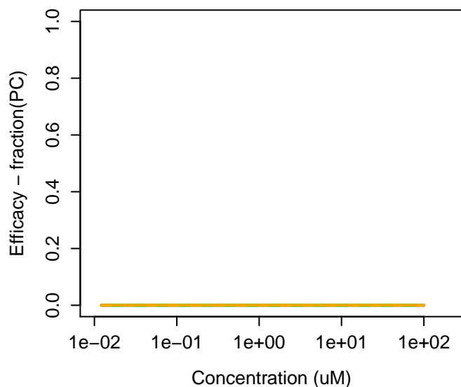
78-70-6 : Linalool
