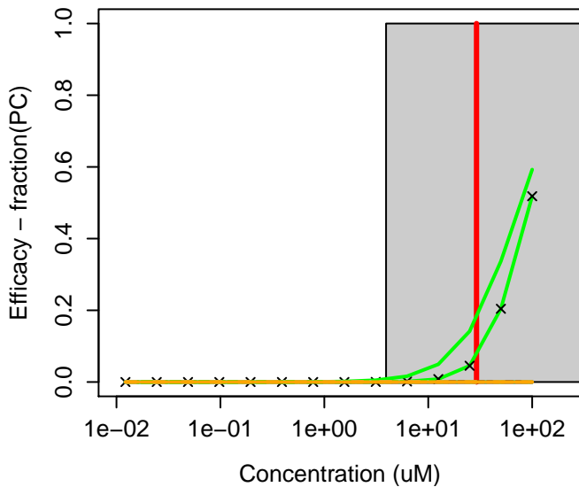
1806-26-4 : 4-Octylphenol
