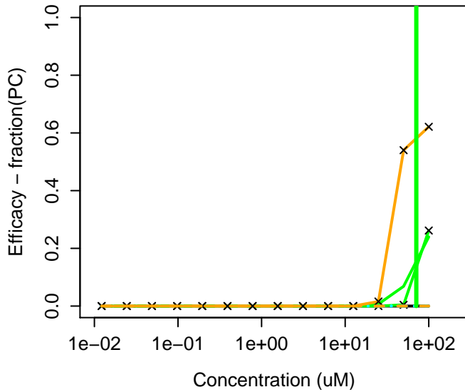
34014-18-1 : Tebuthiuron
