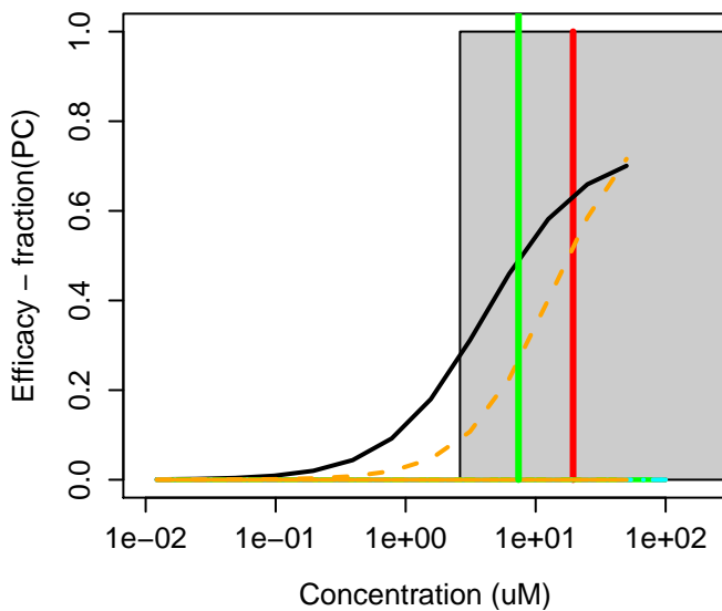
55-38-9 : Fenthion
