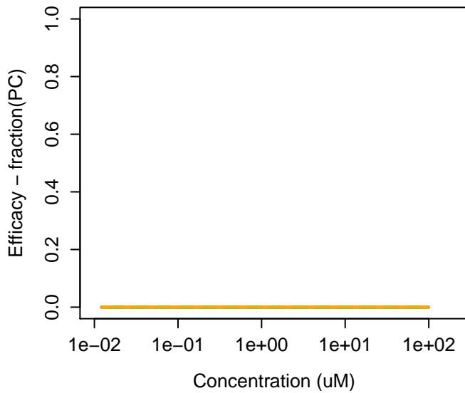
2550-40-5 : Dicyclohexyl disulfide
