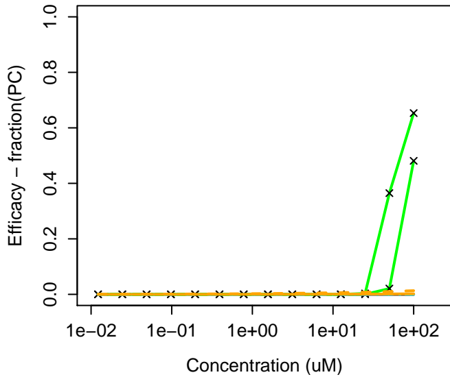
17465-86-0 : gamma-Cyclodextrin
