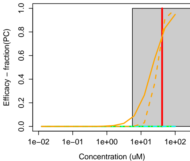
68157-60-8 : Forchlorfenuron
