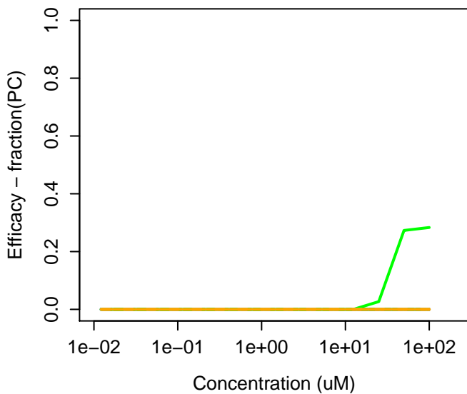
51235-04-2 : Hexazinone
