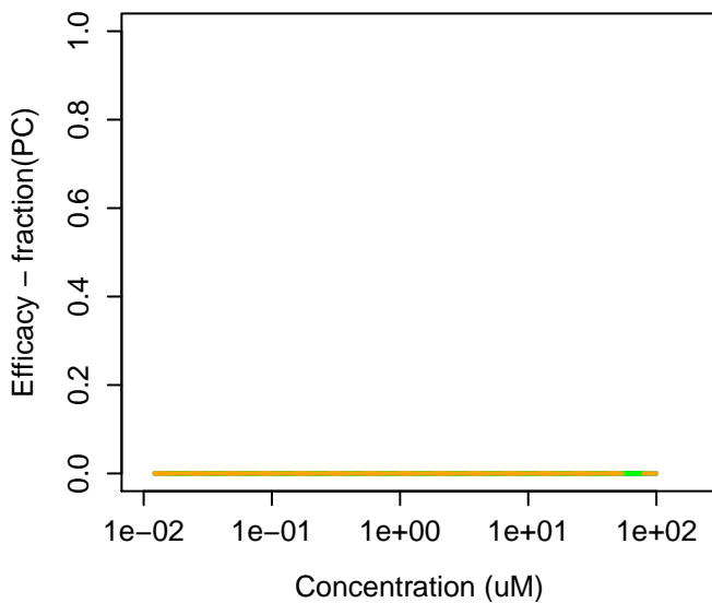
111-40-0 : Diethylenetriamine
