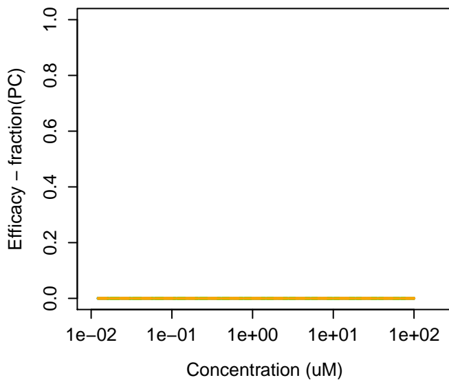
16672-87-0 : Ethephon
