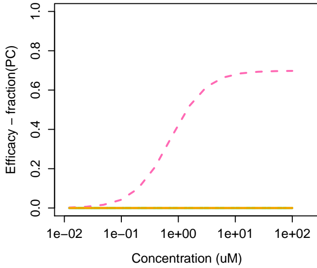
7758-19-2 : Sodium chlorite
