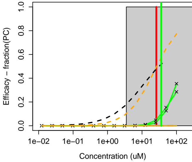
53-16-7 : Estrone
