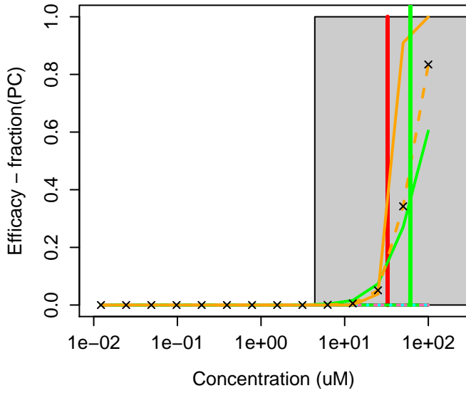
69377-81-7 : Fluroxypyr
