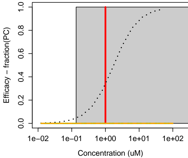
302-79-4 : all-trans-Retinoic acid
