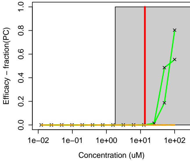
59-67-6 : Nicotinic acid
