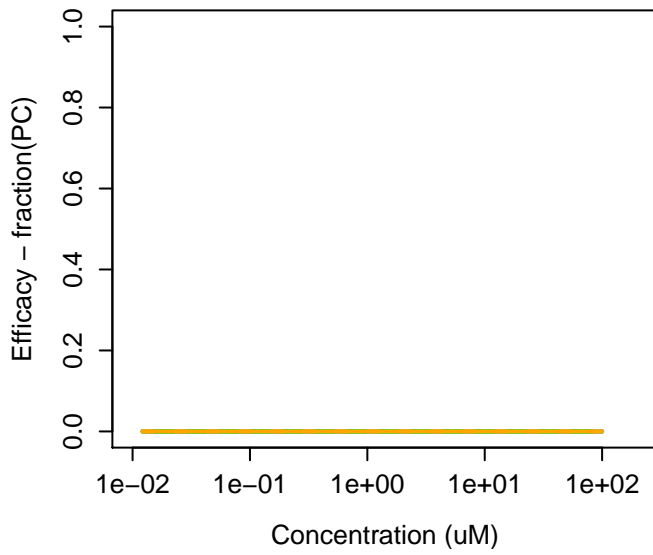
4065-45-6 : Sulisobenzone
