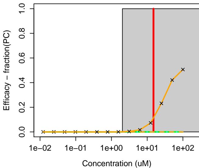
23950-58-5 : Propyzamide
