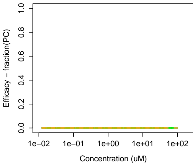
420-04-2 : Cyanamide
