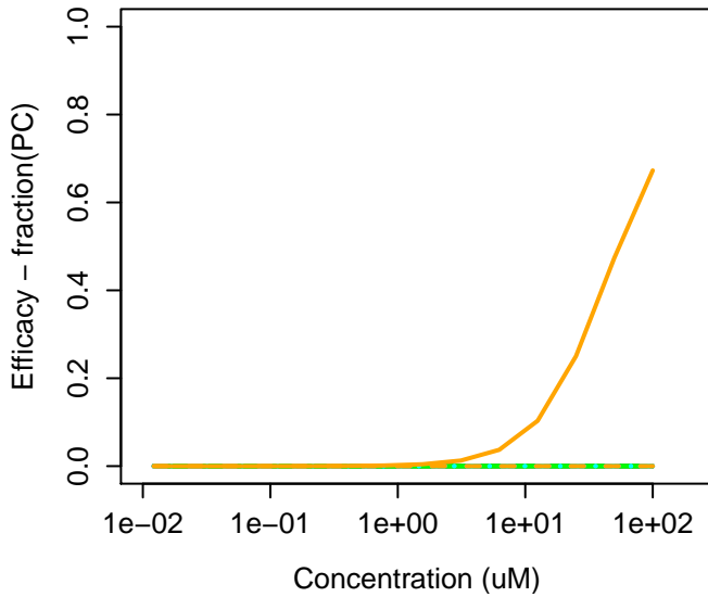
120-47-8 : Ethylparaben
