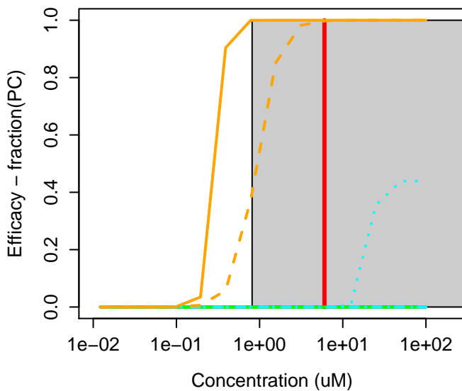
3811-73-2 : Sodium (2-pyridylthio)-N-oxide
