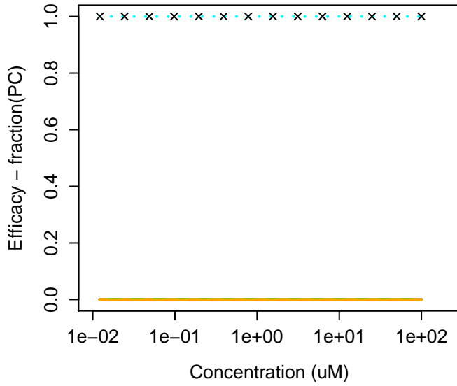
127-07-1 : Hydroxyurea
