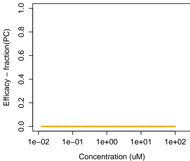
1120-21-4 : Undecane
