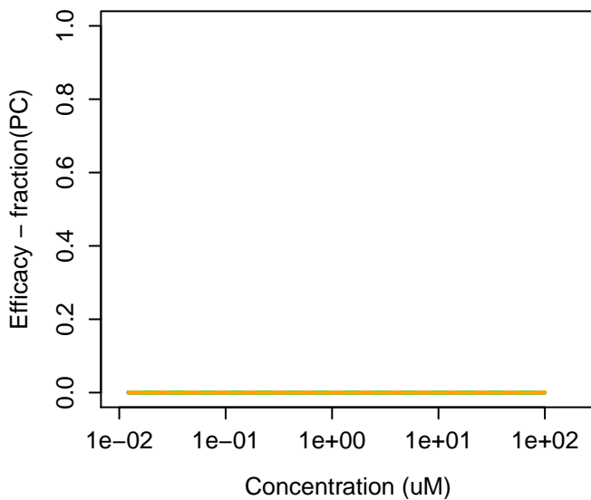
123122-55-4 : Candoxatriol
