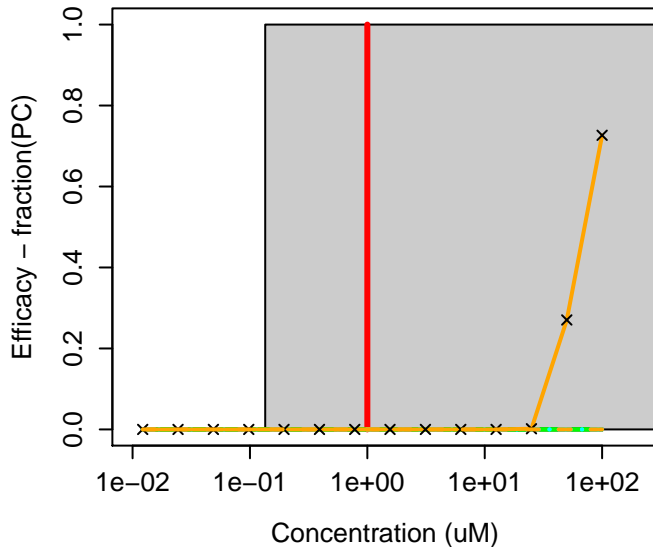
99-62-7 : 1,3-Diisopropylbenzene
