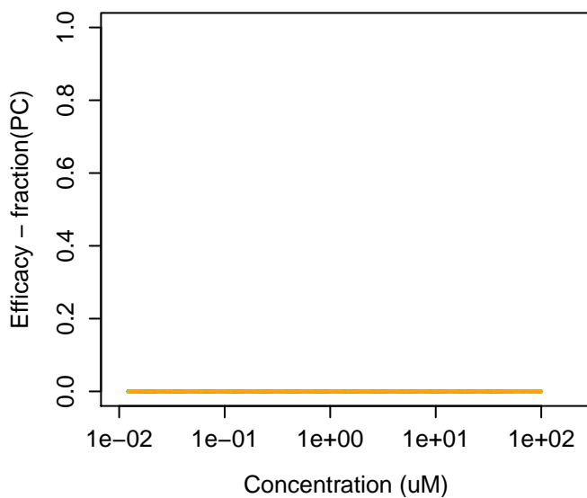
4098-71-9 : Isophorone diisocyanate
