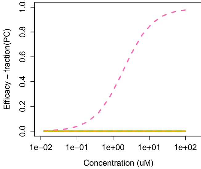
754-91-6 : PFOSA
