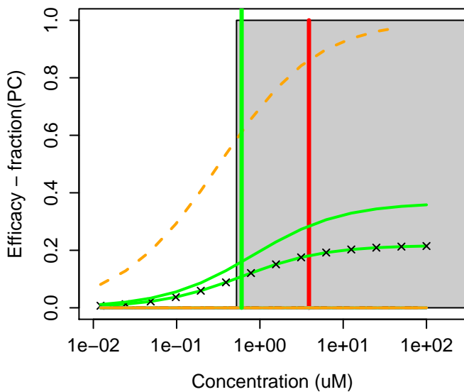
66-81-9 : Cycloheximide
