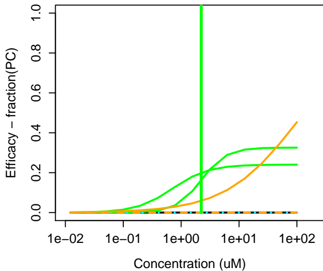
122008-85-9 : Cyhalofop-butyl
