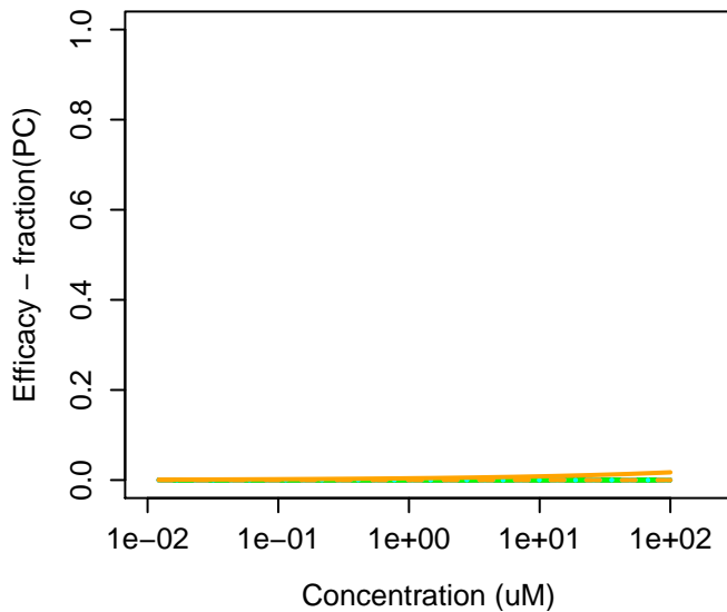
1112-39-6 : Dimethoxydimethylsilane
