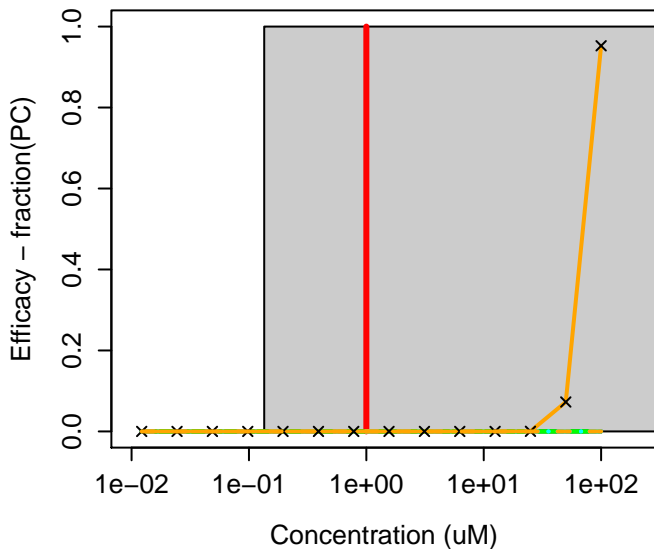
625-55-8 : Isopropyl formate
