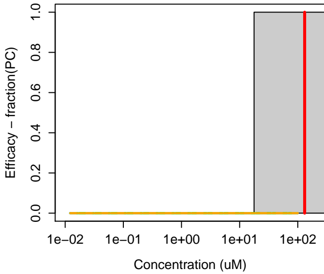
65-23-6 : Pyridoxine
