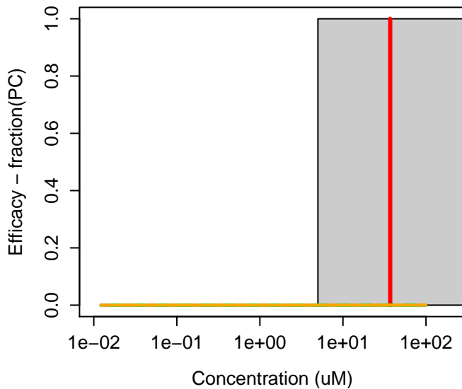
1260-17-9 : Carminic acid
