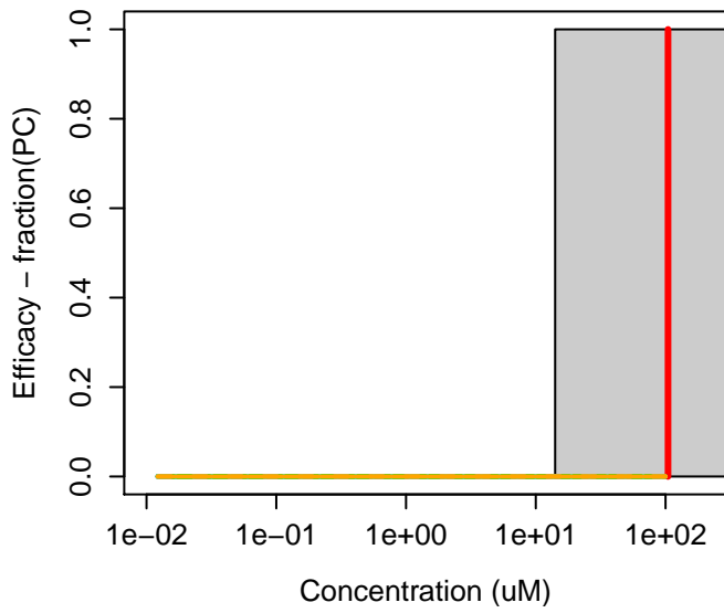
1166-52-5 : Dodecyl gallate
