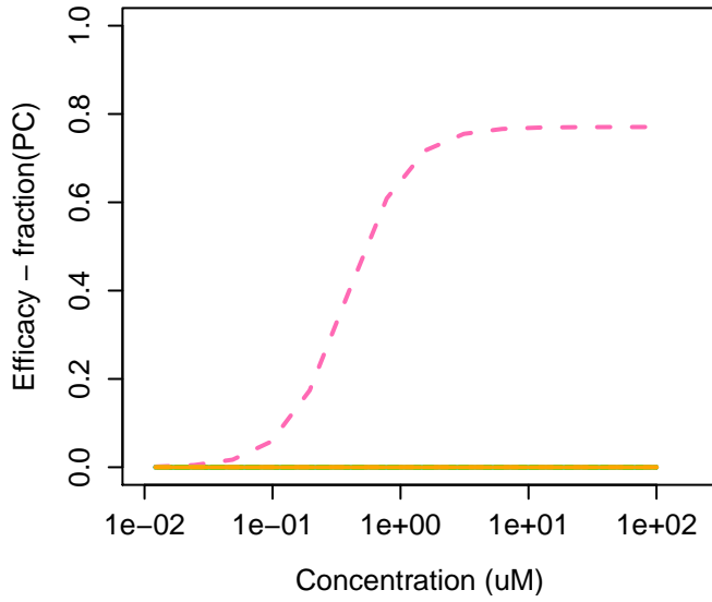
77-86-1 : Tromethamine
