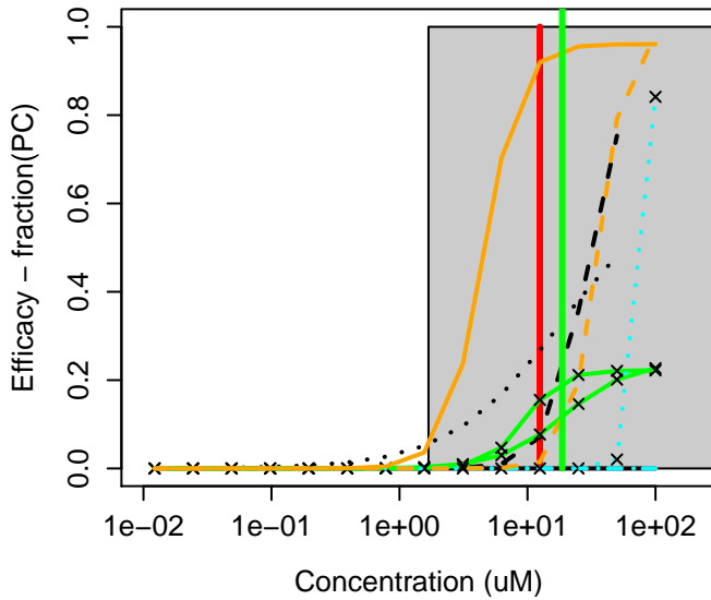
5700-49-2 : 1,2-Ethanediamine dihydriodide
