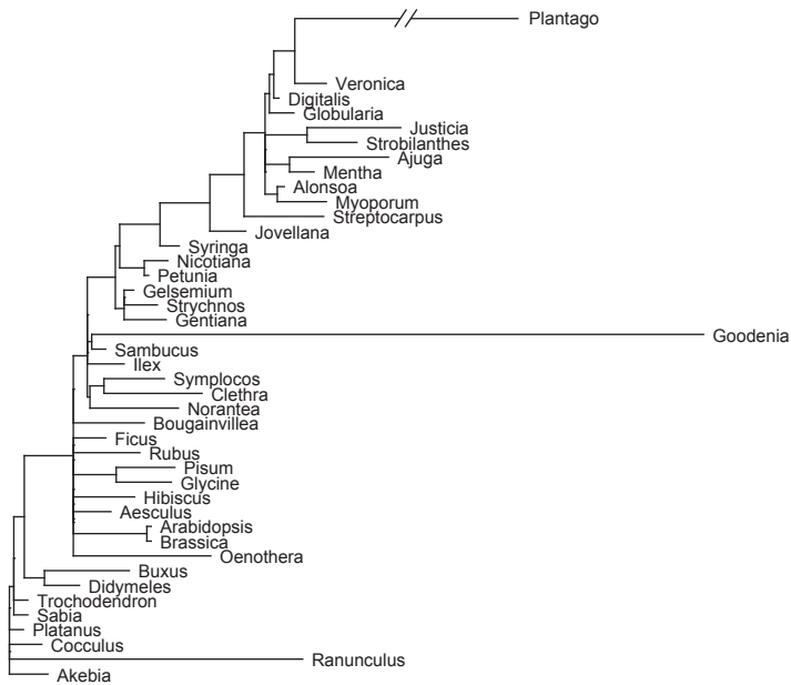
mt SSU rDNA
