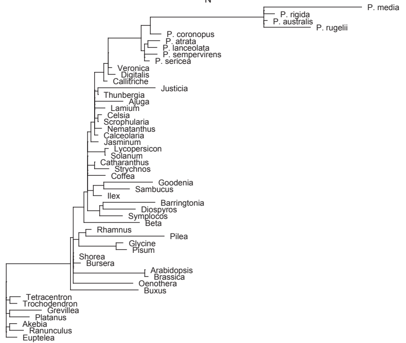
mt atp1 - d_N
