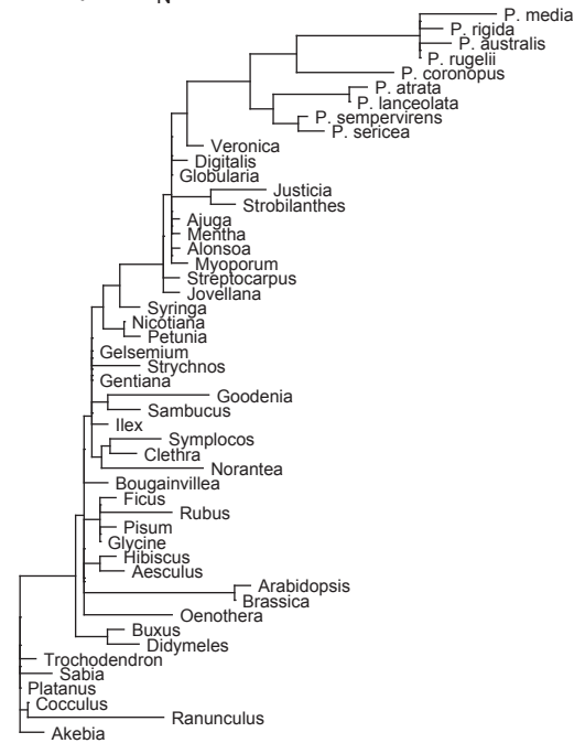
mt atp1 - d_N
