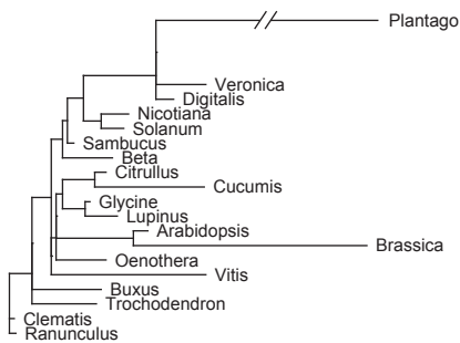
mt SSU rDNA
