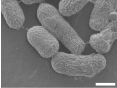
NCR162pl 3.7
