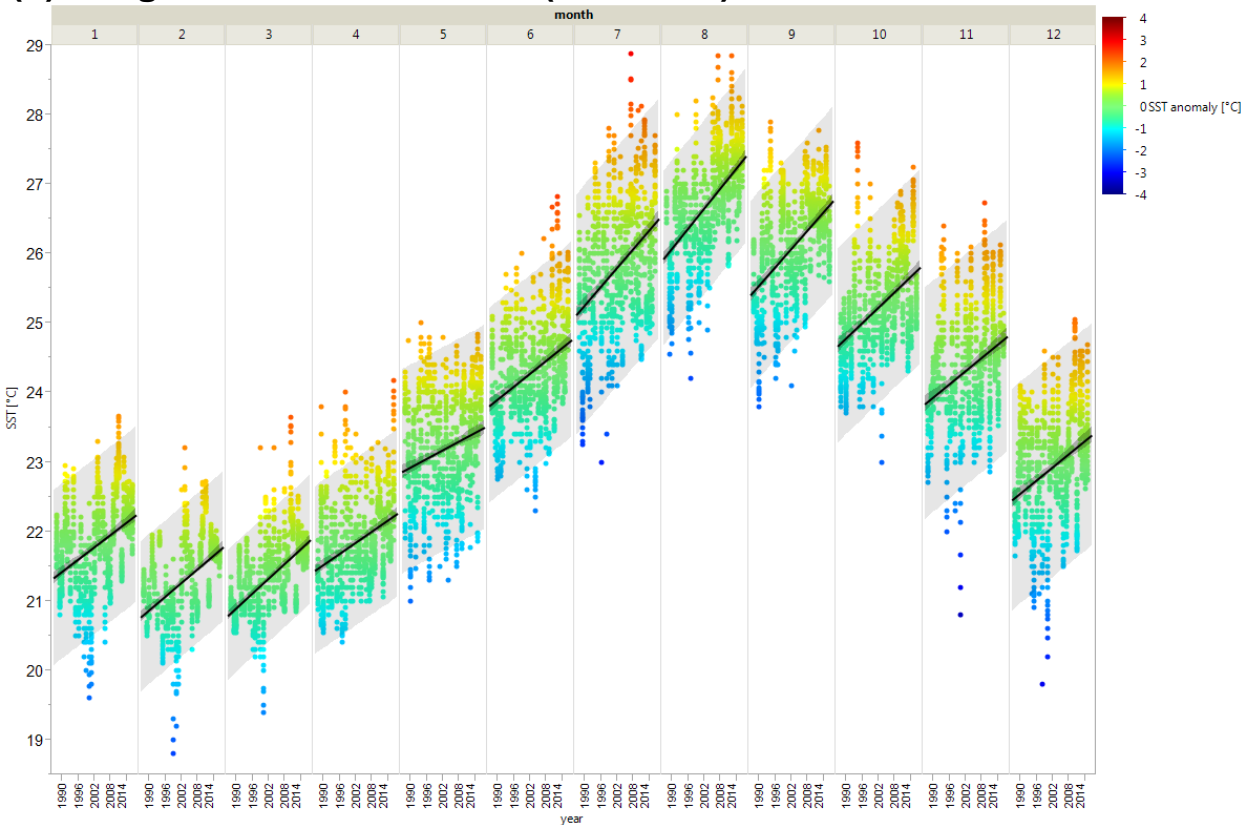
(d) Long-term SST in the GoA (Eilat area) 1988-2016
