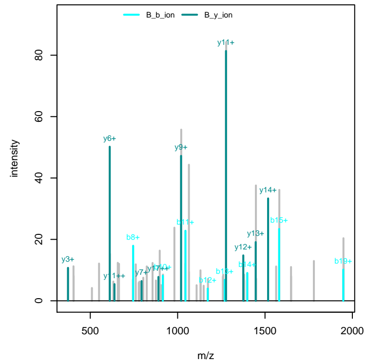
GEILGGM o AAVEQPEKPAAPK+XL_S
