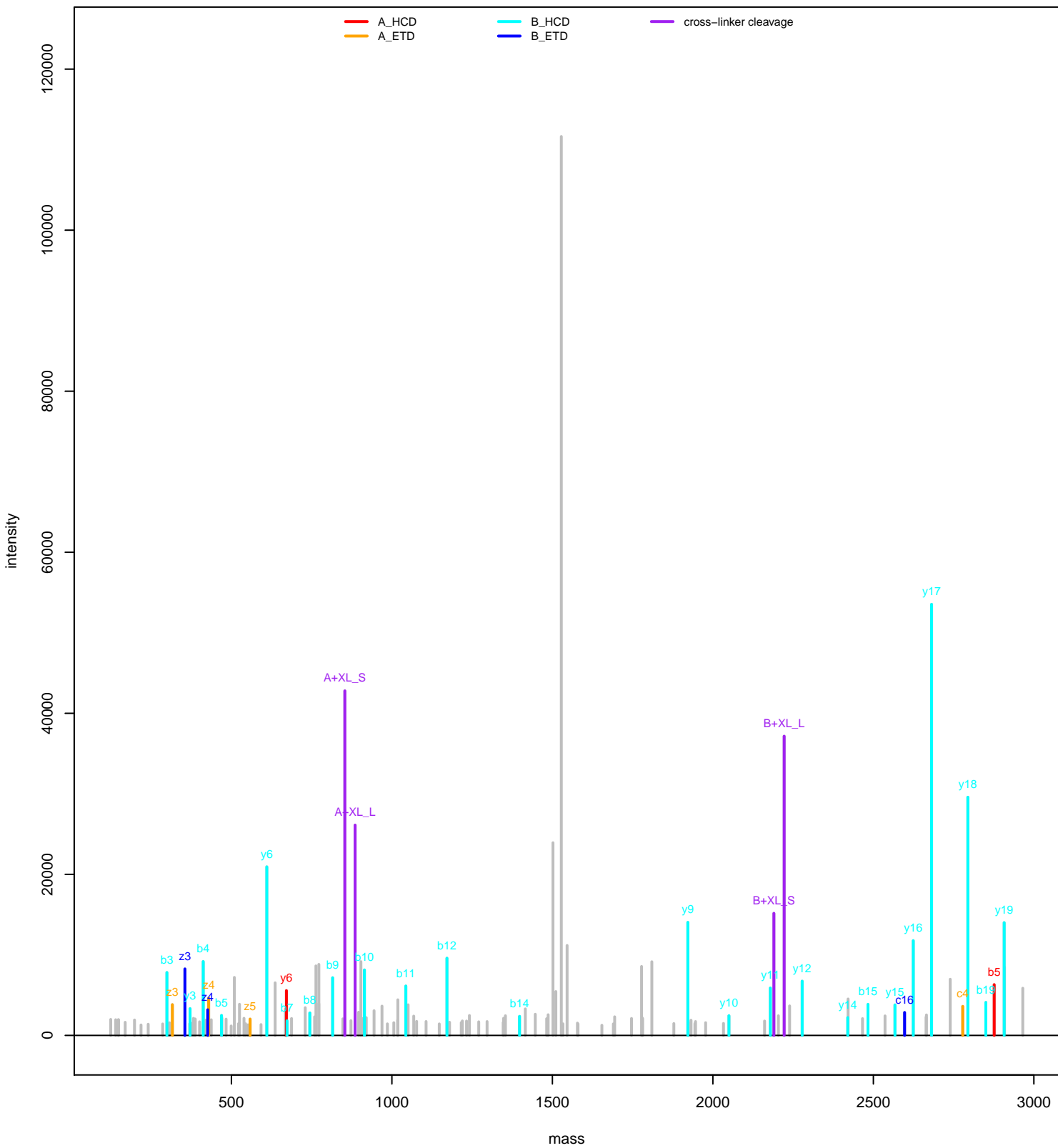
KPELDAK GEILGGM o AAVEQPEKPAAPK
