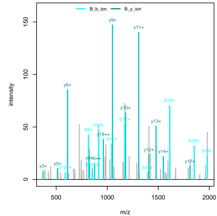
GEILGGM o AAVEQPEKPAAPK+XL_L
