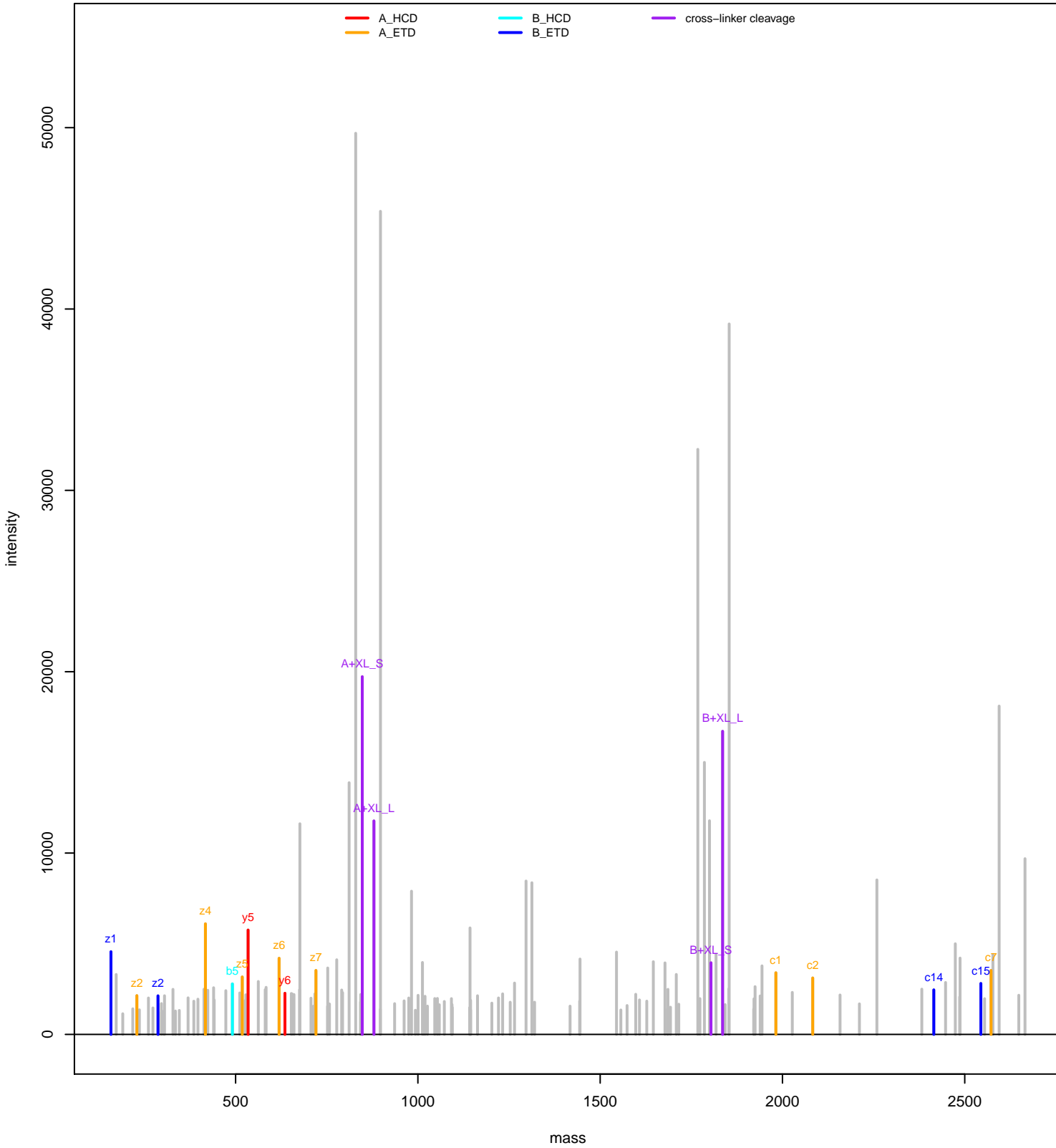
GTTTMGVK GTTTMGVKLD DATRER
