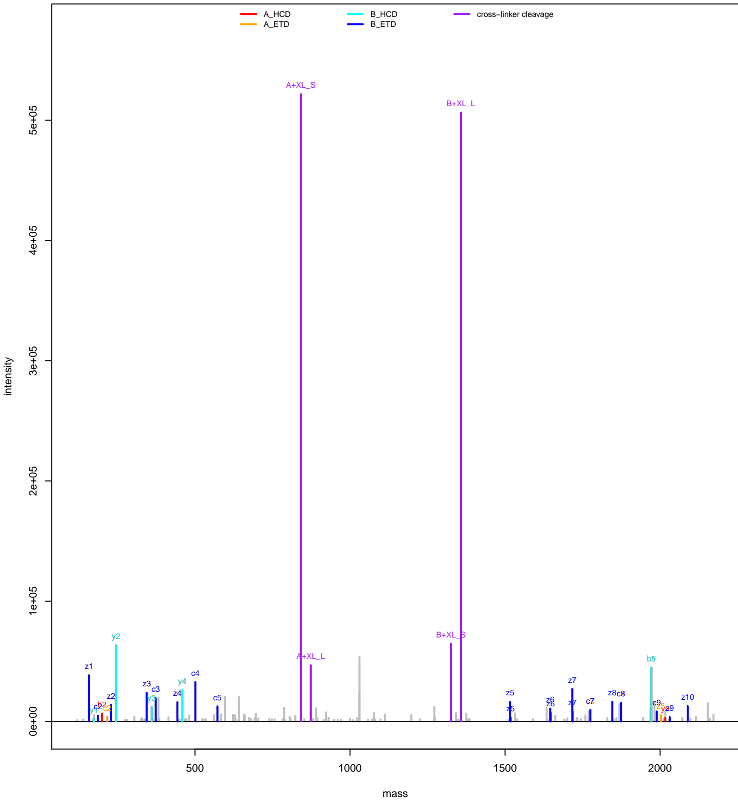
AEKVDAR LGWKA EKVDAR
