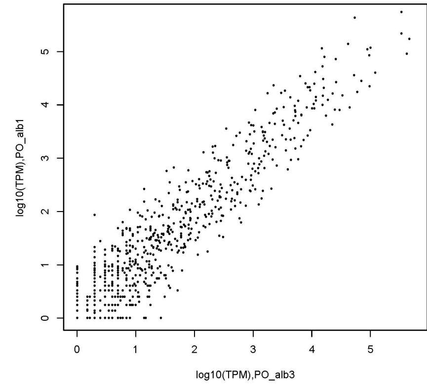
PO_alb3vsPO_alb1,R=0.668080611075564
