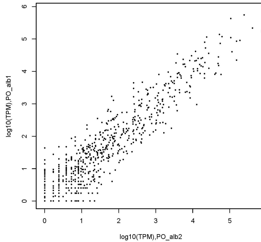
PO_alb2vsPO_alb1,R=0.645041740586478
