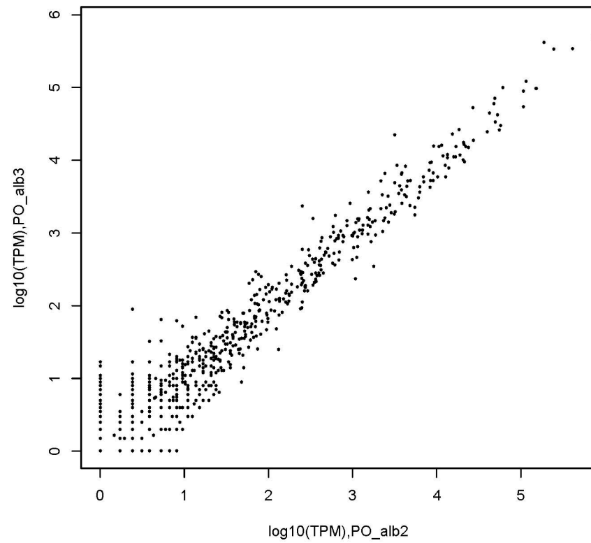
PO_alb2vsPO_alb3,R=0.89962672646609
