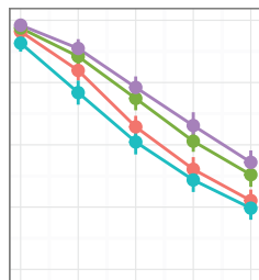
Klekota-Roth
