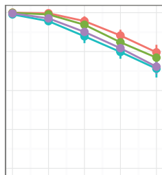
PUBCHEM
