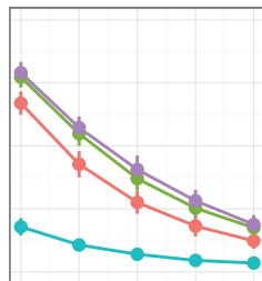
ECFP2
