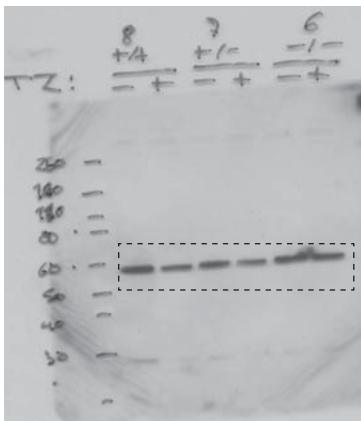
Figure 3E_ZBP1 (Zippy-1)
