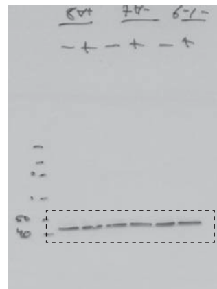
Figure 3E_ACTB
