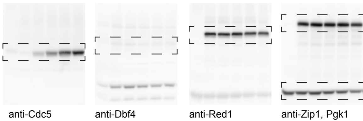
Fig. 6D. ndt80 dbf4-md bob1
