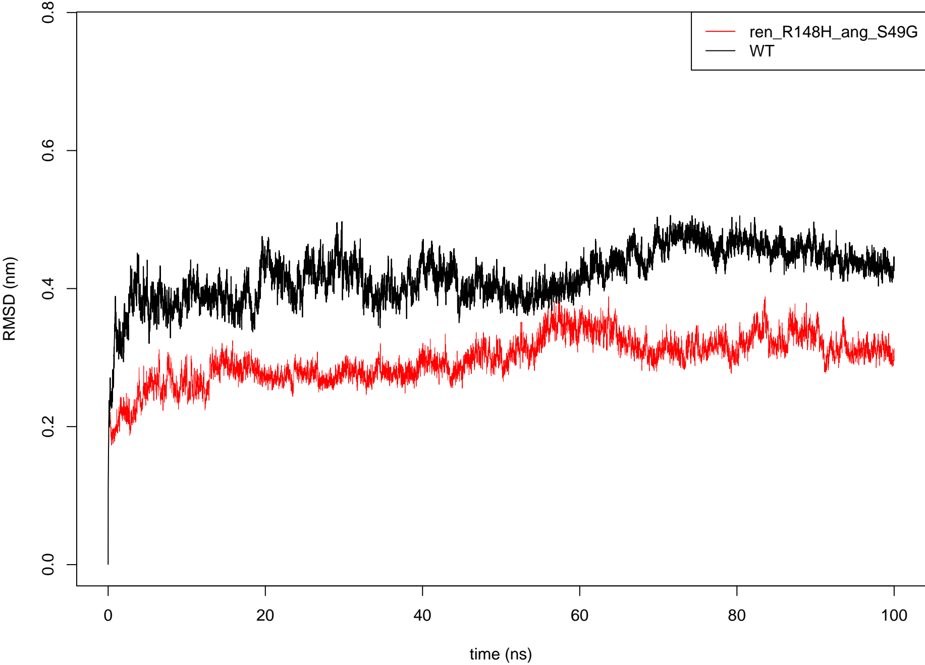
C alpha RMSD: ren_R148H_ang_S49G vs WT
