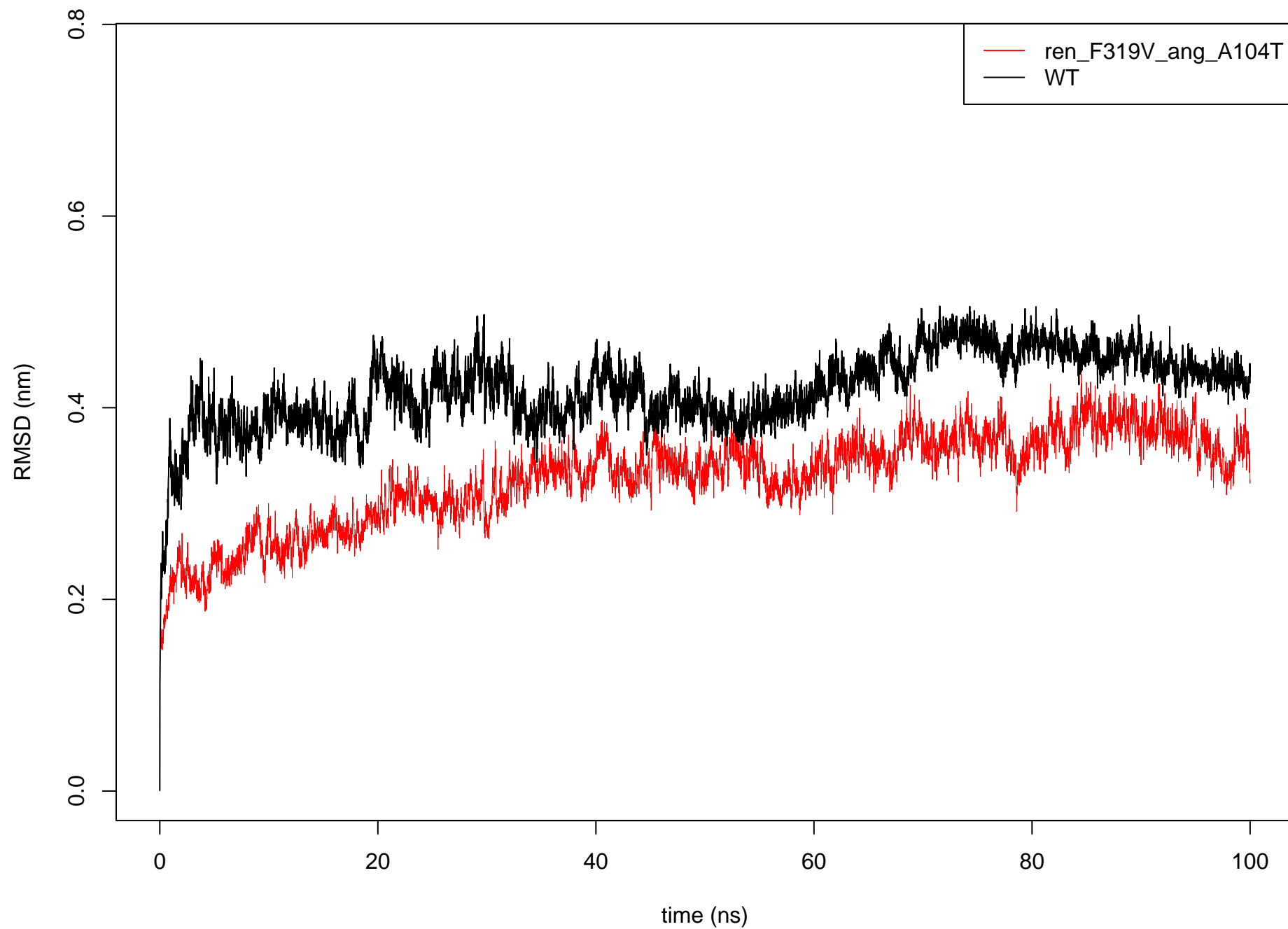
C alpha RMSD: ren_F319V_ang_A104T vs WT
