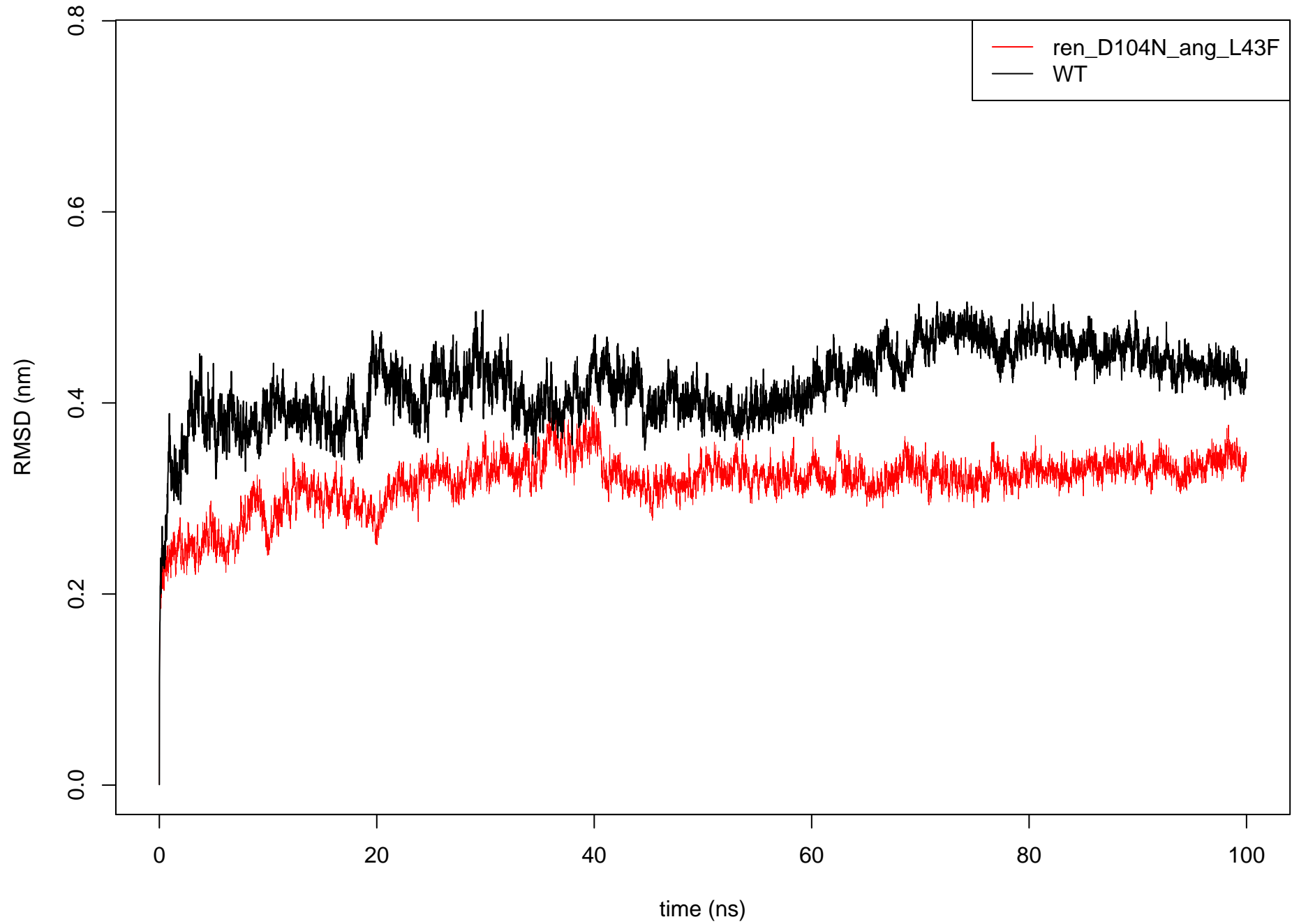
C alpha RMSD: ren_D104N_ang_L43F vs WT
