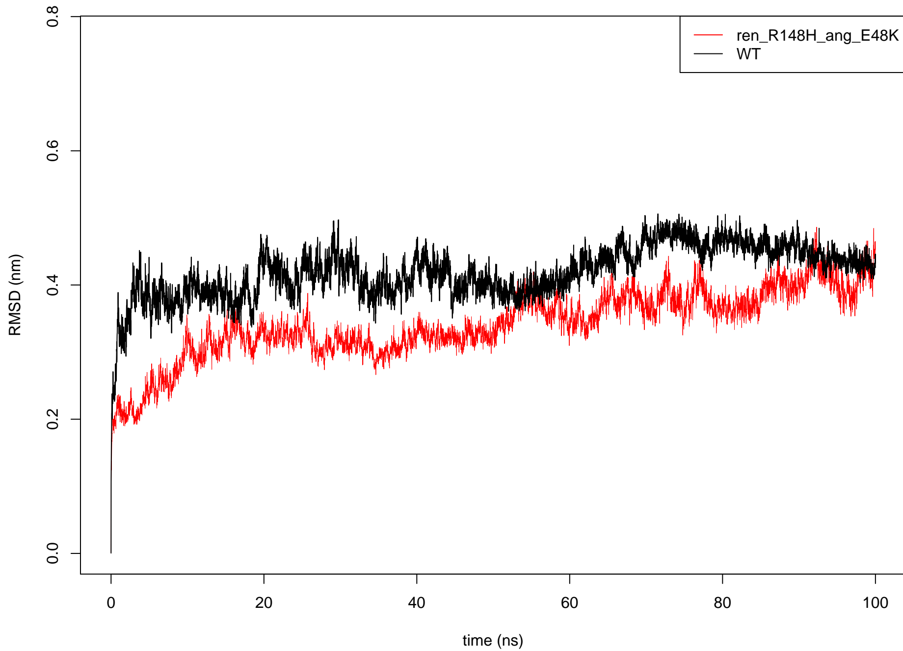
C alpha RMSD: ren_R148H_ang_E48K vs WT
