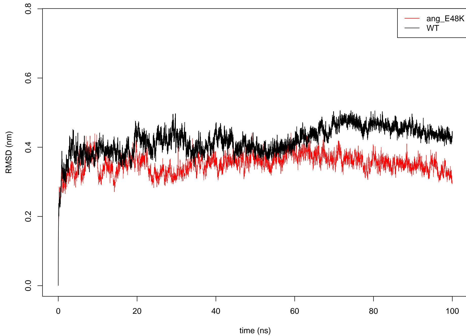
C alpha RMSD: ang_E48K vs WT
