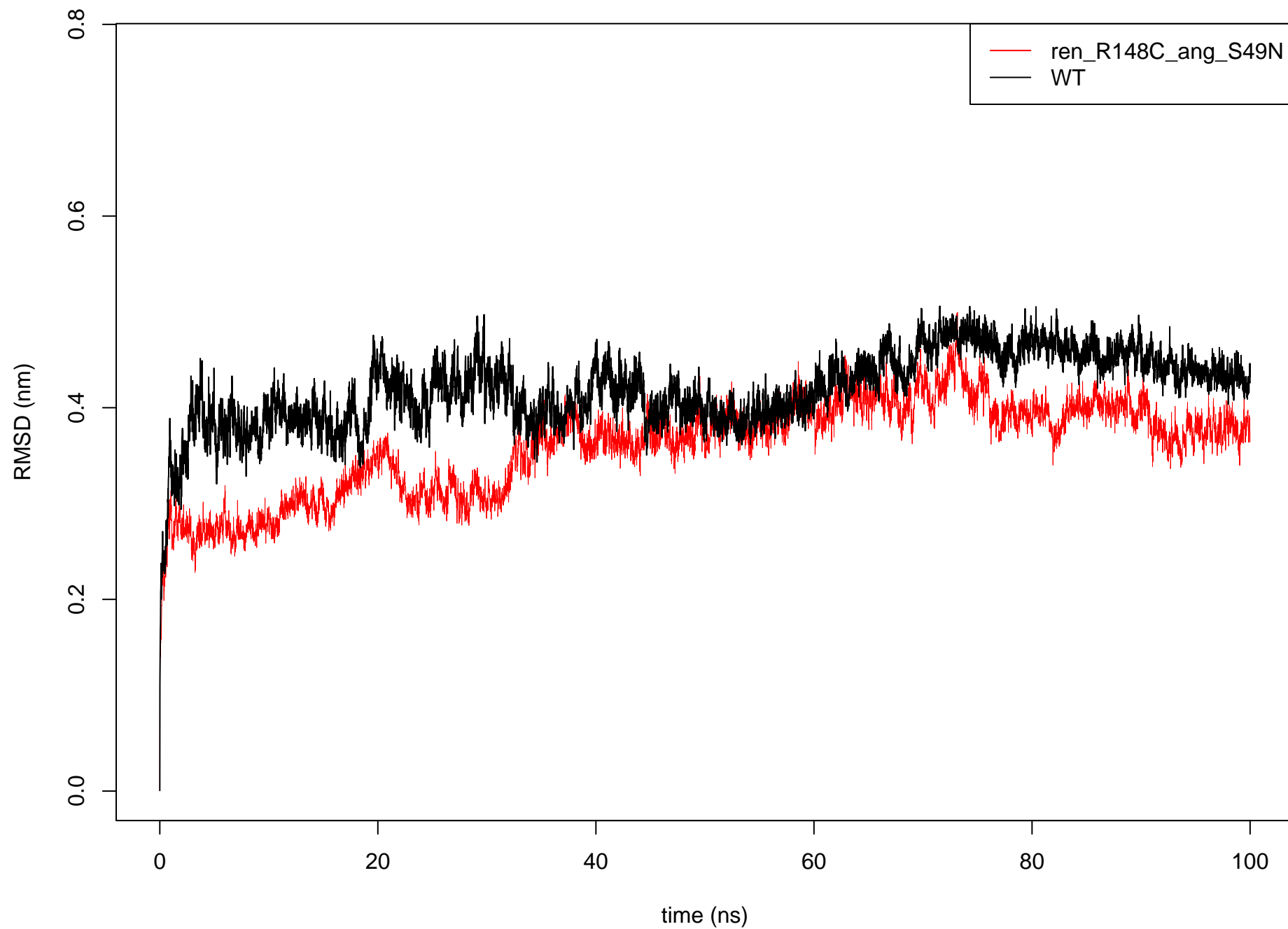
C alpha RMSD: ren_R148C_ang_S49N vs WT
