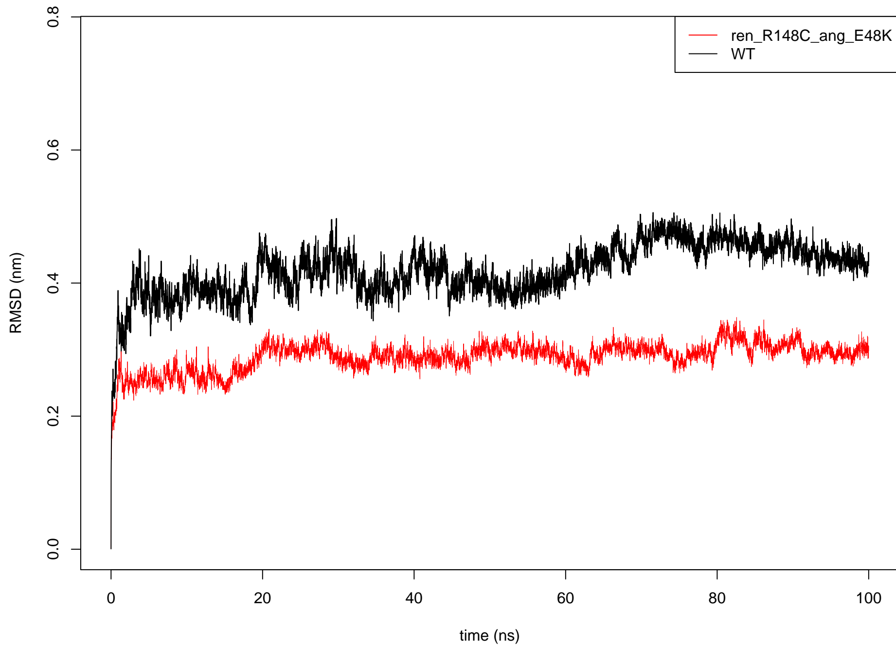
C alpha RMSD: ren_R148C_ang_E48K vs WT
