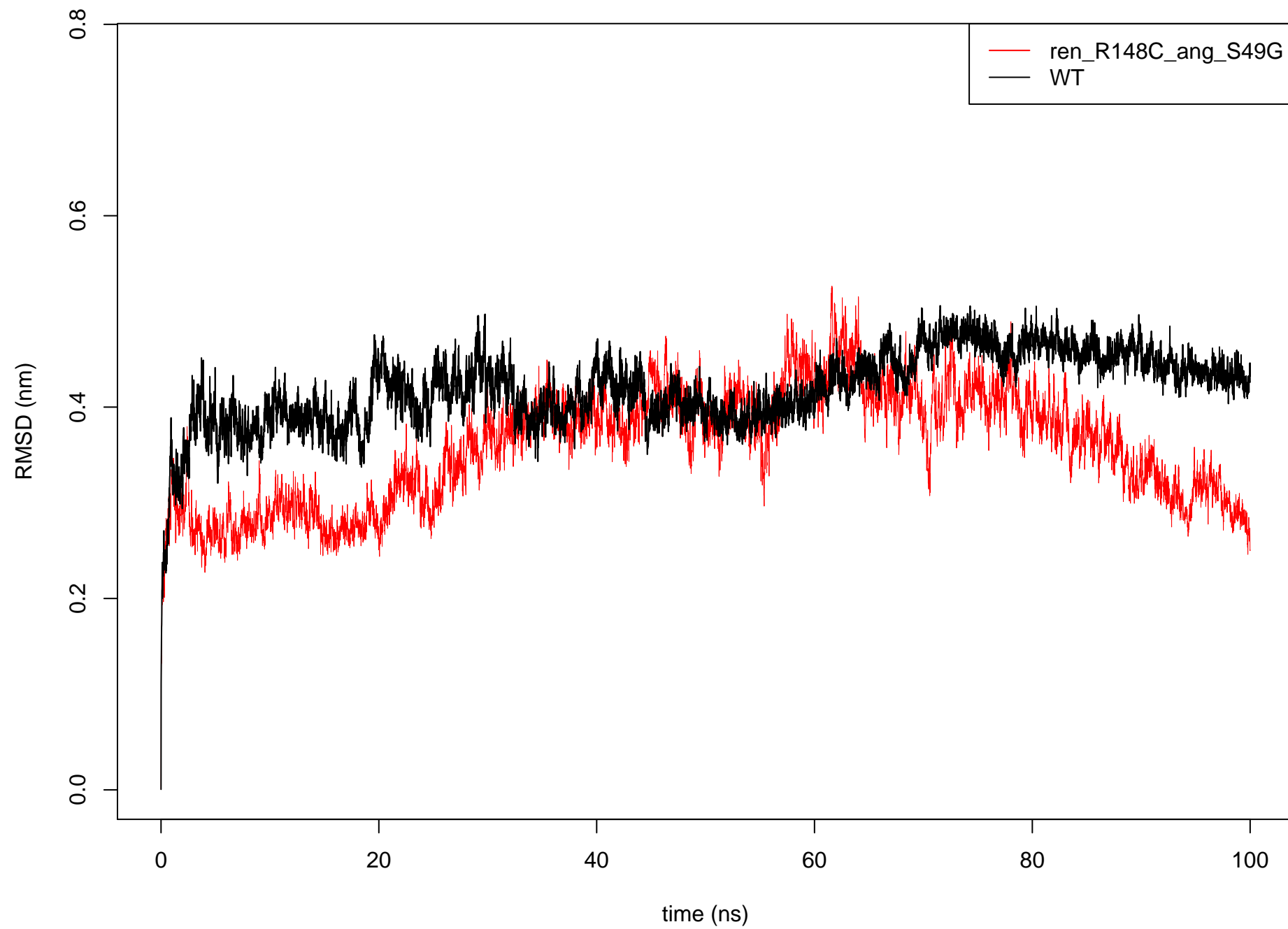
C alpha RMSD: ren_R148C_ang_S49G vs WT
