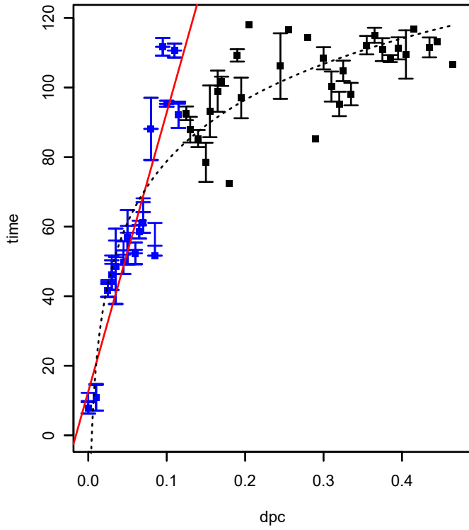
SPO3888 (COG1952) (*HTCC2255-Basal)
