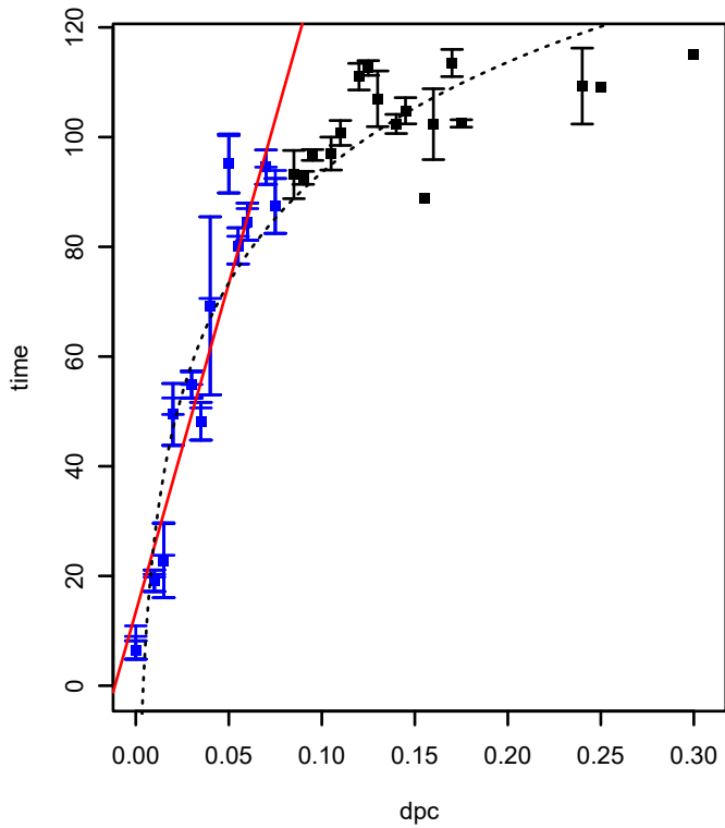
SPO0312 (COG0782) (*HTCC2255-Basal)
