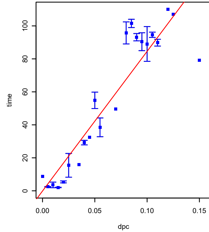
SPO3332 (COG0624) (*HTCC2255-Basal)
