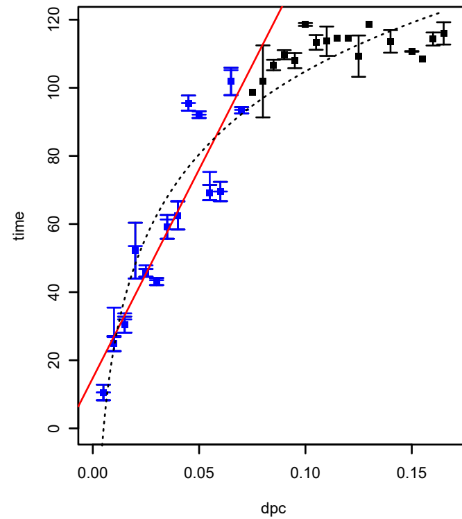
SPO0923 (COG0458) (*HTCC2255-Basal)
