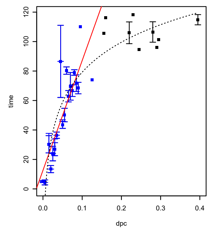
SPO2056 (COG0352) (*HTCC2255-Basal)
