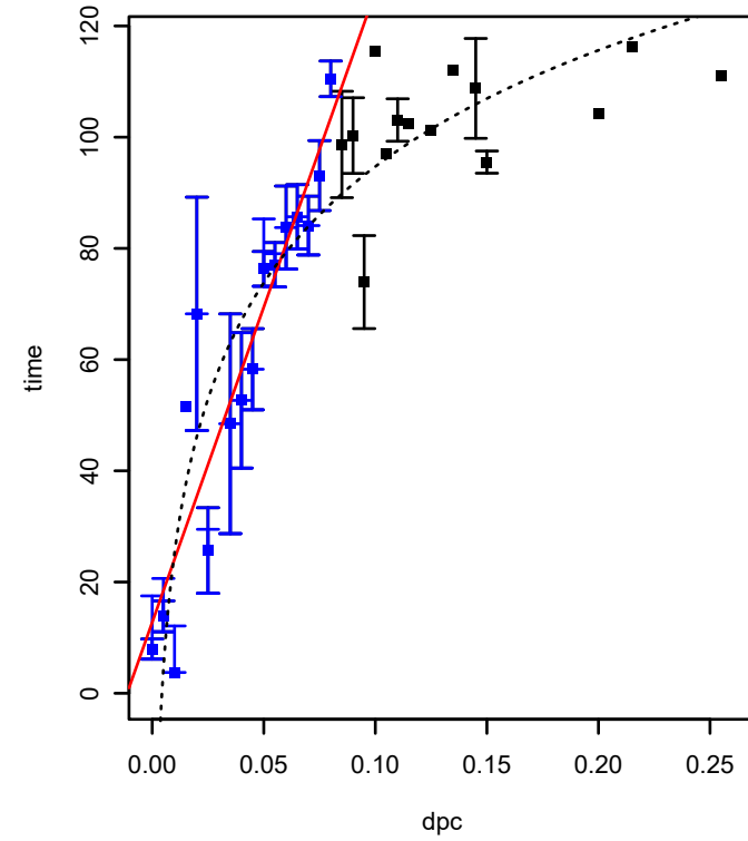
SPO0083 (COG0349) (*HTCC2255-Basal)
