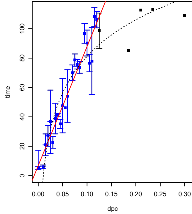
SPO0393 (COG0705) (*HTCC2255-Basal)
