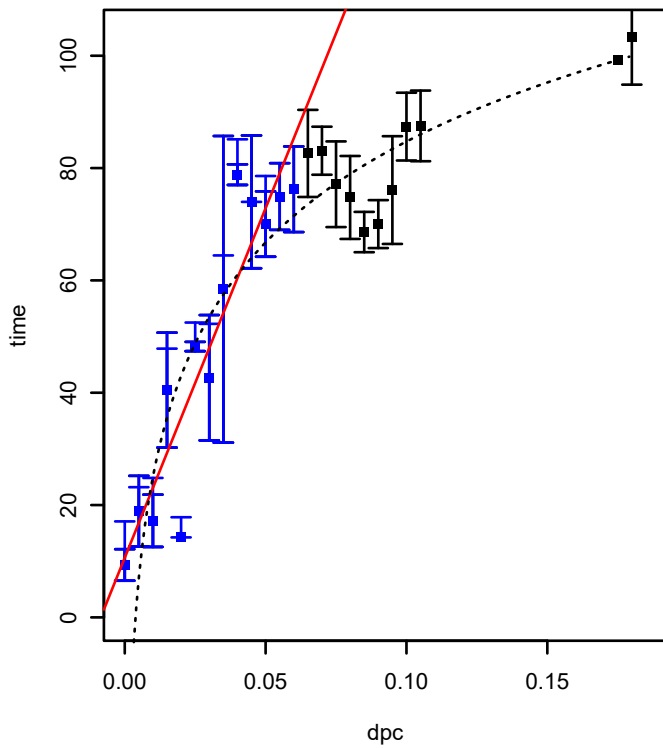
SPO2517 (COG4783) (*HTCC2255-Basal)
