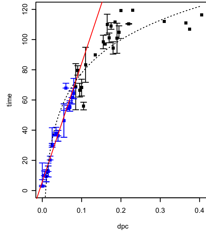
SPO3120 (COG2264) (*HTCC2255-Basal)
