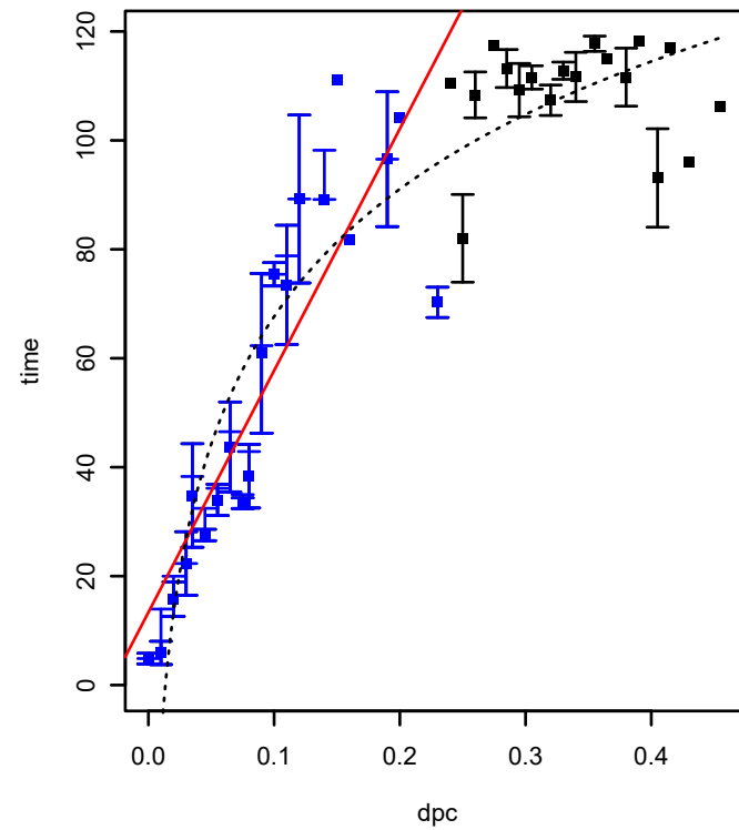
SPO2636 (COG3749) (*HTCC2255-Basal)
