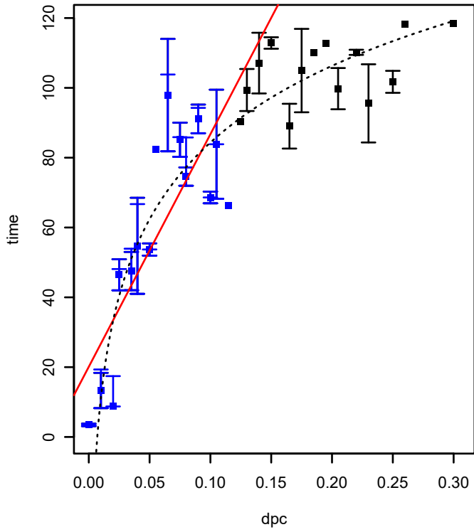
SPO2165 (COG2166) (*HTCC2255-Basal)
