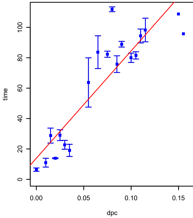
SPO1634 (COG0703) (*HTCC2255-Basal)
