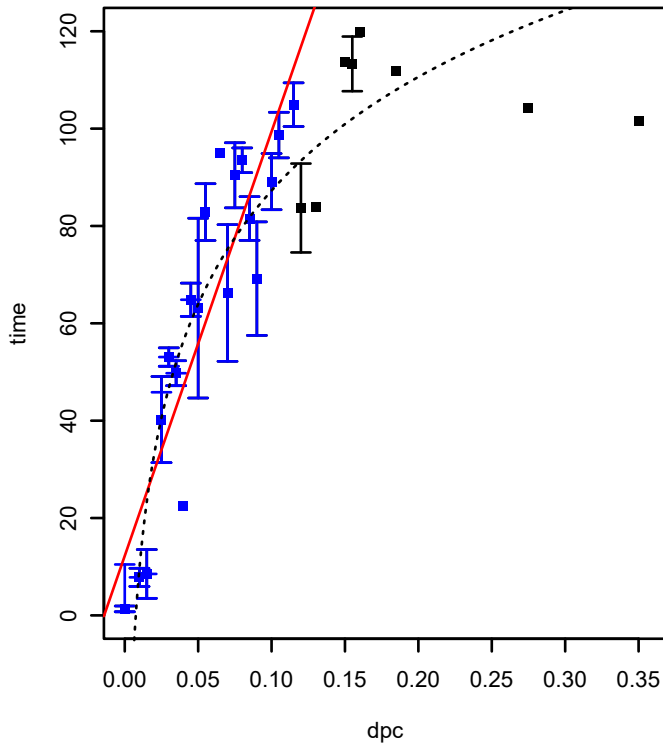
SPO0007 (COG0127) (*HTCC2255-Basal)
