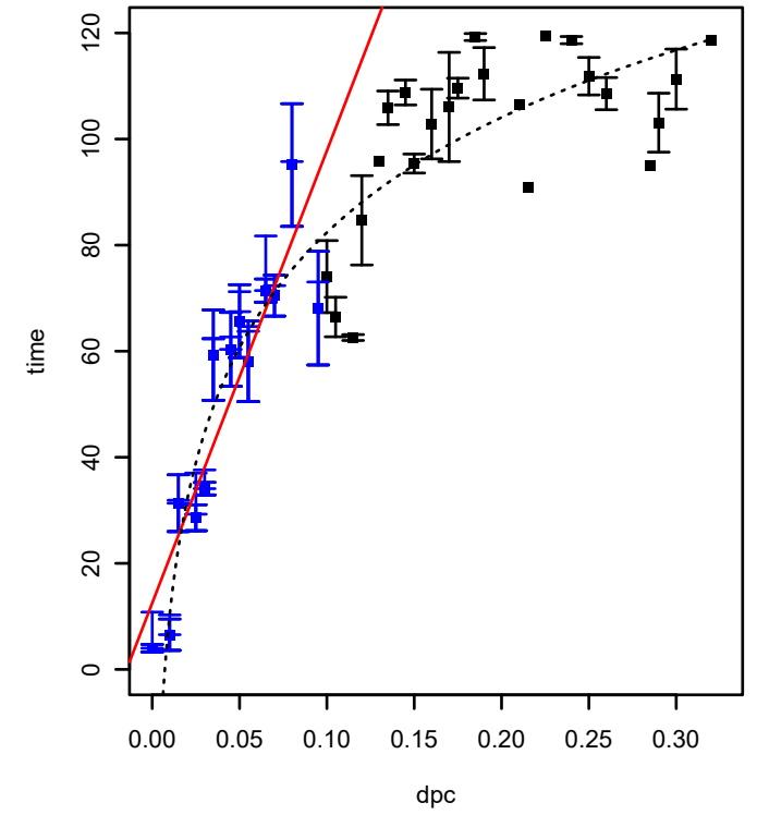
SPO1763 (COG0781) (*HTCC2255-Basal)
