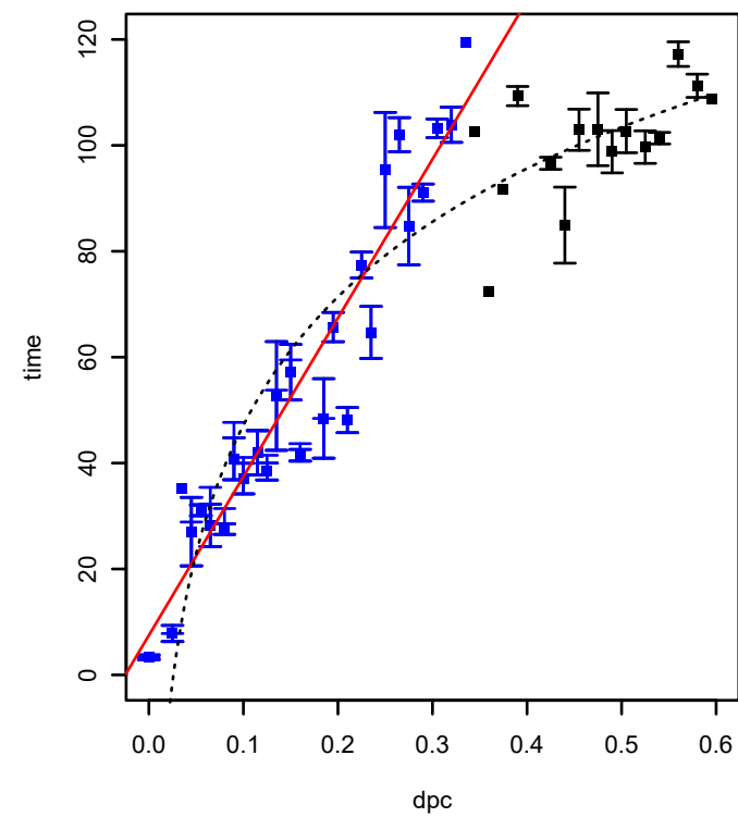
SPO3237 (COG5336) (*HTCC2255-Basal)
