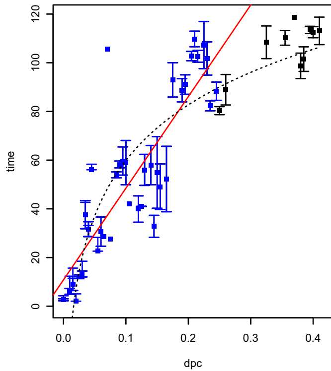
SPO3233 (COG0711) (*HTCC2255-Basal)
