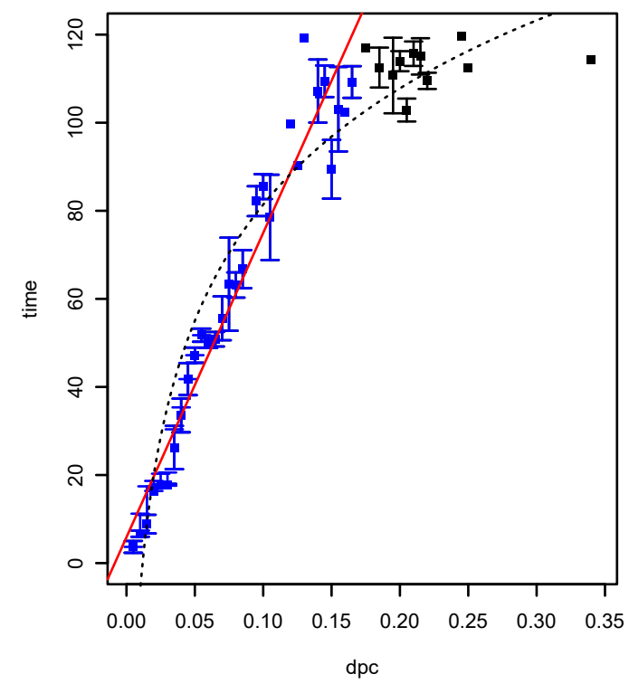
SPO0146 (COG0266) (*HTCC2255-Basal)
