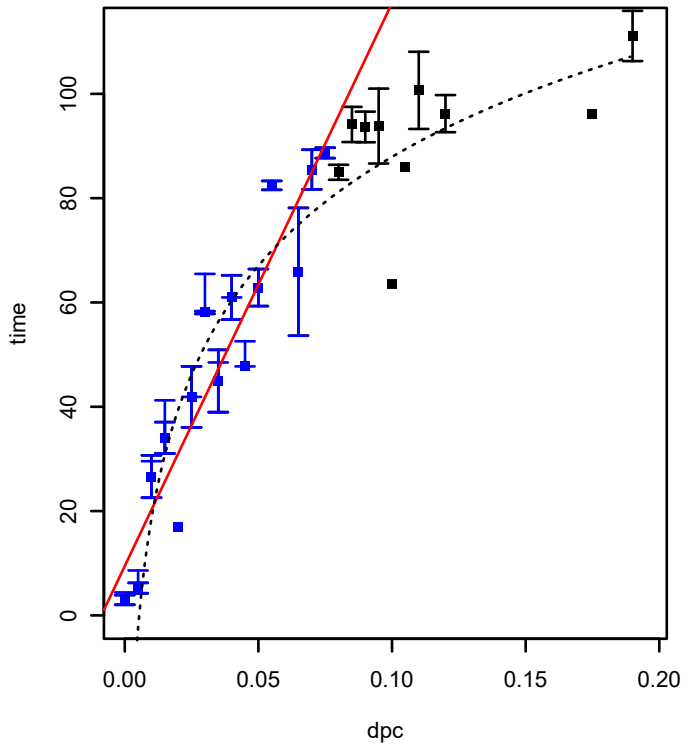
SPO0397 (COG2844) (*HTCC2255-Basal)
