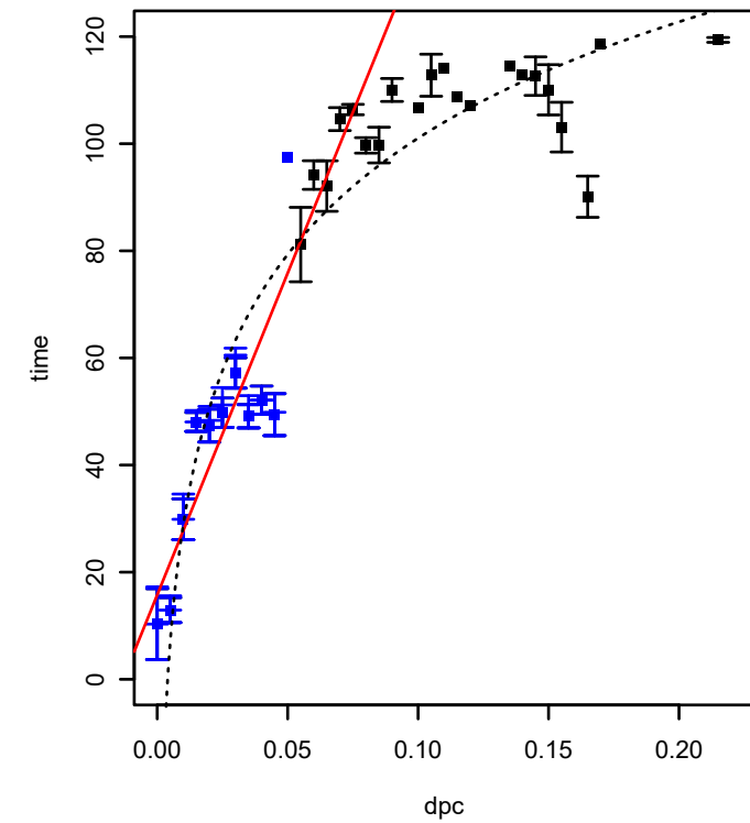
SPO2764 (COG1008) (*HTCC2255-Basal)
