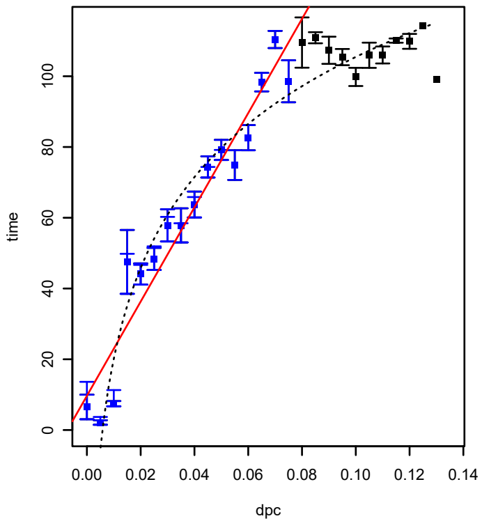
SPO0401 (COG0189) (*HTCC2255-Basal)
