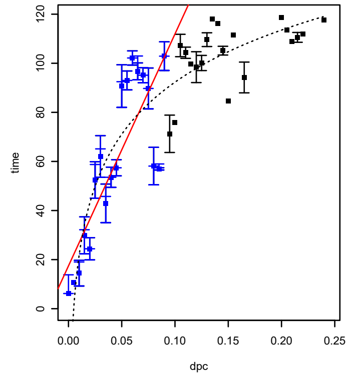
SPO2169 (COG0150) (*HTCC2255-Basal)
