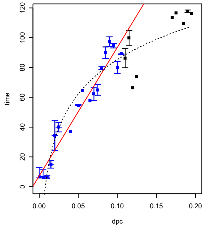
SPO2226 (COG0809) (*HTCC2255-Basal)
