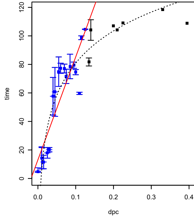
SPO3193 (COG5458) (*HTCC2255-Basal)
