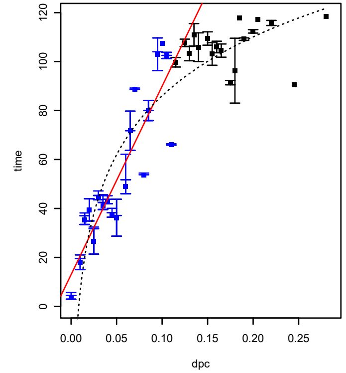
SPO0078 (COG1544) (*HTCC2255-Basal)
