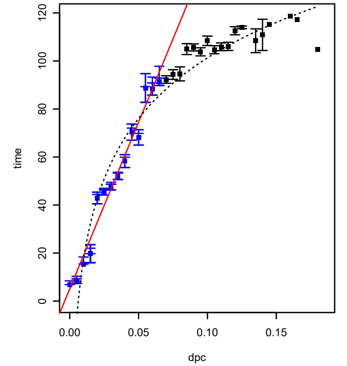
SPO0332 (COG0165) (*HTCC2255-Basal)
