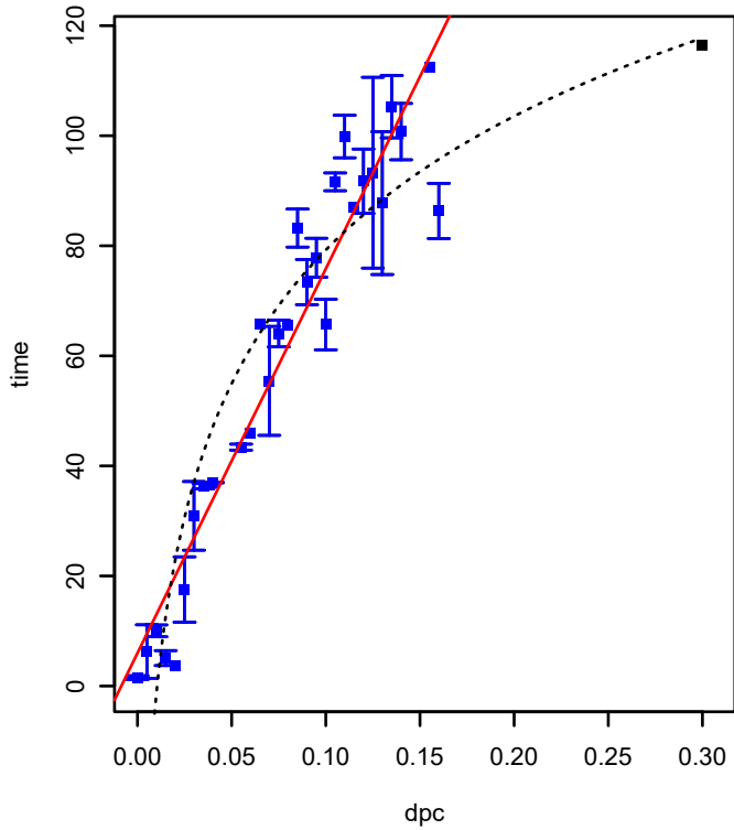
SPO0410 (COG0476) (*HTCC2255-Basal)
