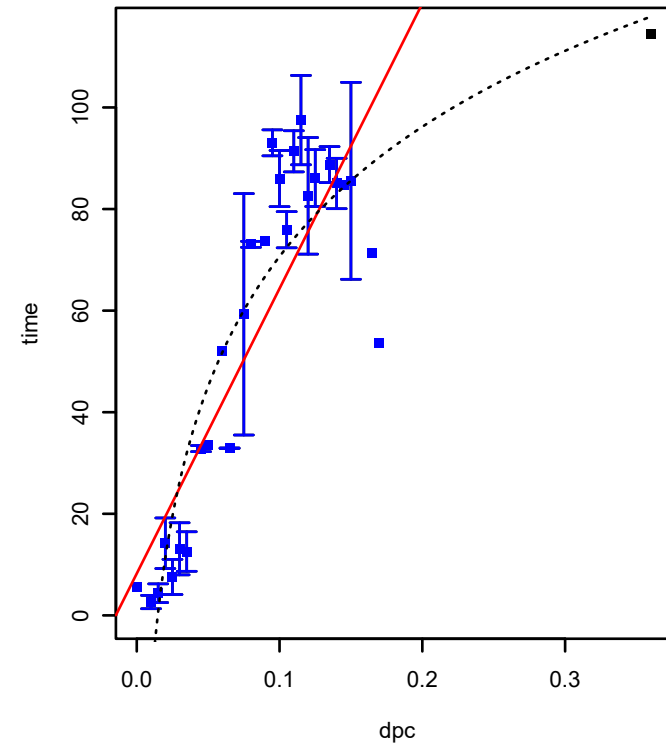
SPO3892 (COG0424) (*HTCC2255-Basal)
