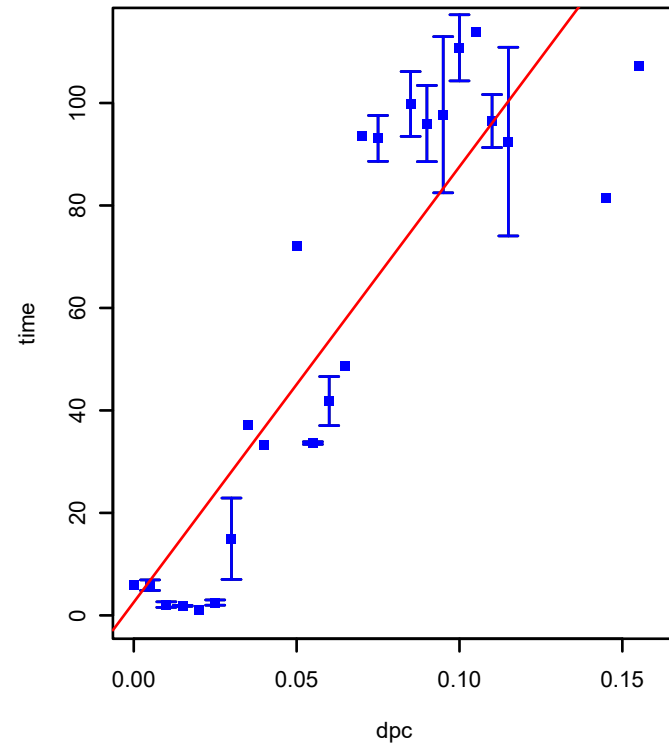
SPO0059 (COG1364) (*HTCC2255-Basal)
