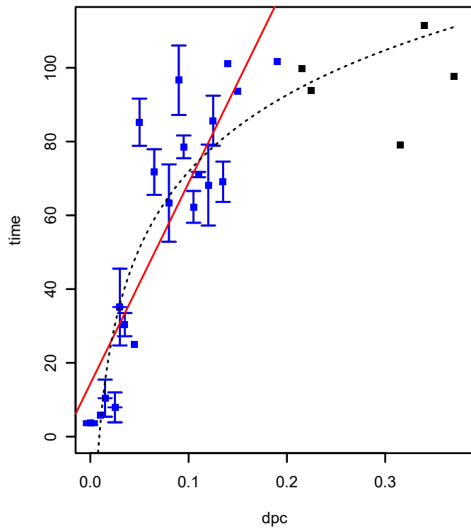
SPO3373 (COG0597) (*HTCC2255-Basal)
