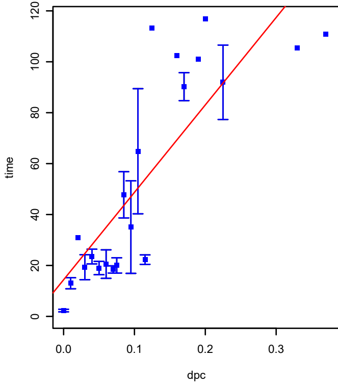
SPO0912 (COG0073) (*HTCC2255-Basal)
