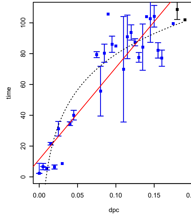
SPO3855 (COG0240) (*HTCC2255-Basal)
