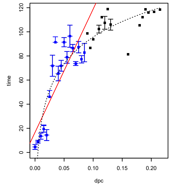
SPO0073 (COG0276) (*HTCC2255-Basal)
