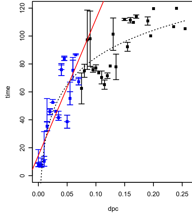
SPO2955 (COG2239) (*HTCC2255-Basal)
