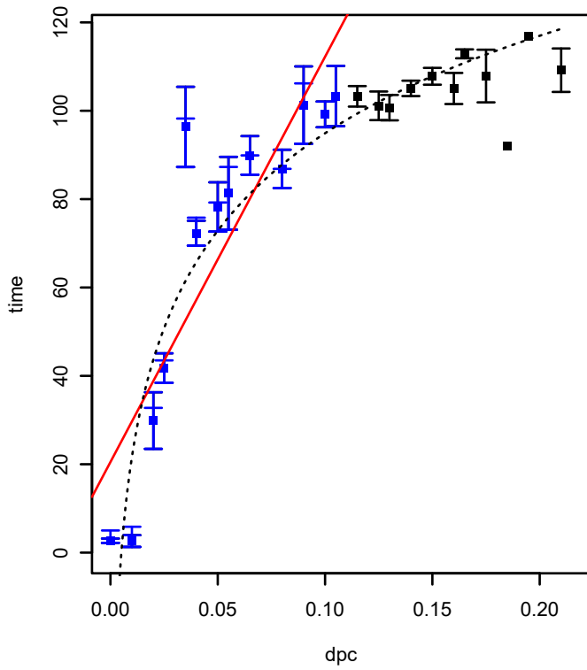
SPO0060 (COG1051) (*HTCC2255-Basal)
