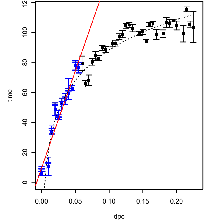
SPO2340 (COG0605) (*HTCC2255-Basal)
