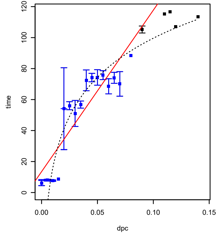
SPO0813 (COG1304) (*HTCC2255-Basal)
