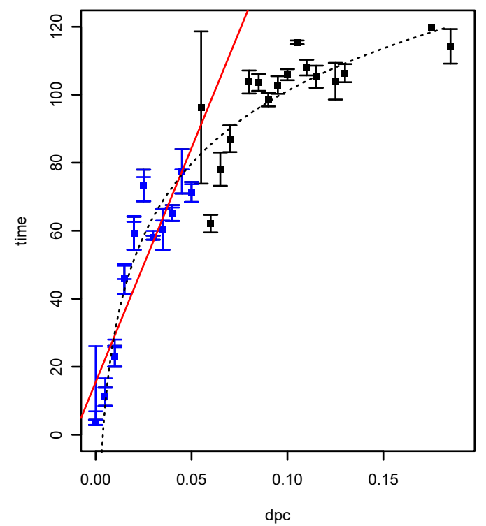
SPO1377 (COG0505) (*HTCC2255-Basal)
