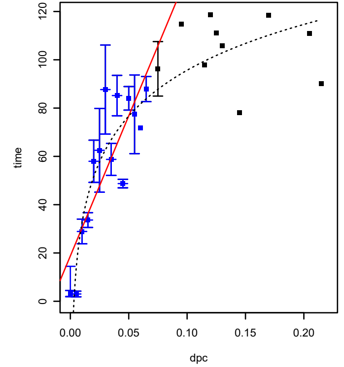
SPO3278 (COG0284) (*HTCC2255-Basal)
