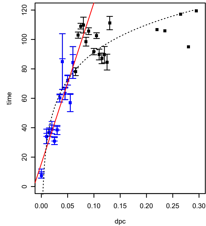
SPO2767 (COG0839) (*HTCC2255-Basal)
