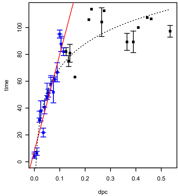
SPO1688 (COG2050) (*HTCC2255-Basal)
