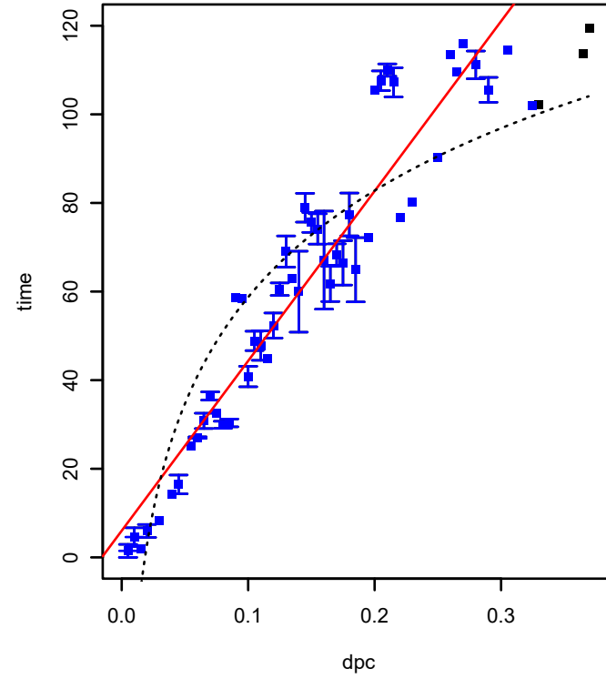
SPO0907 (COG1565) (*HTCC2255-Basal)
