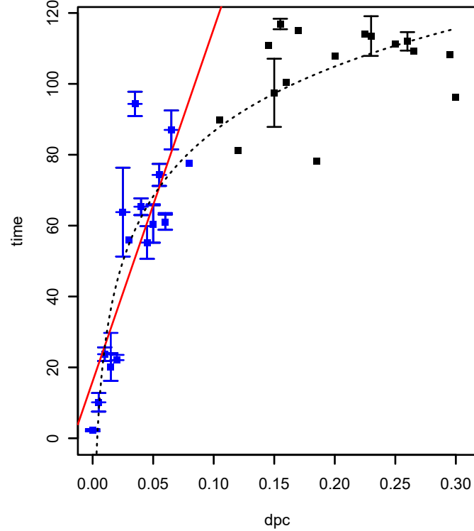
SPO0669 (COG0040) (*HTCC2255-Basal)
