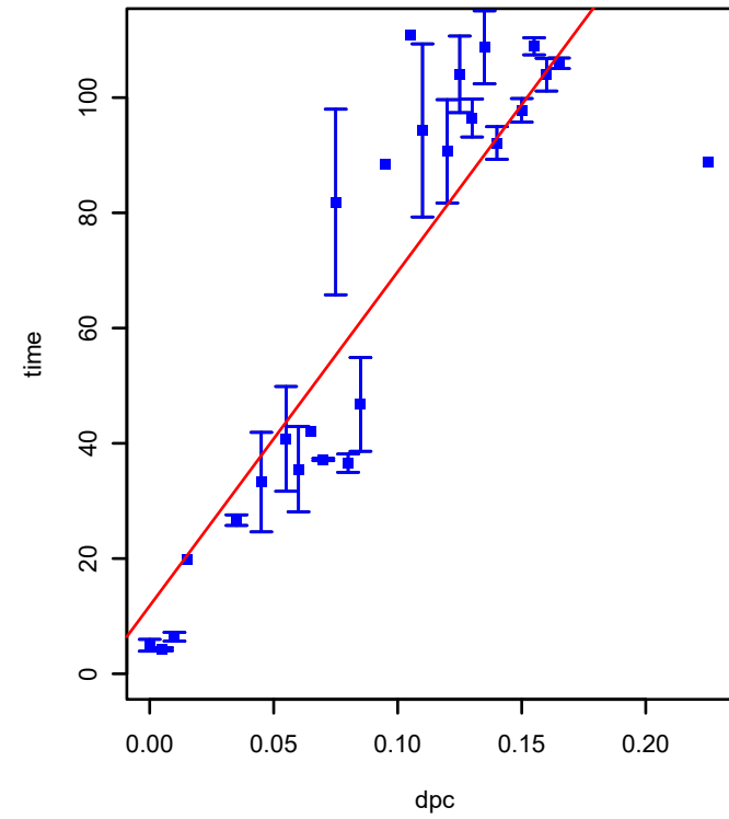
SPO3282 (COG3741) (*HTCC2255-Basal)
