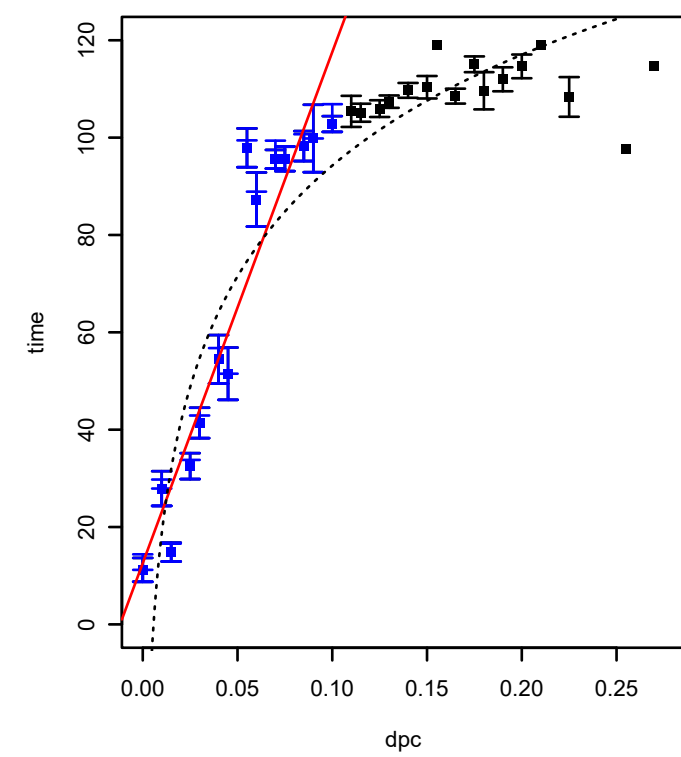
SPO2511 (COG1734) (*HTCC2255-Basal)
