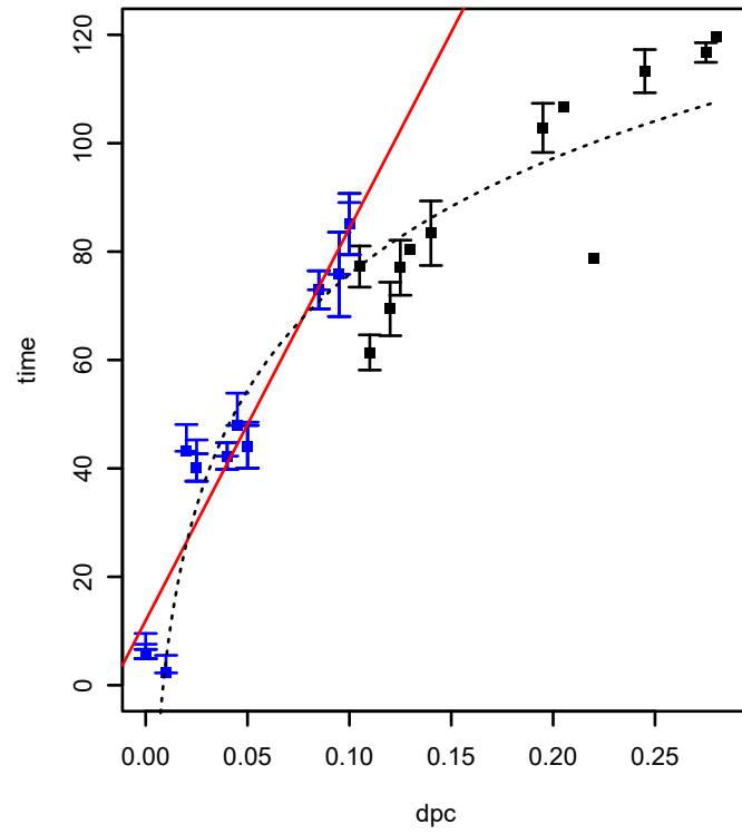
SPO1360 (COG3773) (*HTCC2255-Basal)
