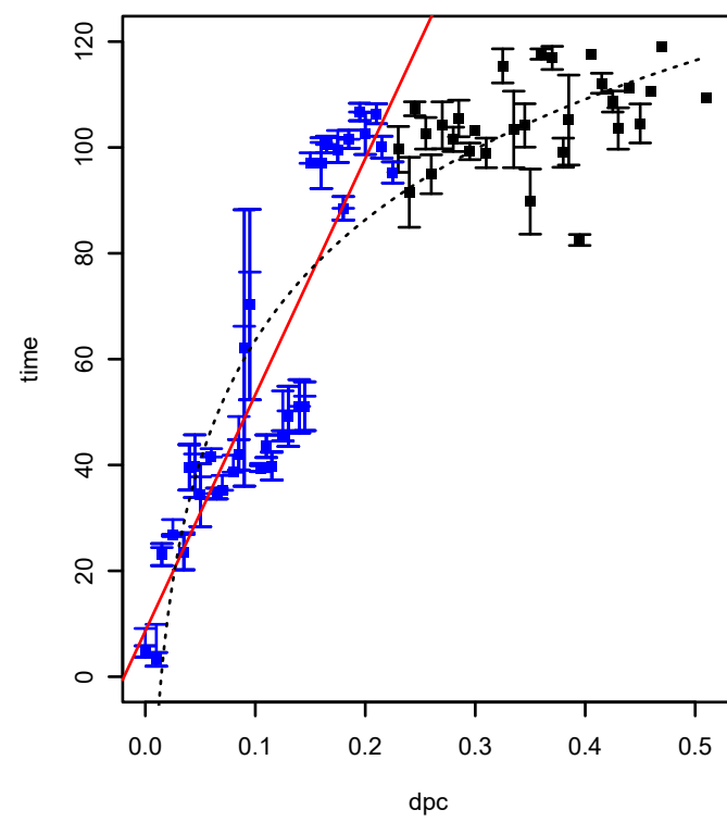
SPO0062 (COG2740) (*HTCC2255-Basal)
