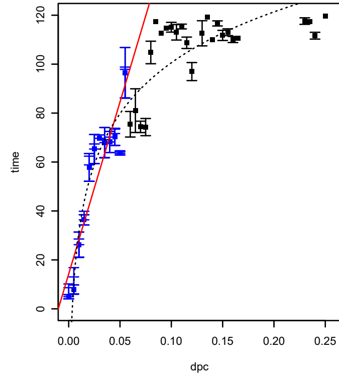
SPO2328 (COG1160) (*HTCC2255-Basal)
