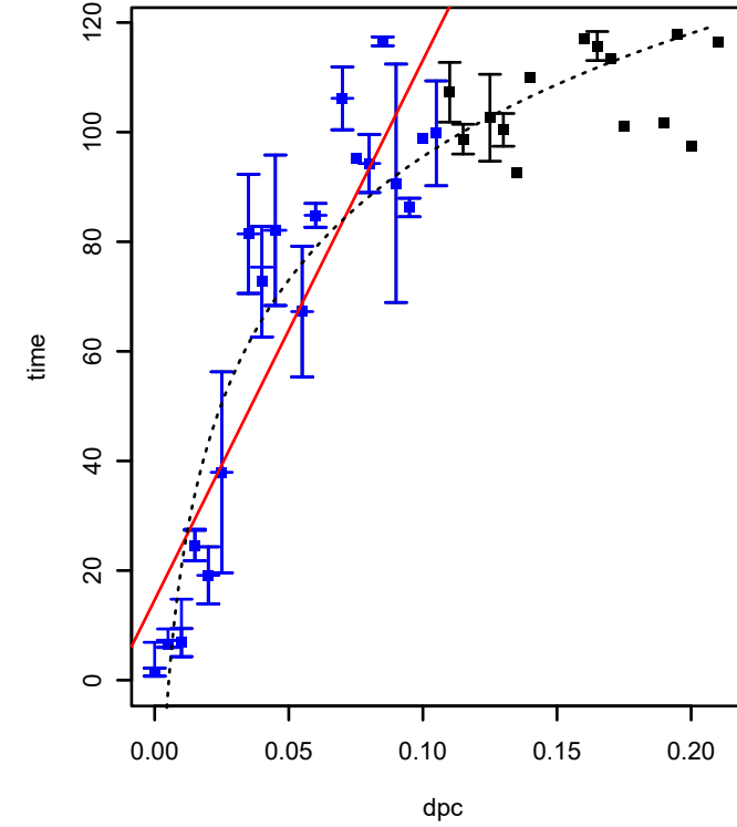
SPO3425 (COG0708) (*HTCC2255-Basal)
