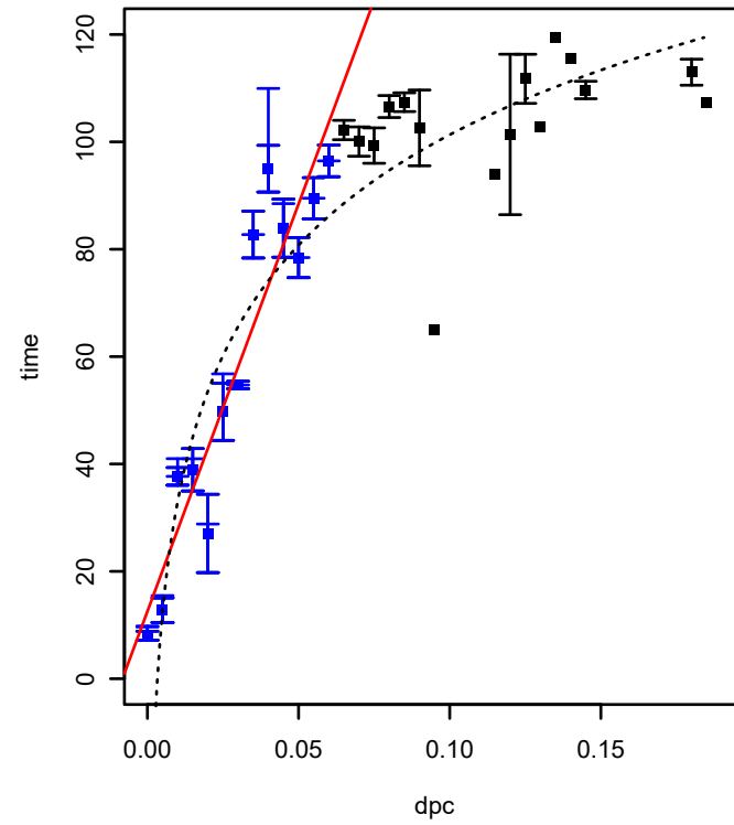
SPO2271 (COG0304) (*HTCC2255-Basal)
