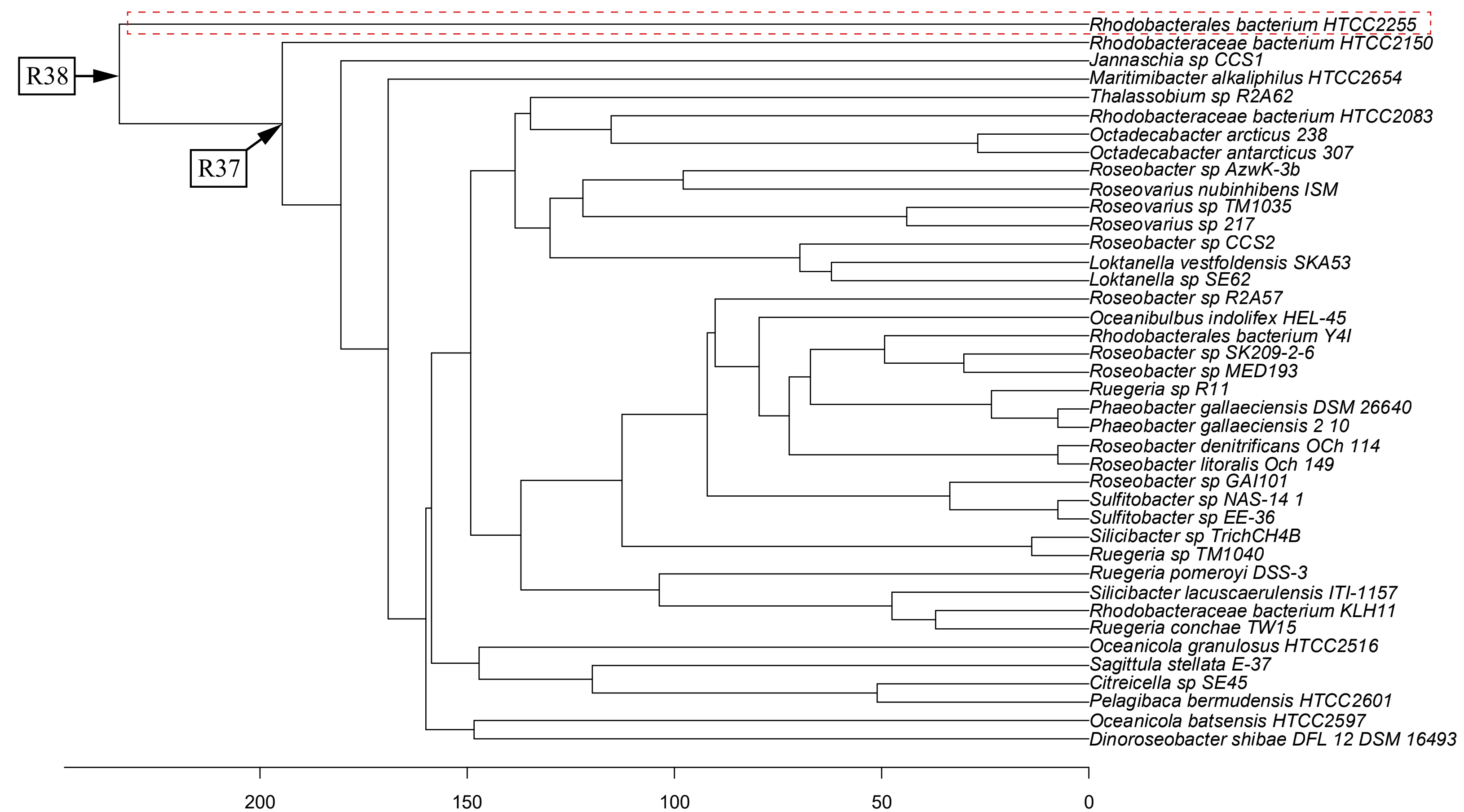
(A) SPO3237 (COG5336)
