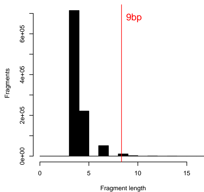
H) N = 1e+06
