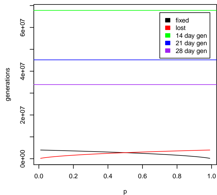
H) N = 1e+06
