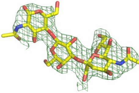
2Fo-Fc map
