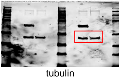
VPS35
