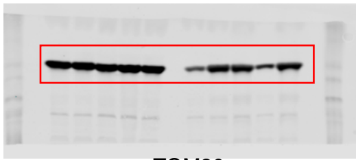
TOM20
