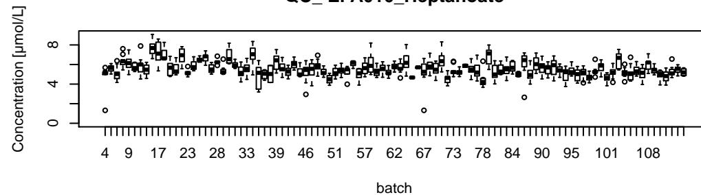
QC_EPA016_Heptanoate
