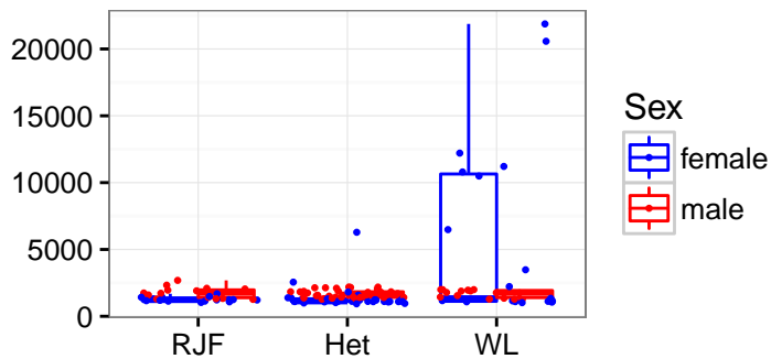
ENSGALT00000000548_LOXL2
