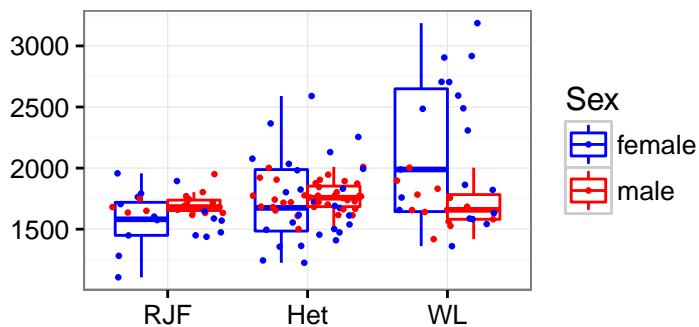
ENSGALT00000006851_ENSGALG000000004299
