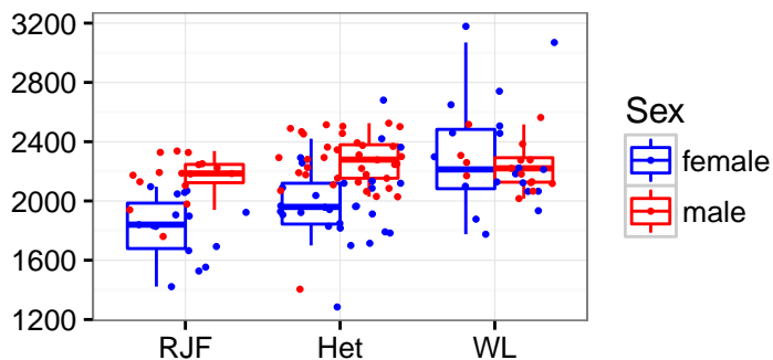
ENSGALT000000020835_CHPT1_CHICK
