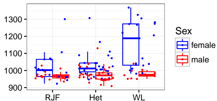
NM_204937_COCH
