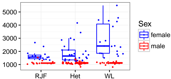
ENSGALT00000002921_UPK3B
