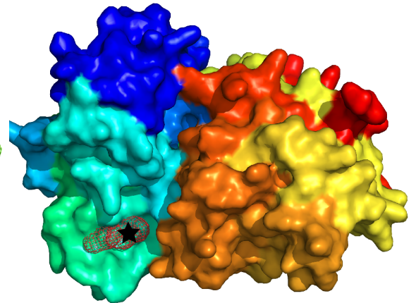
(d) Holo-LieIF trunc /MD
