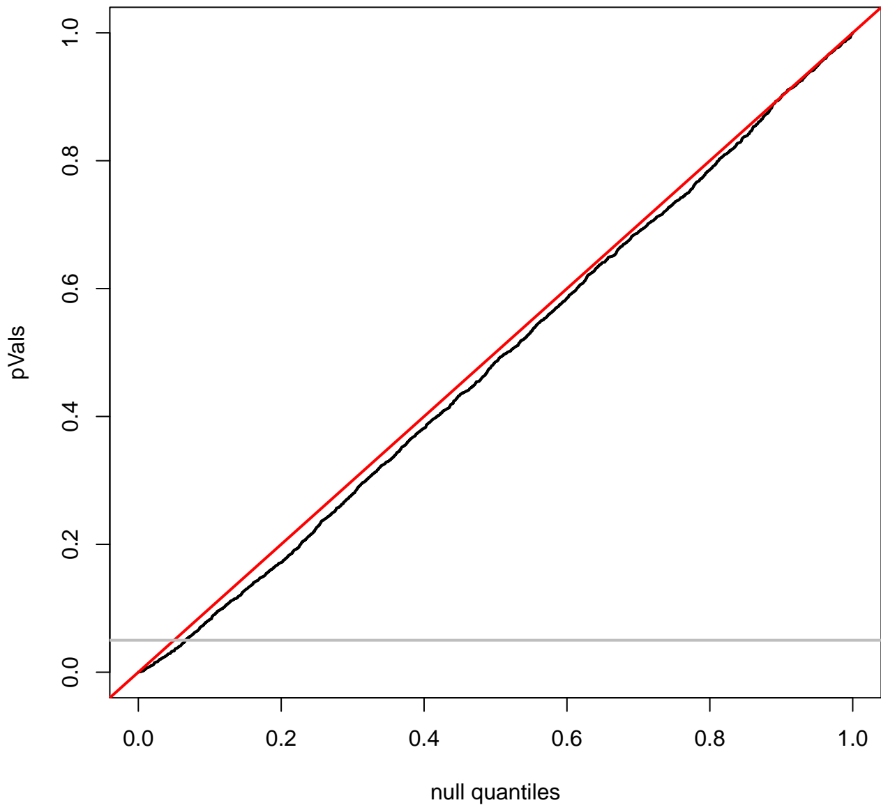
quantile plot for CESC
