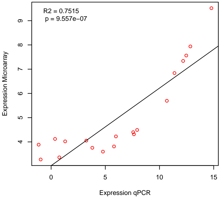
CYP24A1
