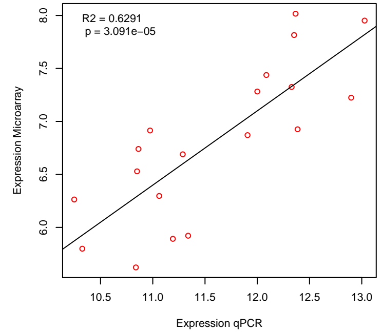
C1R
