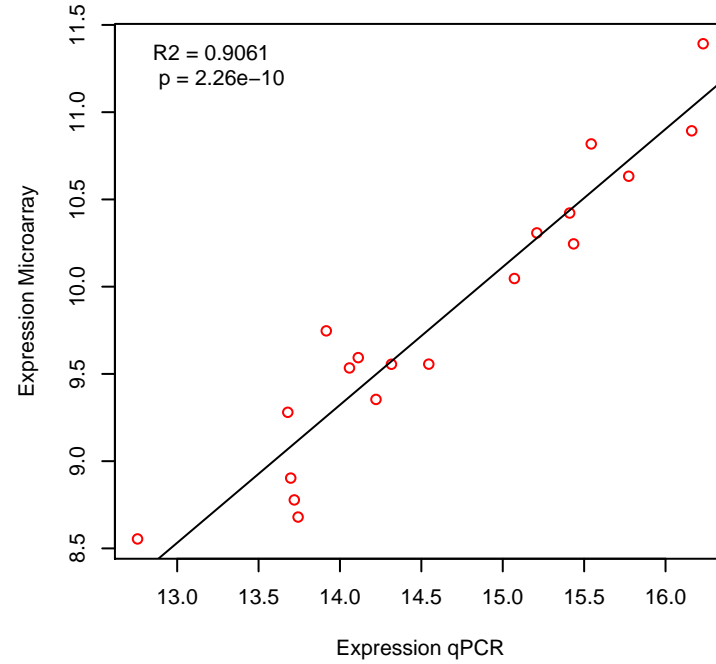
SPP1
