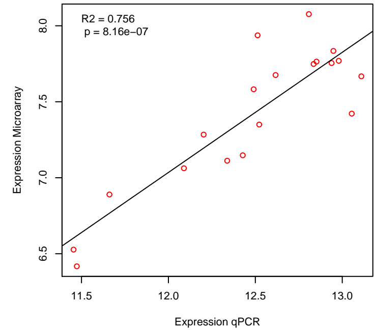
VDR
