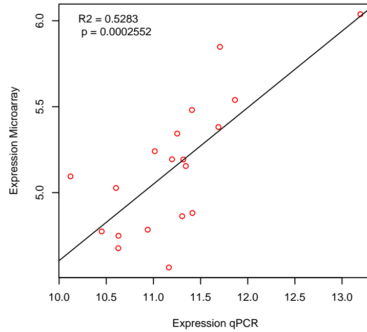
NFATC2
