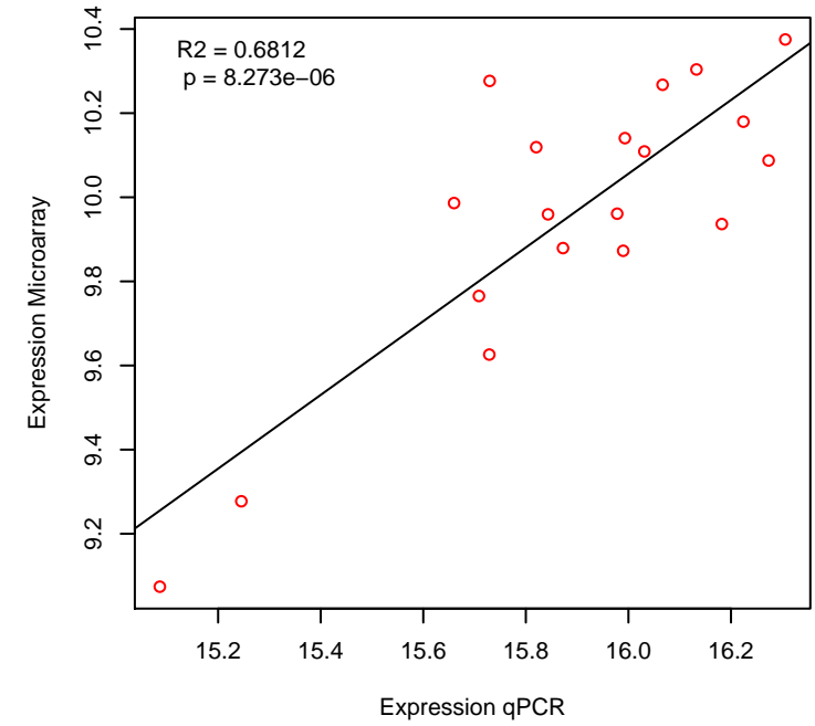
PTH1R
