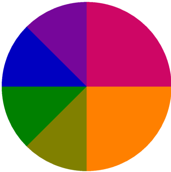
A. alabamensis (n=8)
