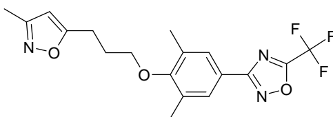
b) Pleconaril
