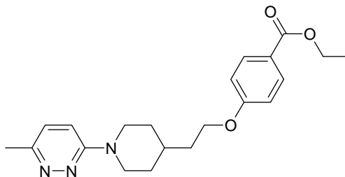
a) Pirodavir
