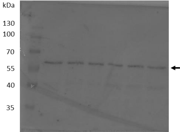
PKC \zeta
