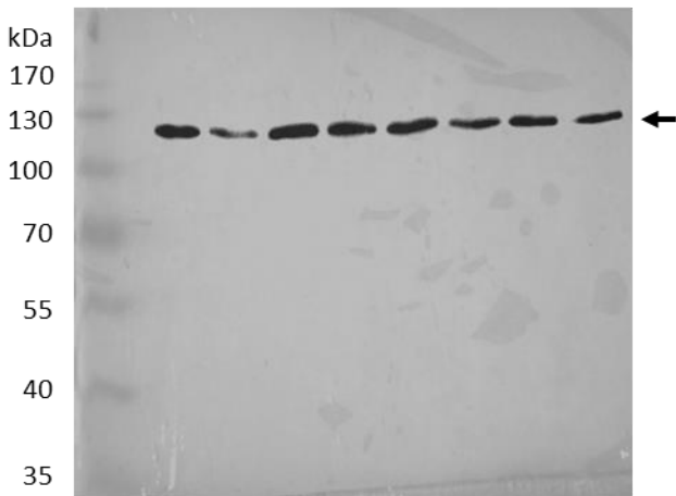
PKD1
