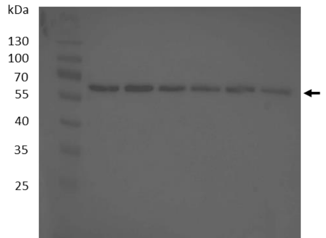
p-Akt Ser473
