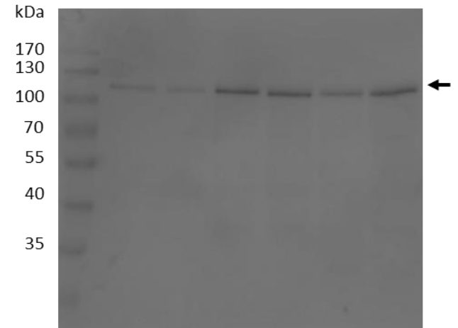
PKD2
