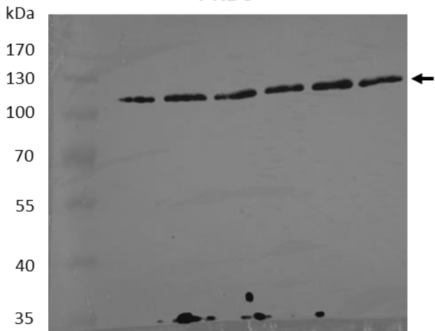
PKD3
