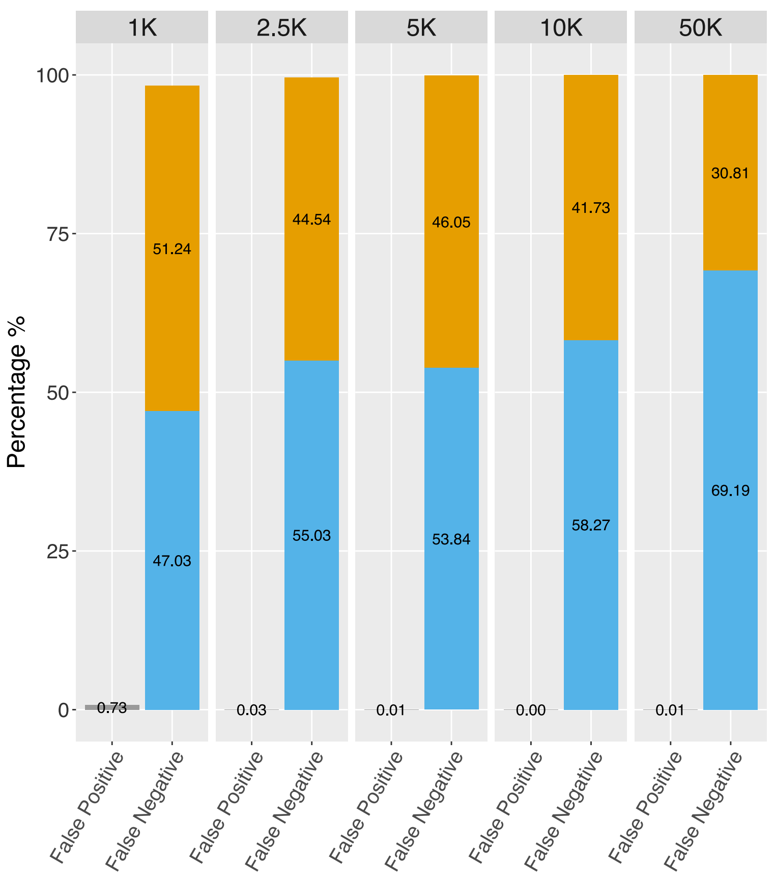
15% allelic error
