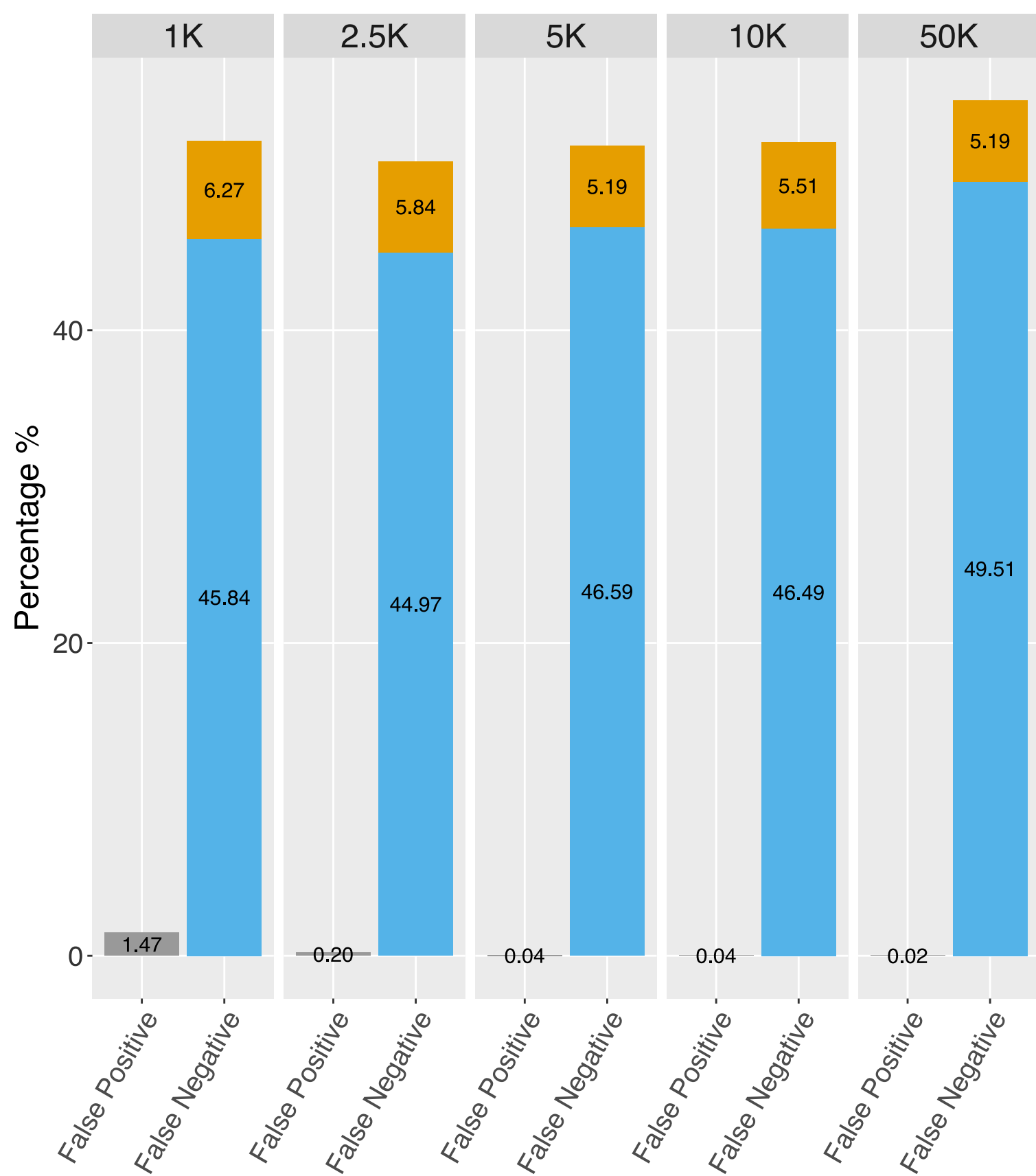
15% allelic error
