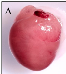
Wildtype
