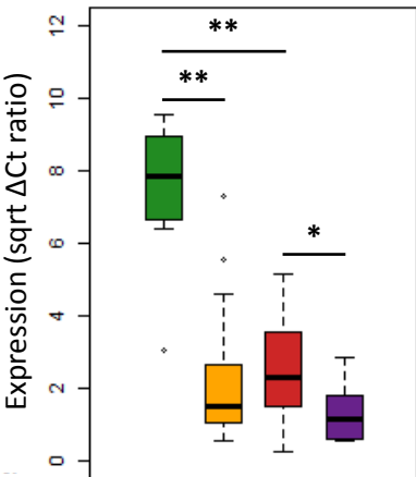
miR-203a-3p
