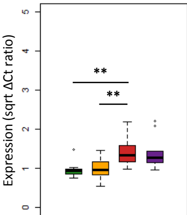
miR-15b-5p
