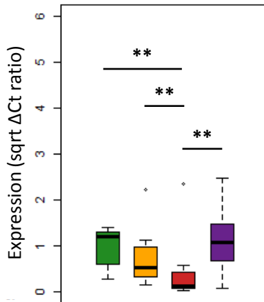
miR-375
