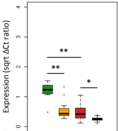
miR-149-5p
