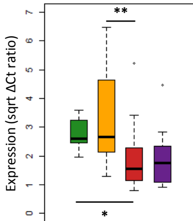
miR-125b-5p
