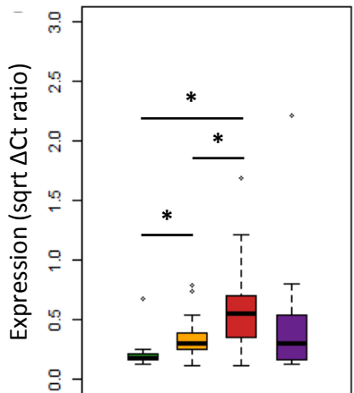
miR-9-5p
