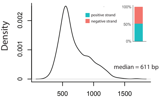
All genes (n=904)
