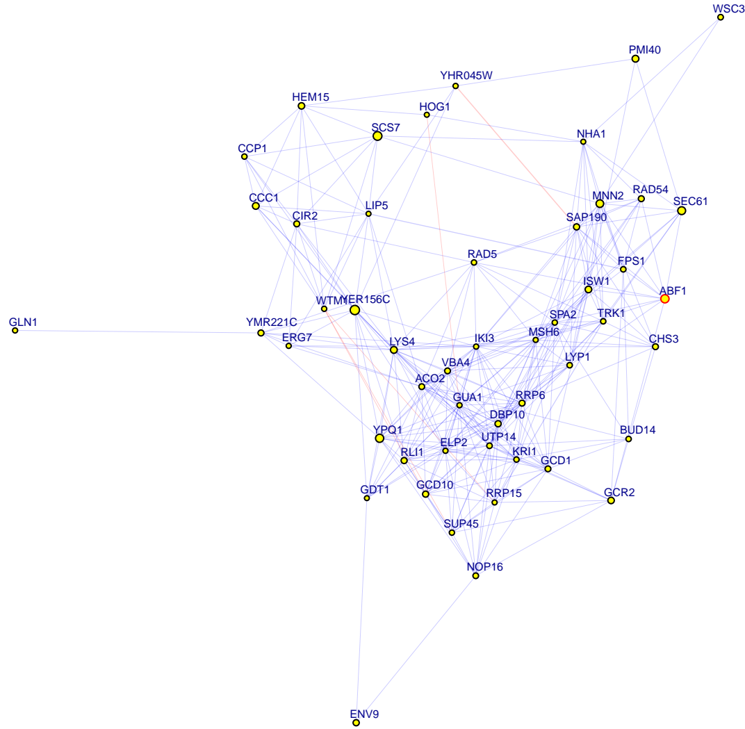
chrXI:232667_A/T top 50 down genes
