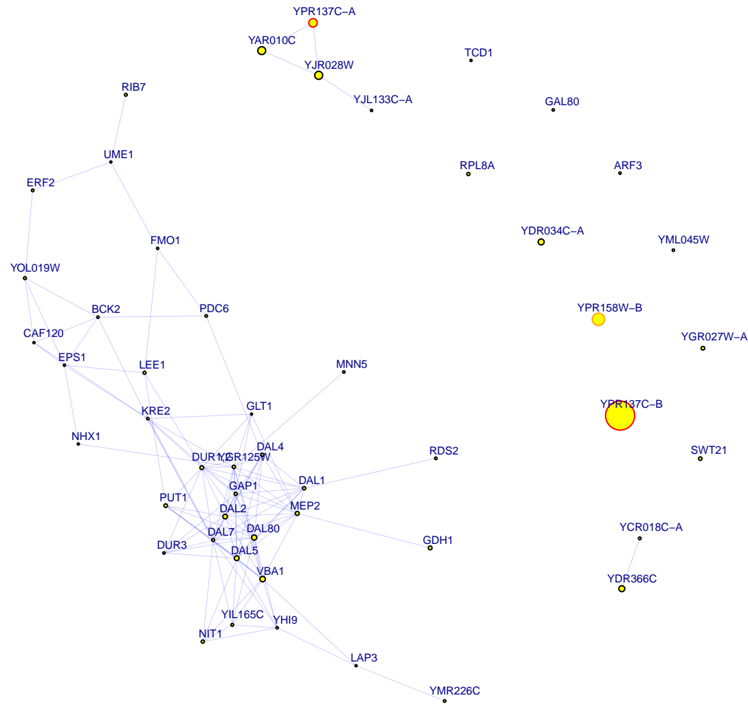
chrXVI:812990_T/C top 50 down genes
