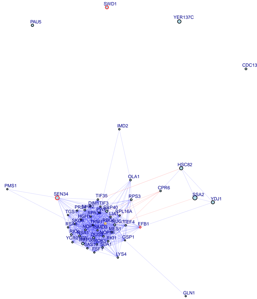
chr1:159467_G/A top 50 up genes
