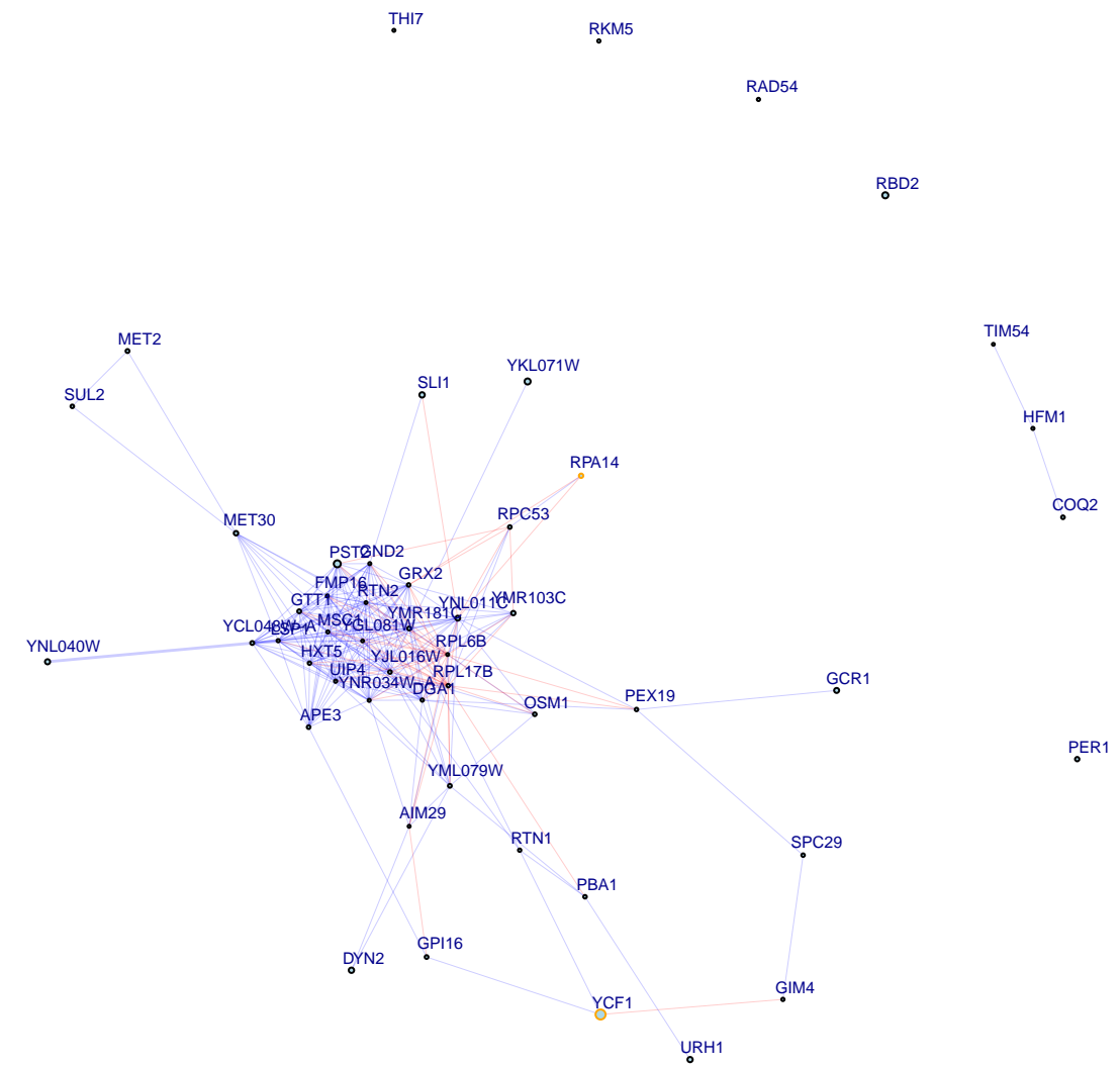
chrIV:745766_G/A top 50 up genes
