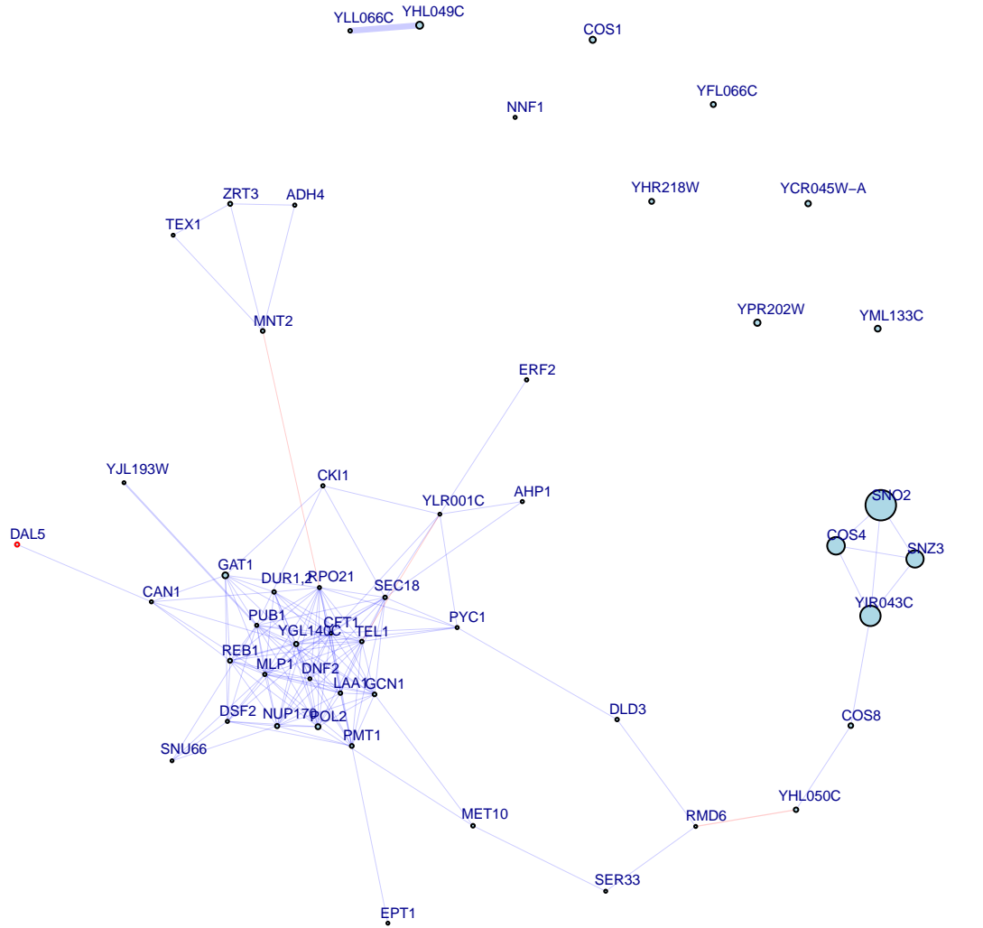
chrX:722130_T/C top 50 up genes
