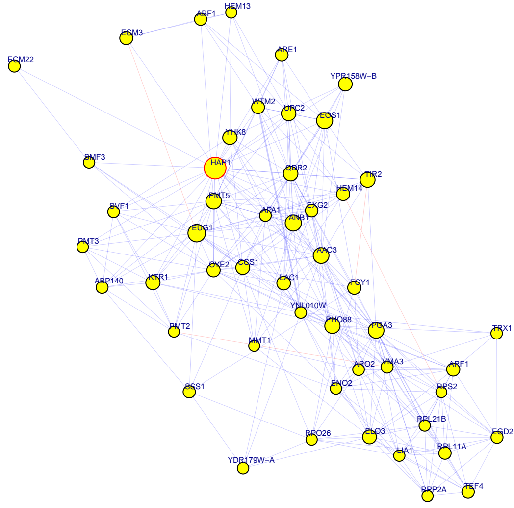
chrXII:657022_T/C top 50 down genes
