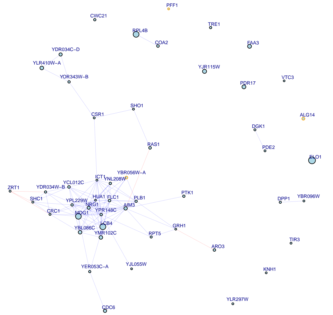
chrII:370967_C/T top 50 up genes
