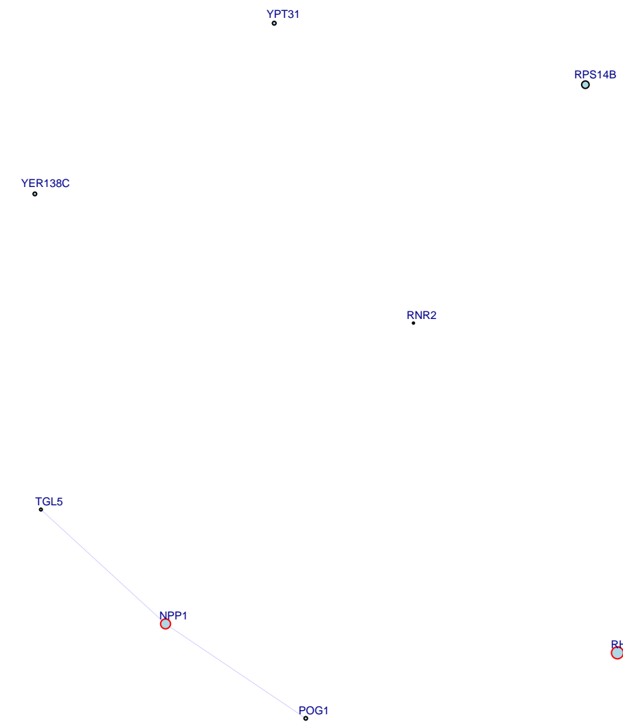
chrIII:166390_G/C top 9 up genes
