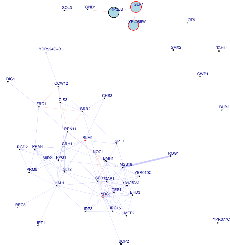
chrXVI:383928_G/A top 50 up genes
