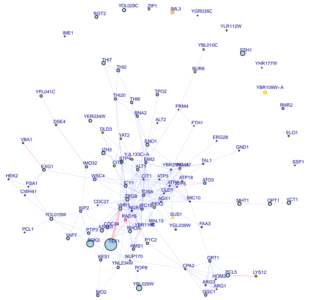
chrII:464478_G/A top 100 up and down genes
