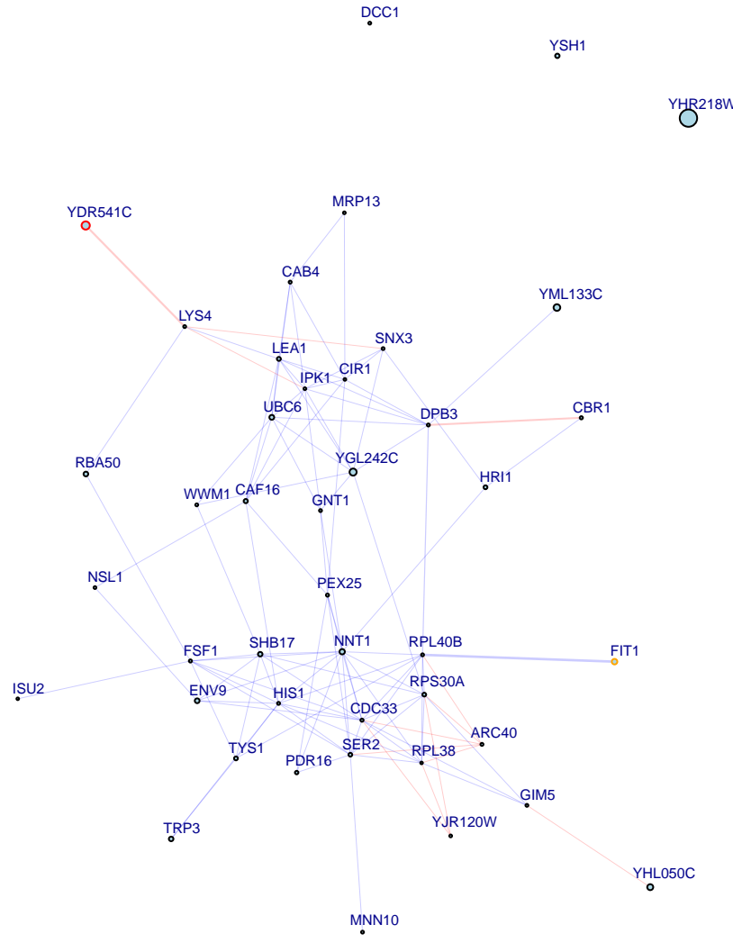
chrIV:1521369_A/C top 50 up genes
