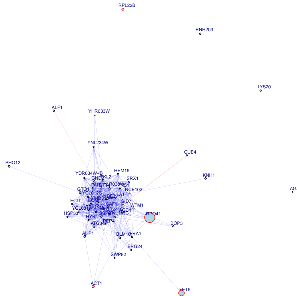
chrVI:71959_C/T top 50 up genes
