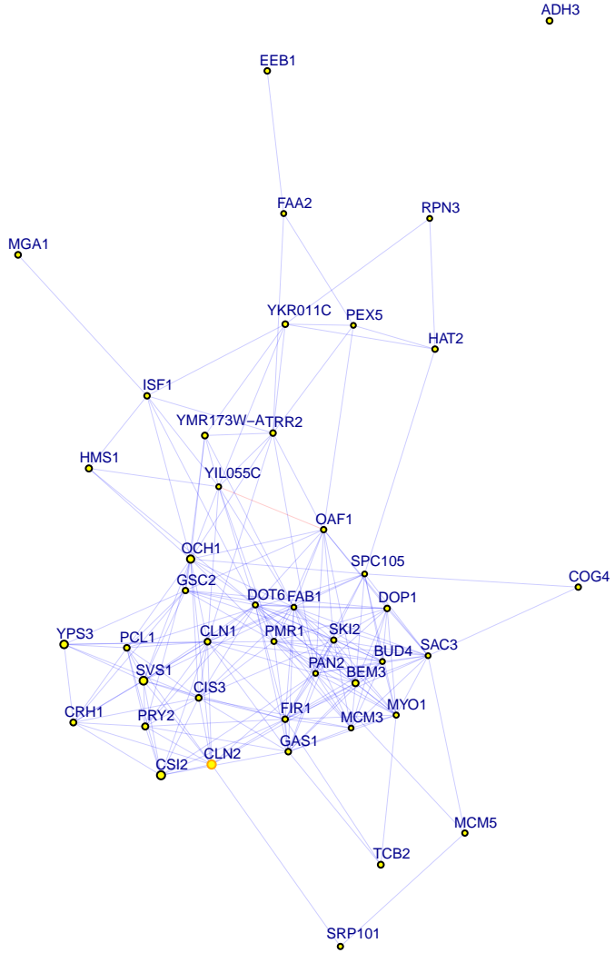
chrXVI:84945_G/A top 50 down genes
