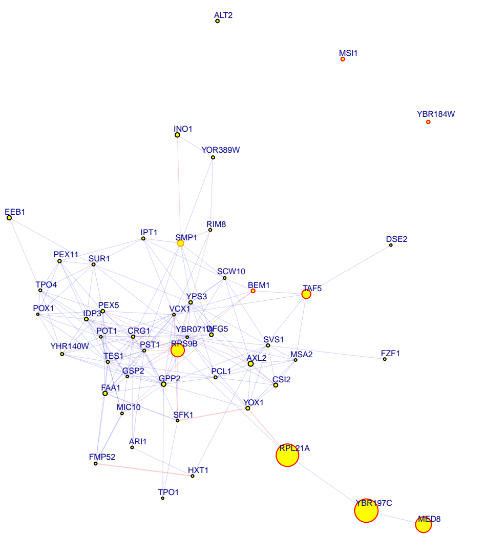
chrII:619028_C/A top 50 down genes
