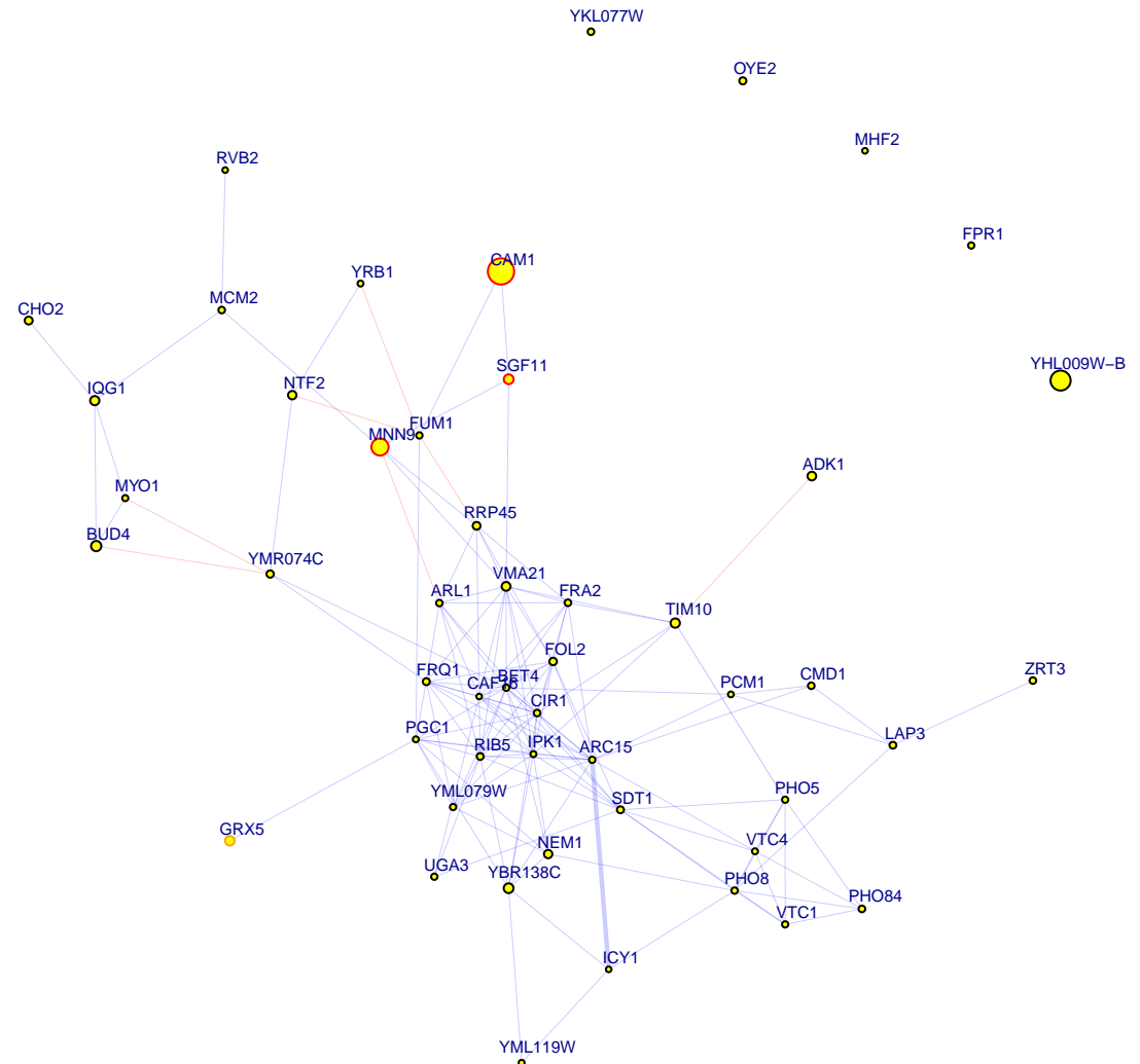
chrXVI:463543_G/A top 50 down genes
