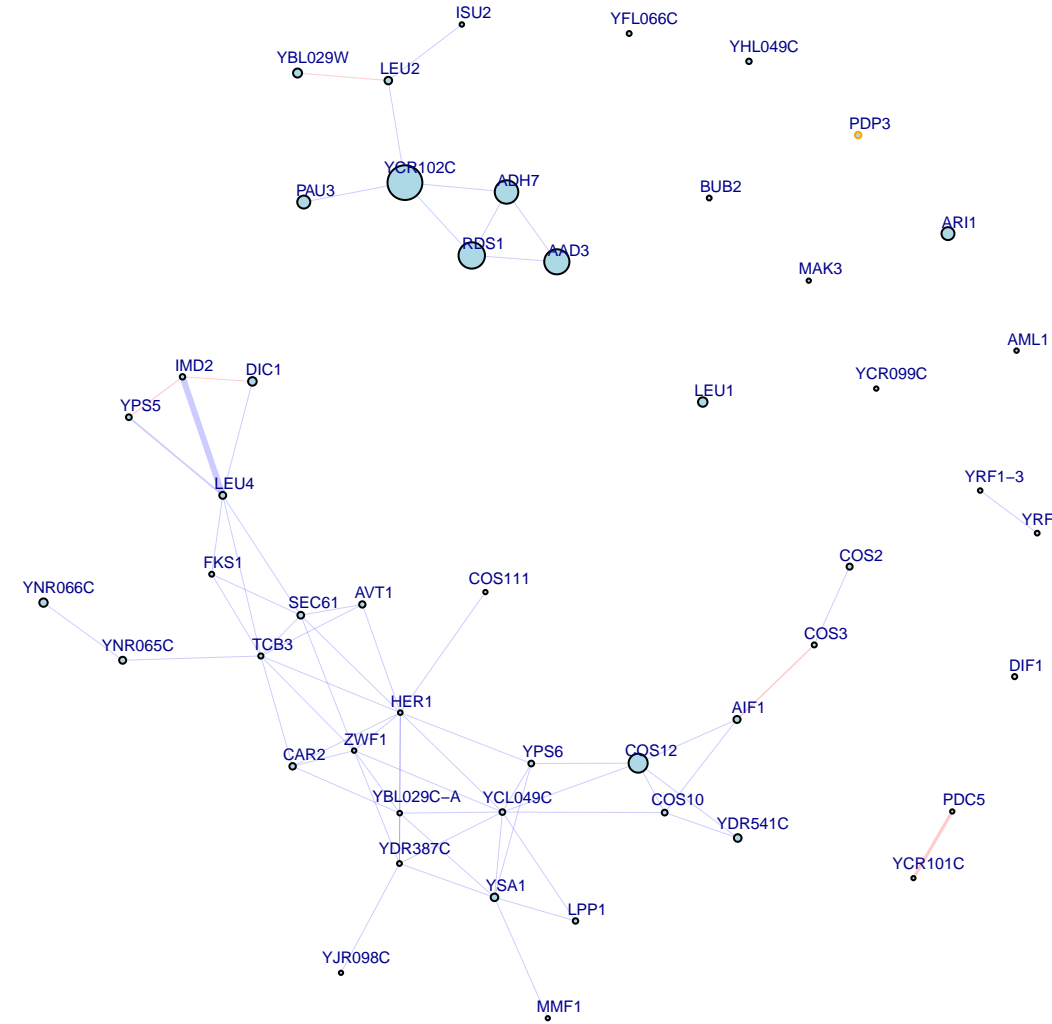
chrXII:1058607_C/T top 50 up genes
