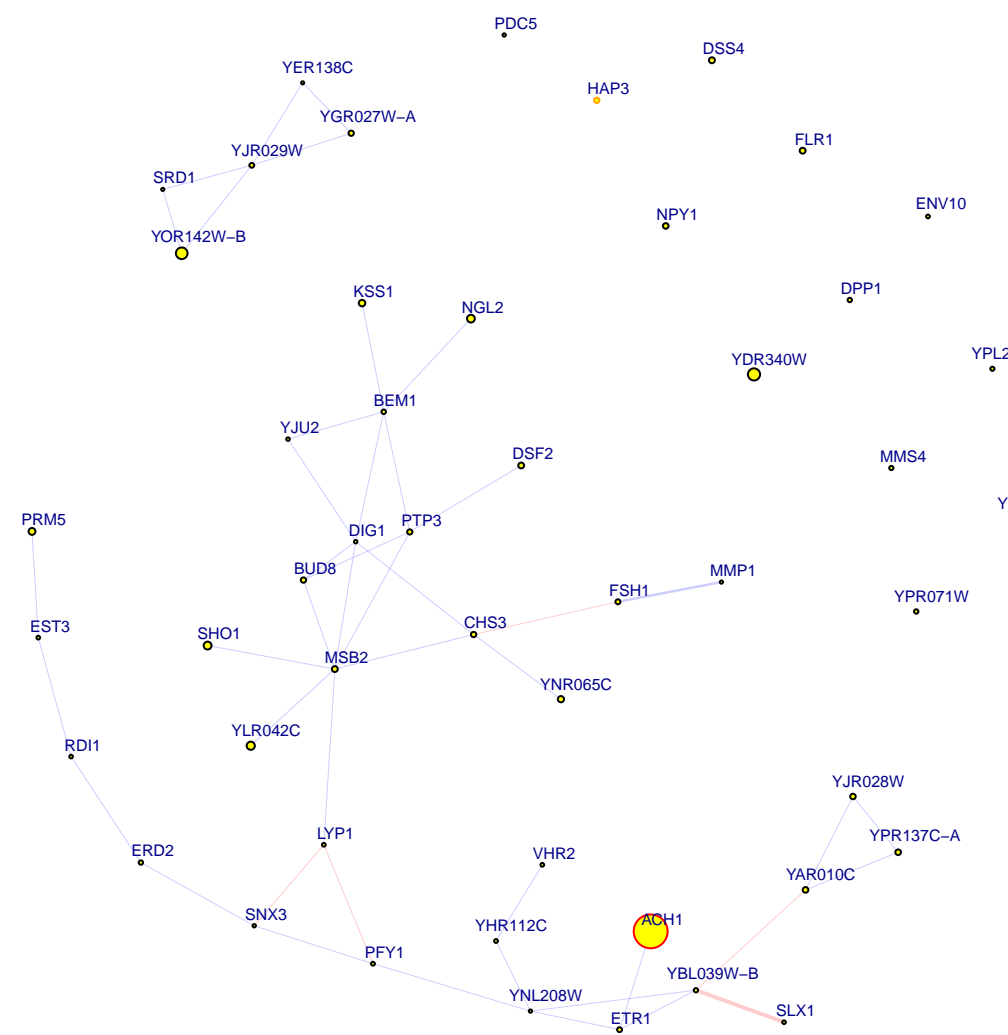
chrII:195177_T/A top 50 down genes
