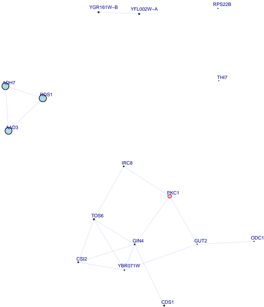
chrII:13061_G/T top 18 up genes
