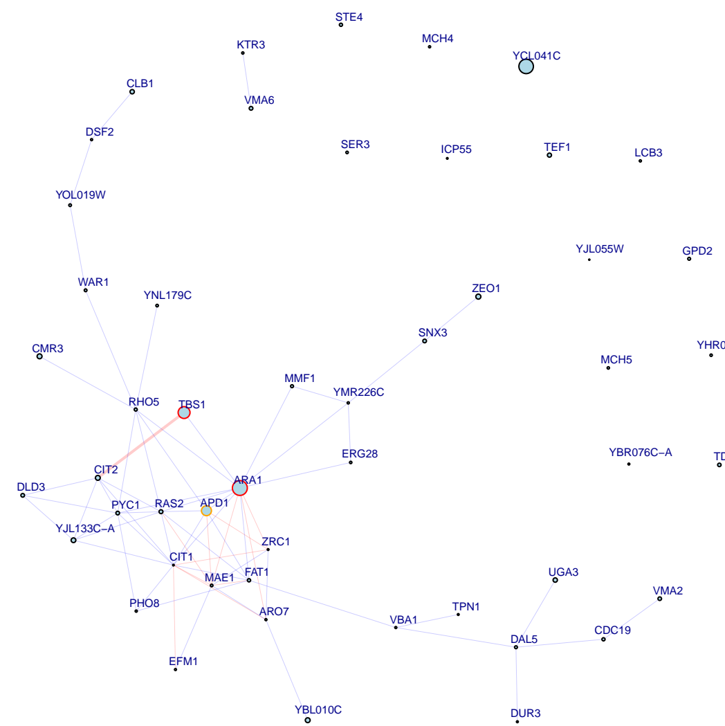
chrII:541139_G/A top 50 up genes
