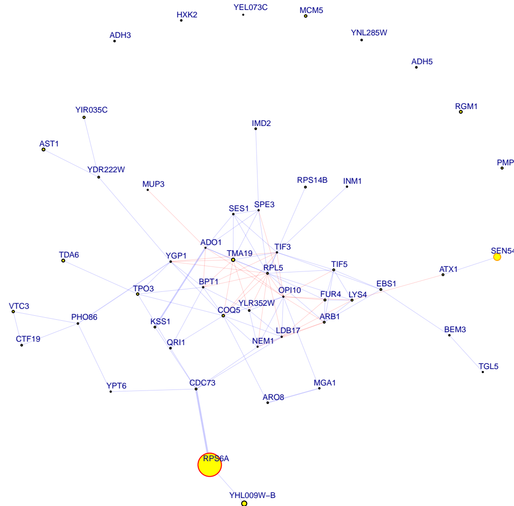
chrXVI:383928_G/A top 50 down genes
