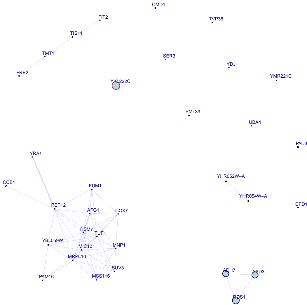
chrXI:4534_G/A top 34 up genes
