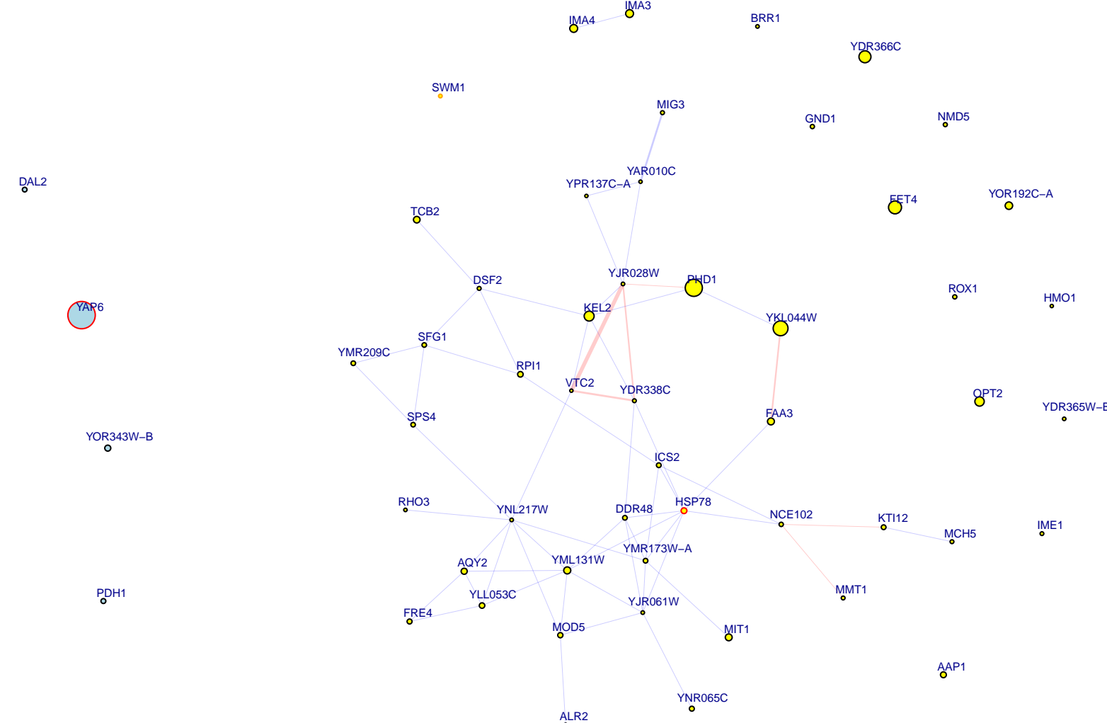
chrIV:975156_A/G top 50 down genes
