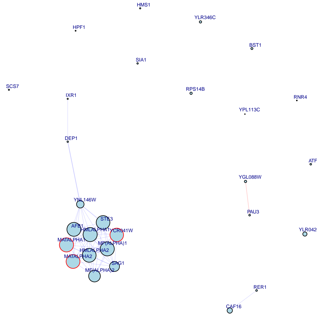
chrIII:201185_C/A top 28 up genes
