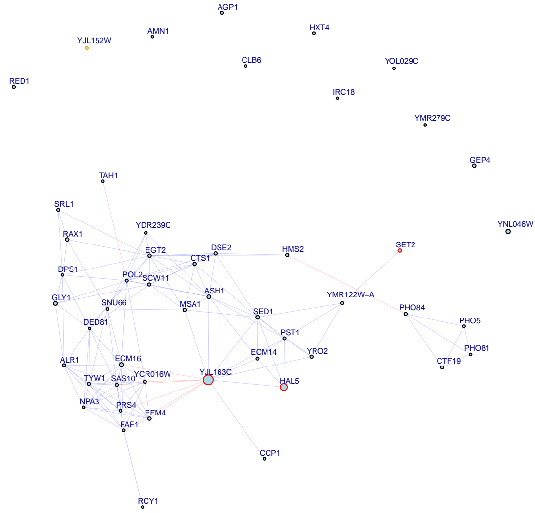
chrX:108904_A/G top 50 up genes
