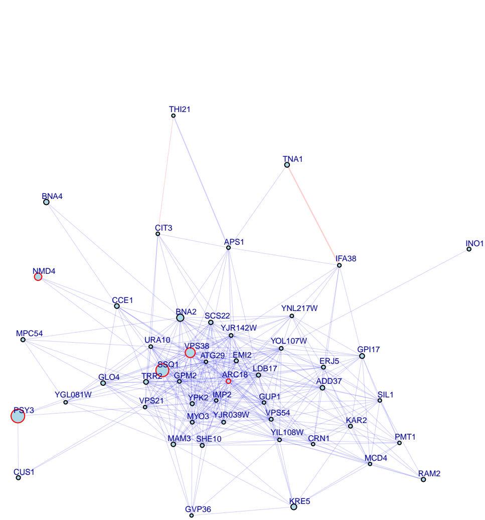
chrXII:848842_A/G top 50 up genes
