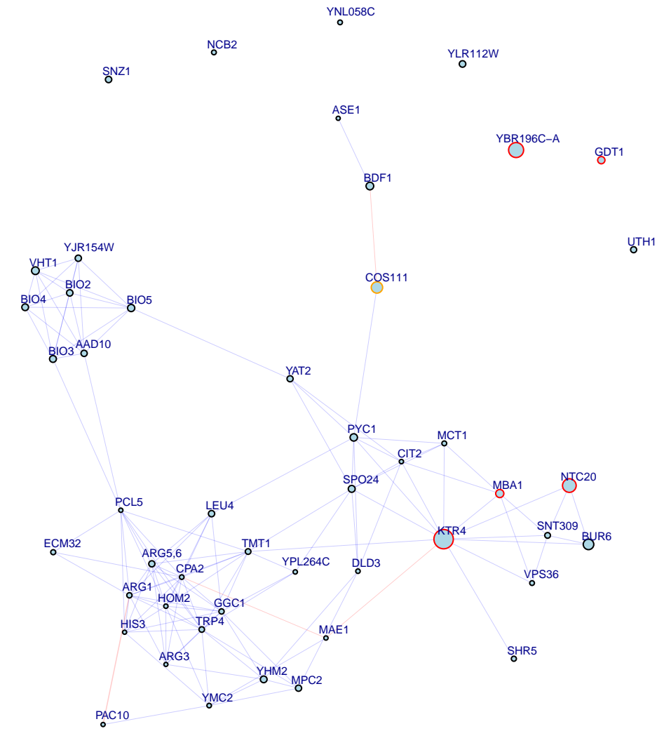
chrII:619028_C/A top 50 up genes
