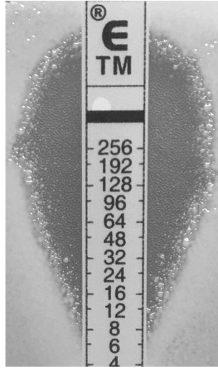
recA::Tc/precA
